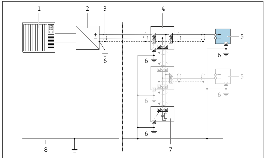
13 Пример подключения для PROFIBUS PA
