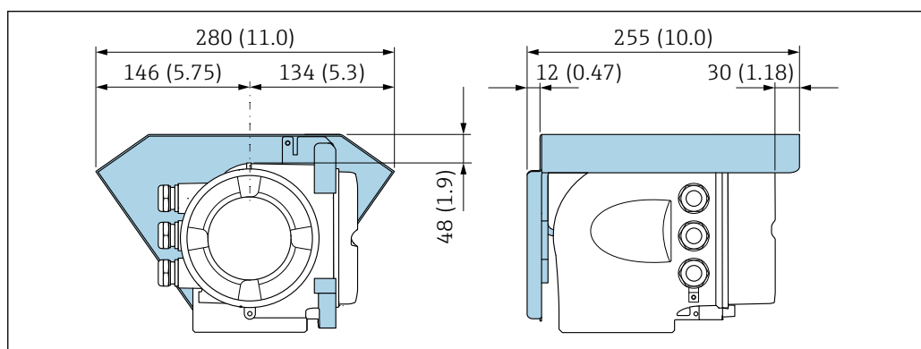
12 Защитный козырек от погодных явлений для прибора Proline 500; единицы измерения – мм (дюймы)
