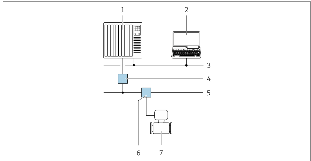
24 Варианты дистанционной работы через сеть PROFIBUS PA
