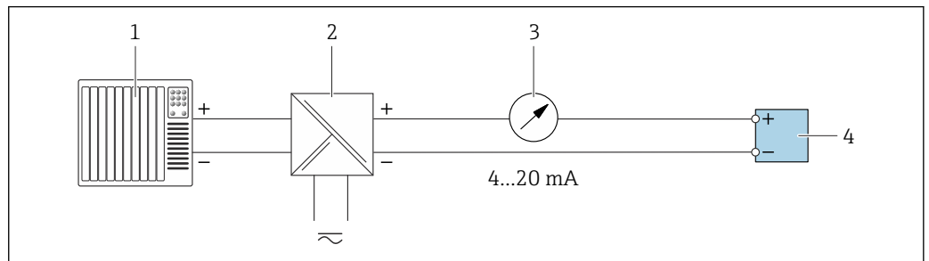
▣ 22 Пример подключения для токового выхода 4–20 мА (пассивного)
