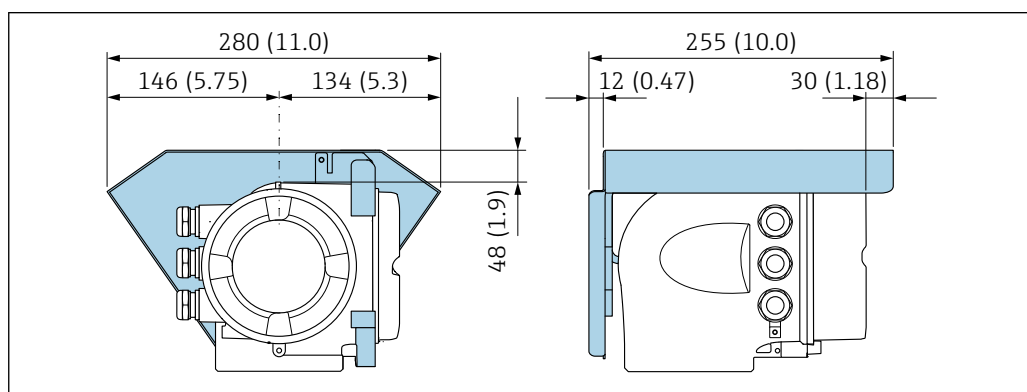
9 Защитный козырек от погодных явлений для прибора Proline 500; единицы измерения – мм (дюймы)
