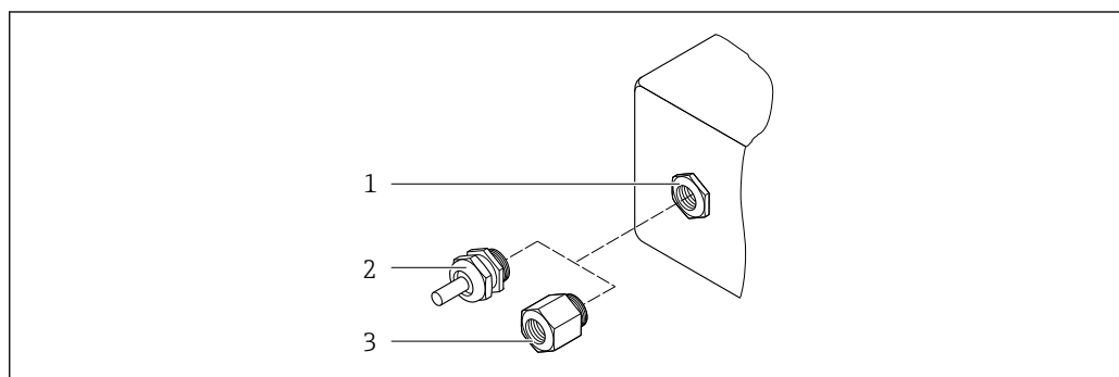
45 Возможные варианты кабельных вводов/кабельных уплотнений
