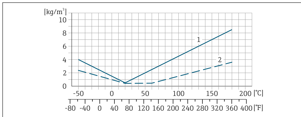
1 Калибровка по плотности на месте эксплуатации, в примере – при температуре +20 °C (+68 °F) 2 Расширенная калибровка плотности
