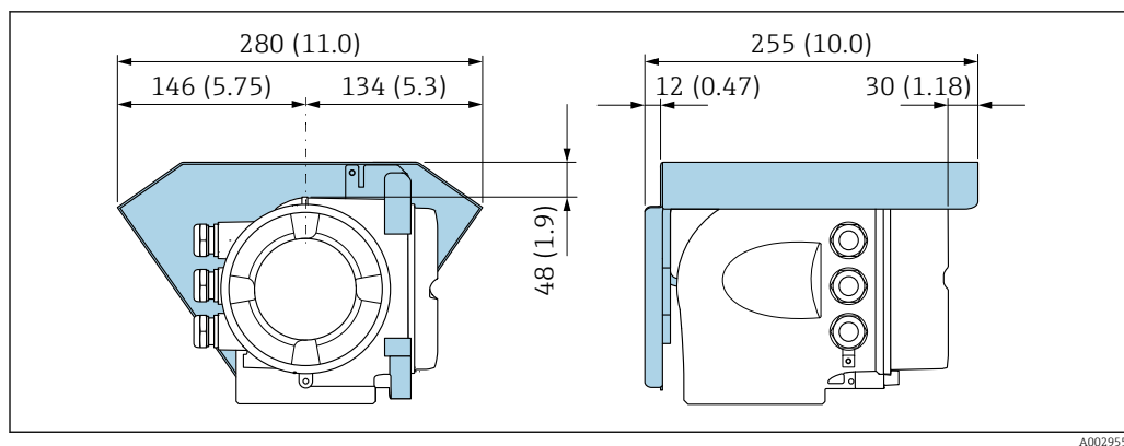
10 Защитный козырек от погодных явлений для прибора Proline 500; единицы измерения – мм (дюймы)
