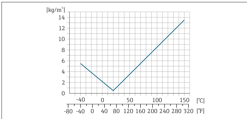
43 Калибровка по плотности на месте эксплуатации, в примере – при температуре +20 °C (+68 °F)
