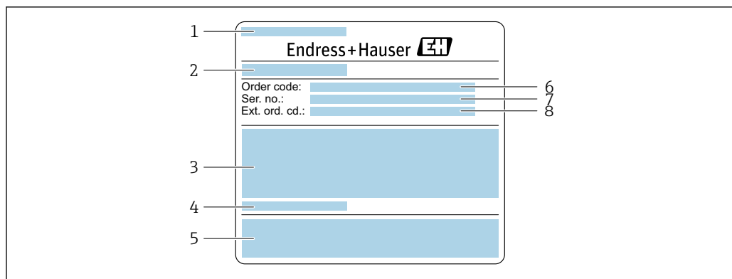
5 Пример заводской таблички датчика, часть 1
