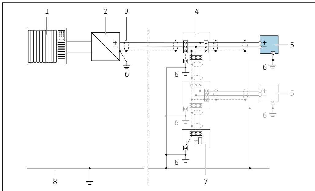
20 Пример подключения для PROFIBUS PA
