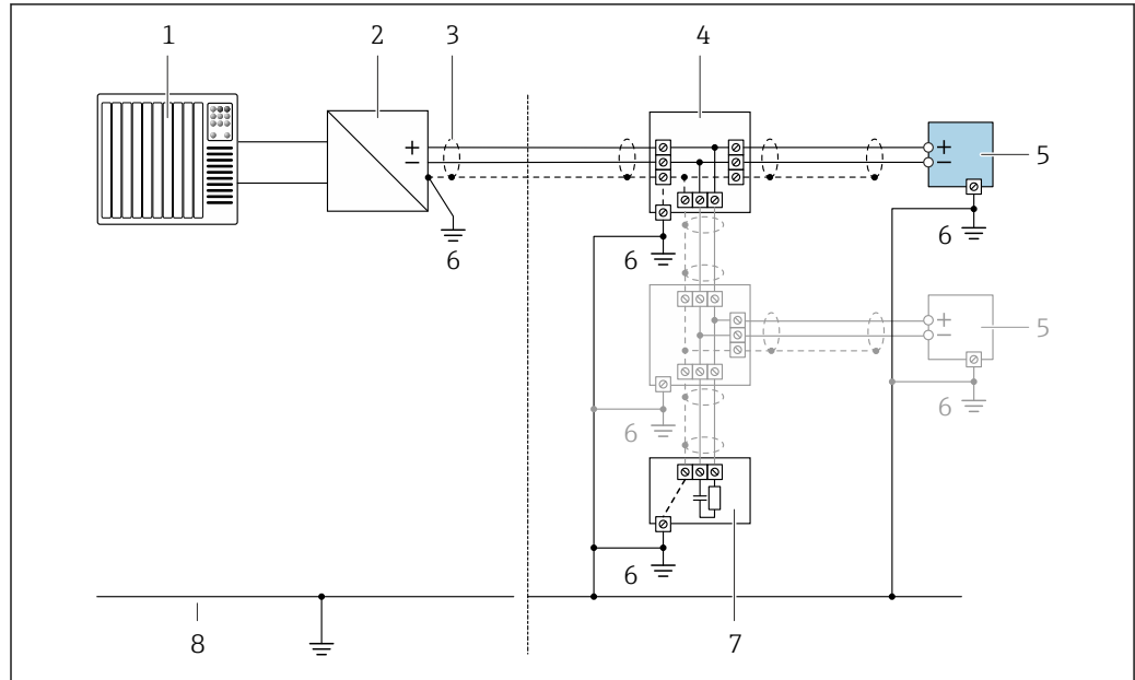
18 Пример подключения для PROFIBUS PA
