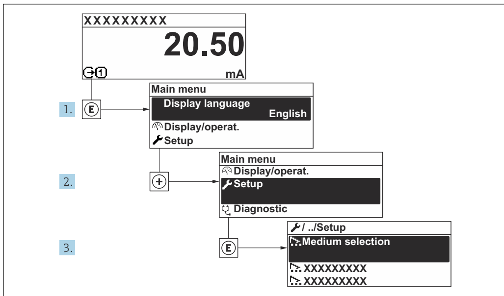
34 Навигация к меню "Настройка" на примере локального дисплея
