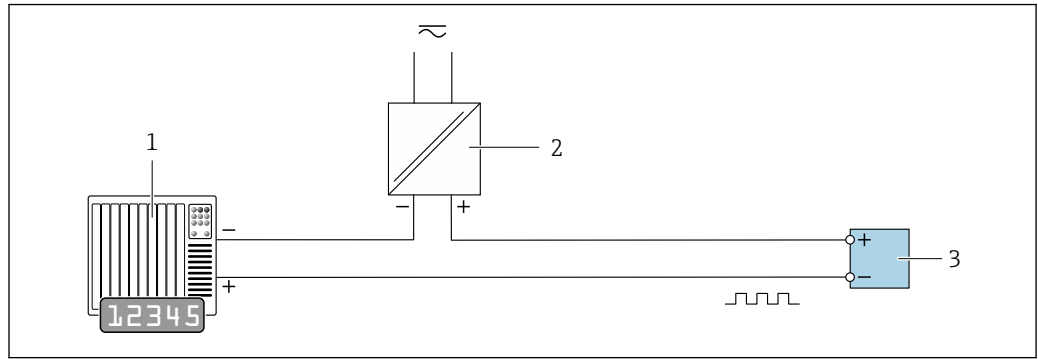
图 11 接线示例：脉冲/频率输出（无源信号）
