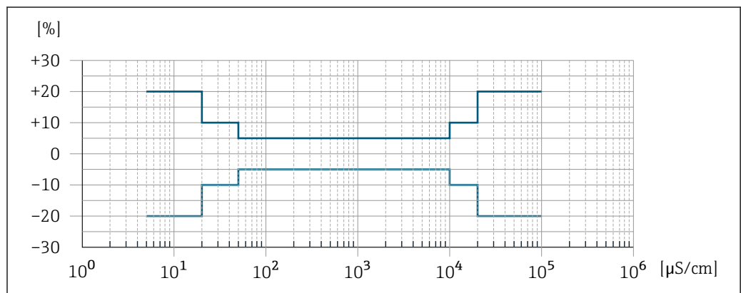
图 32 测量误差 (可选: 订购选项“电导率测量标定”，选型代号 CW)
