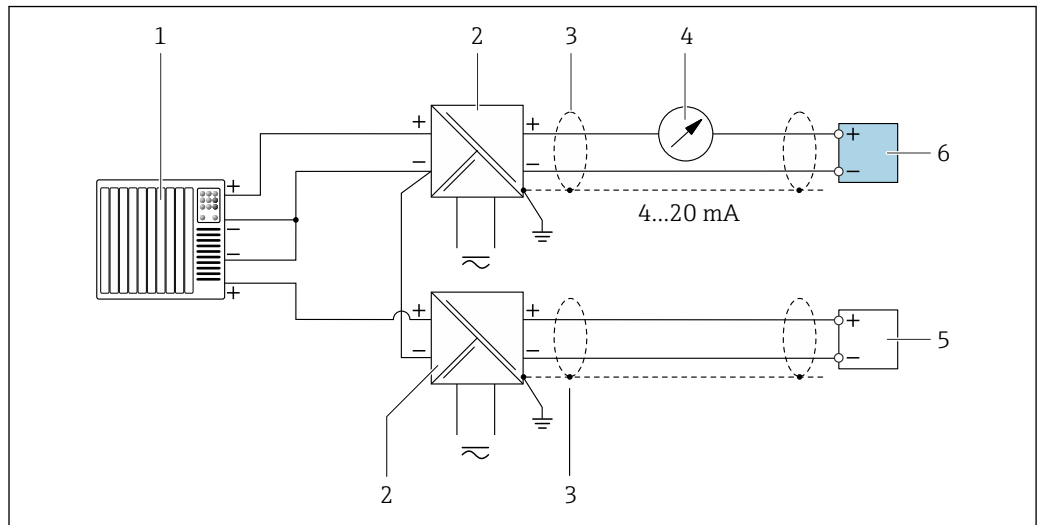
图 10 接线实例：HART 输入，公共端接负极（无源信号）
