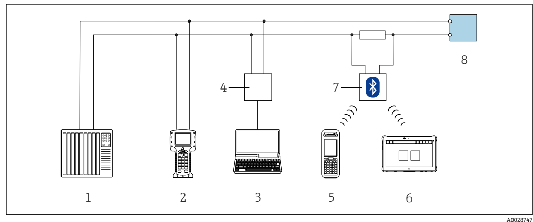
图 24 通过 HART 通信进行远程操作（有源信号）
