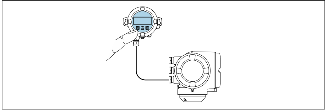
图 39 通过远传显示单元 DKX001 操作
