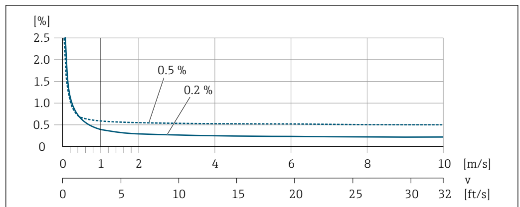
图 34 最大测量误差 (% o.r.)
