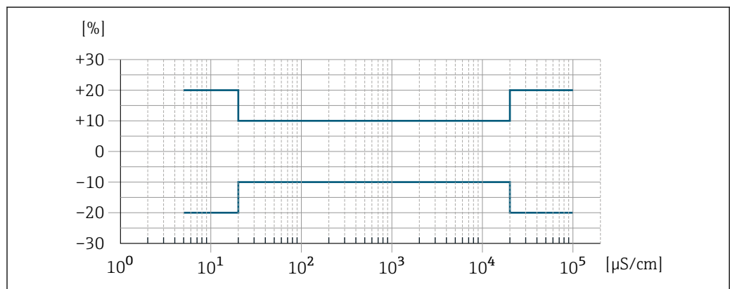
图 35 测量误差 (标准)
