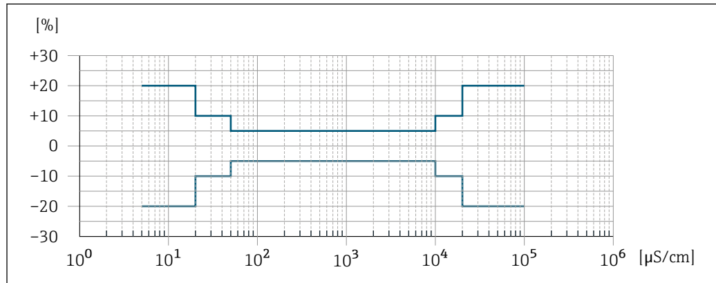
36 Écart de mesure (en option : caractéristique de commande "Mesure de conductivité étalonnée", option CW)
