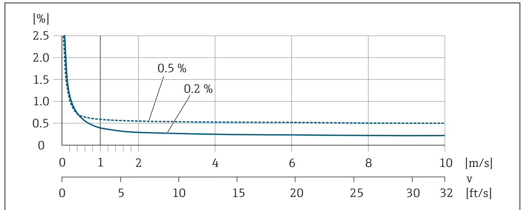
34 Écart de mesure max. en % de m.
