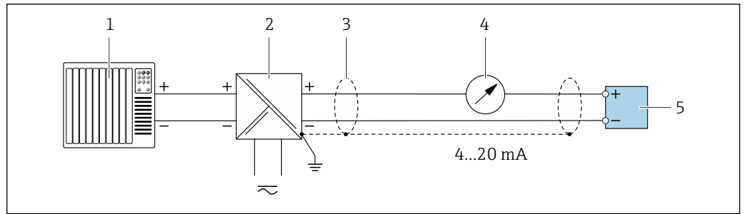
9 Exemple de raccordement pour sortie courant 4 à 20 mA HART (passive)
