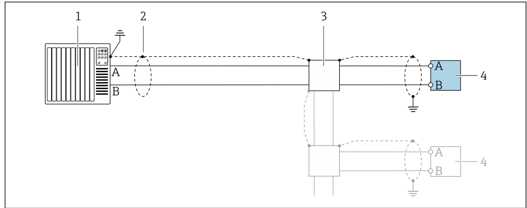
图 8 接线实例：PROFIBUS DP，非危险区和防爆 2 区/ Div. 2 防爆场合
