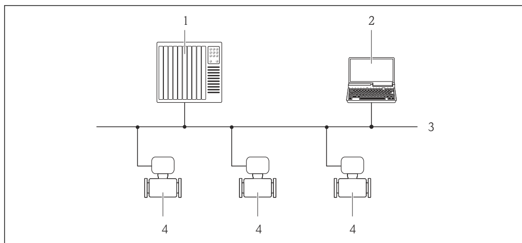
图 20 通过 PROFIBUS DP 网络进行远程操作
