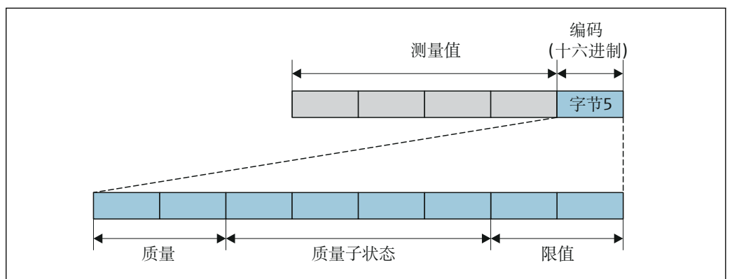
图 26 编码字节结构
