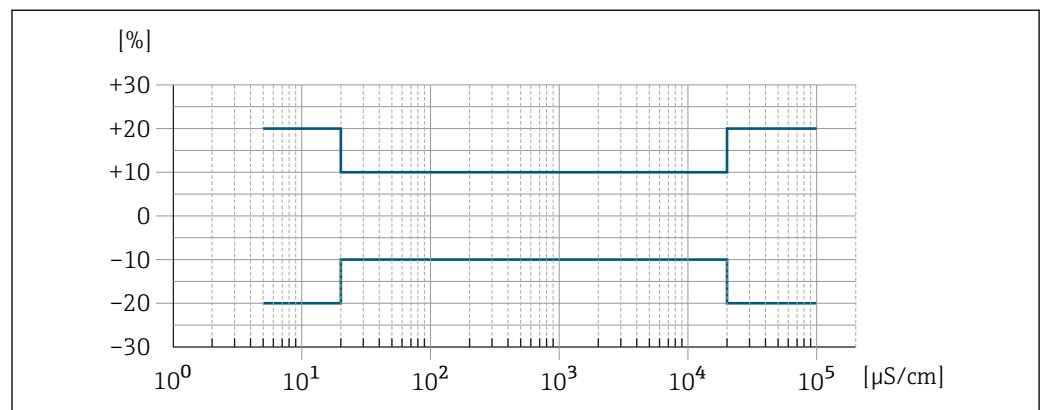
图 30 测量误差 (标准)
