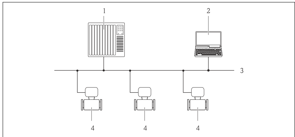
20 Opções para operação remota através da rede PROFIBUS DP
