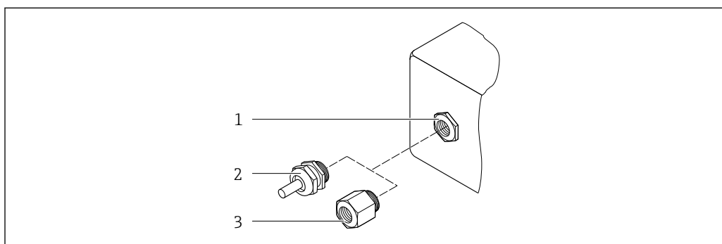
32 Possíveis entradas para cabo/prensa-cabos
