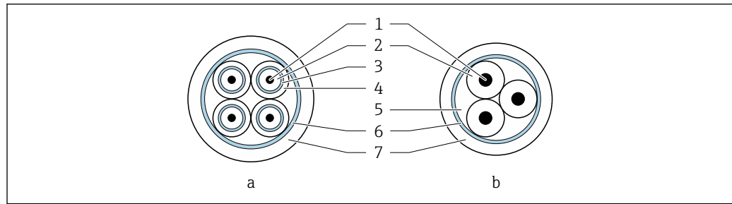
图 23 电缆截面图
