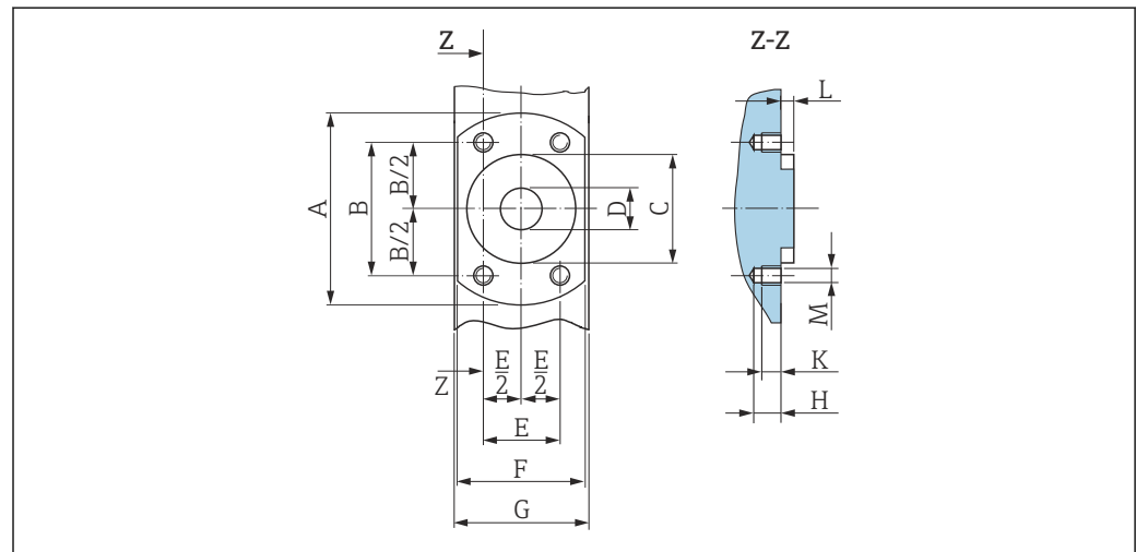
图 62 正视图，无过程连接
