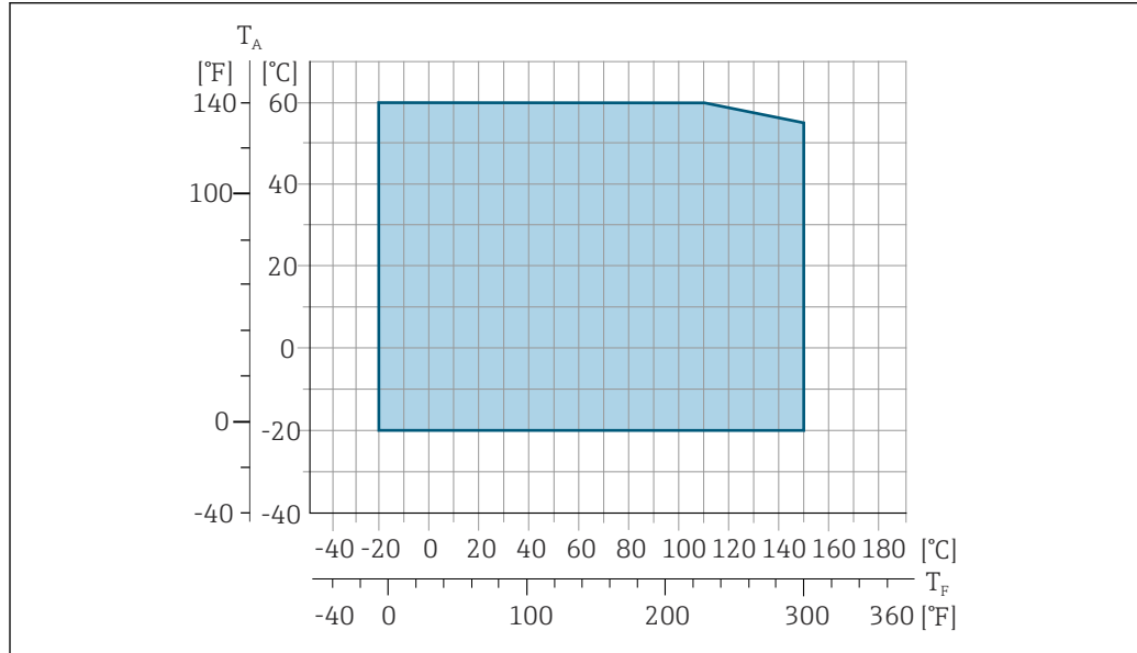
图 35 Promag 500 (模拟)
