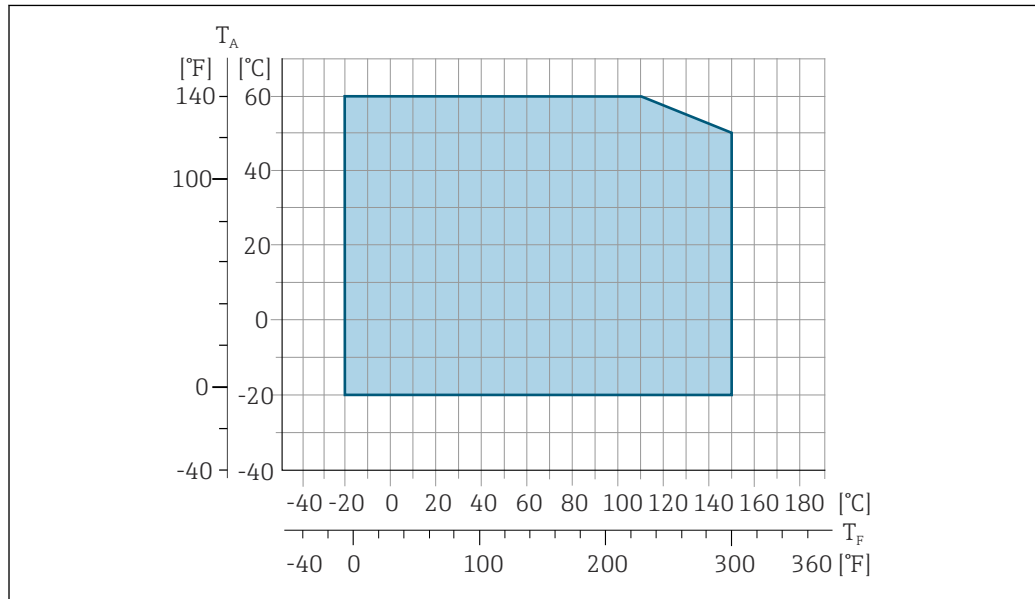
图 34 Promag 500 (数字)
