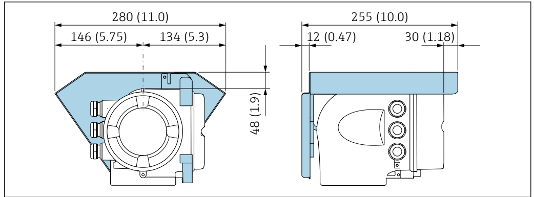
图 65 Proline 500 变送器的防护罩的外形尺寸图；单位：mm (in)
