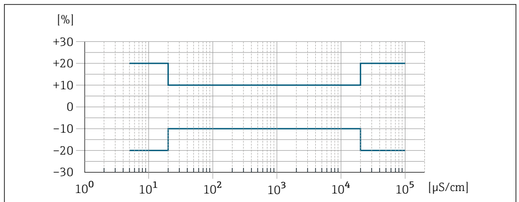
图 25 测量误差 (标准)
