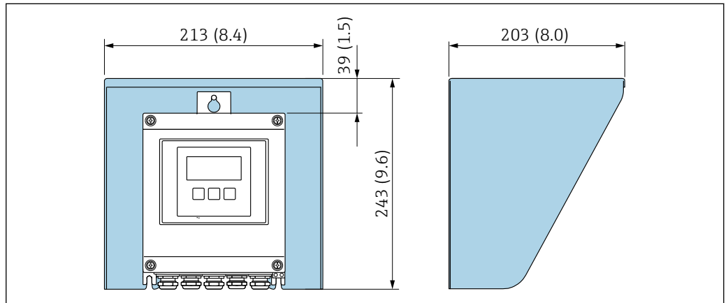
图 56 Proline 500 (数字) 变送器的防护罩的外形尺寸图; 单位: mm (in)
