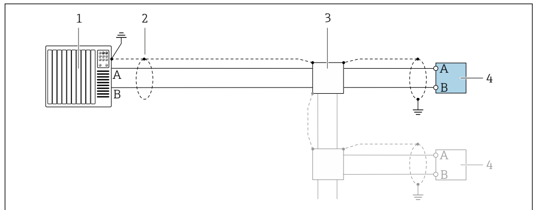
图 17 接线实例：PROFIBUS DP，非危险区和防爆 2 区 / Div. 2 防爆场合
