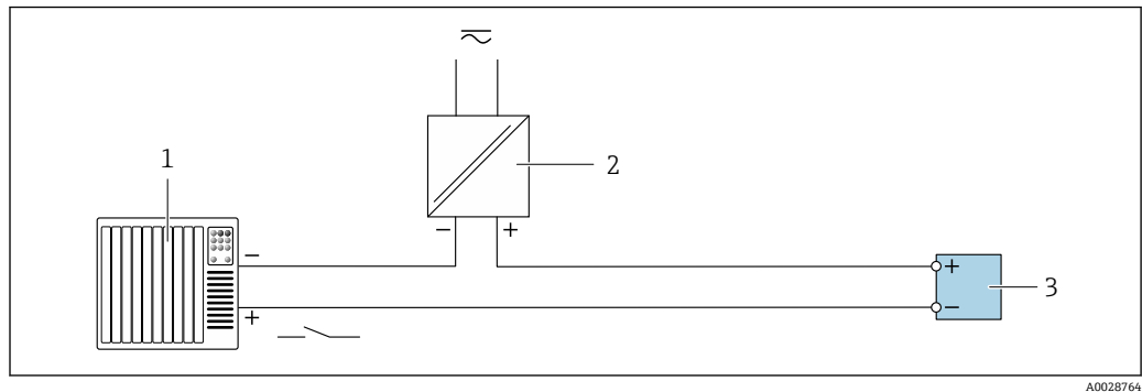
图 24 接线实例：状态输入
