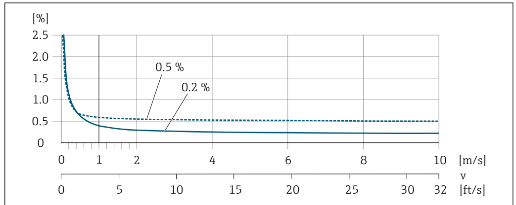
图 39 最大测量误差 (% o.r.)
