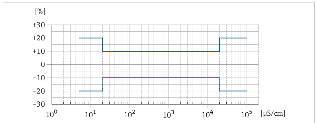
图 40 测量误差 (标准)
