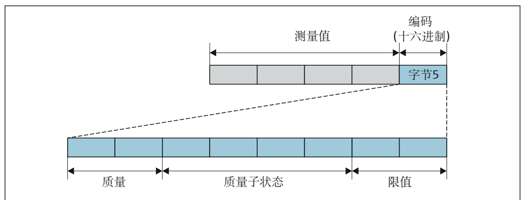
图 36 编码字节结构
