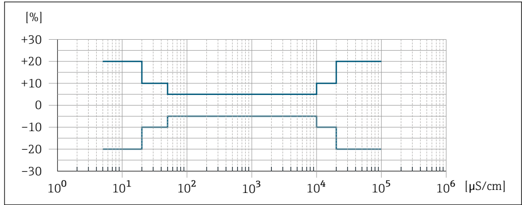
图 41 测量误差 (可选: 订购选项“电导率测量标定”, 选型代号 CW)
