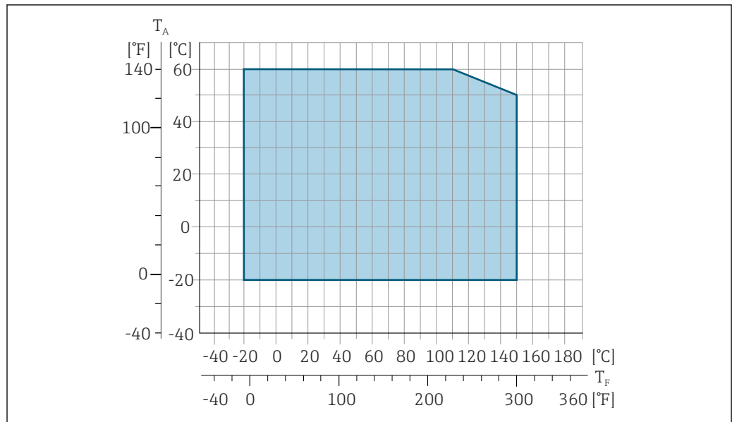
图 44 Promag 500 (数字)
