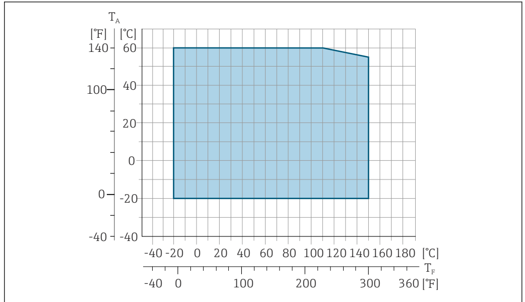
图 45 Promag 500 (模拟)
