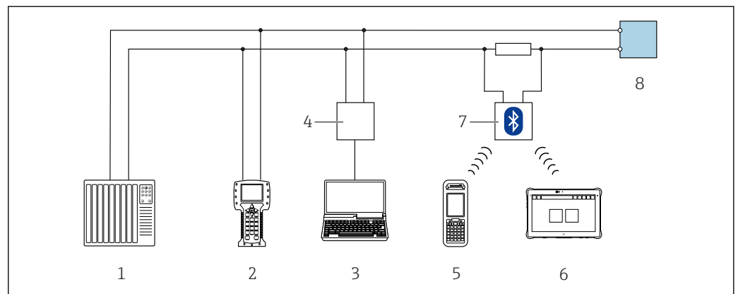
图 20 通过 HART 通信实现远程操作
