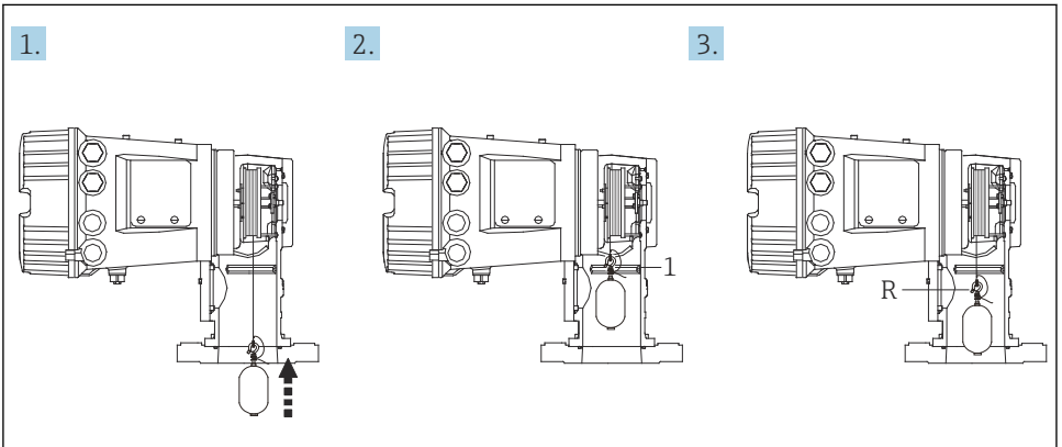
28 Sekvensen vid referenskalibrering
