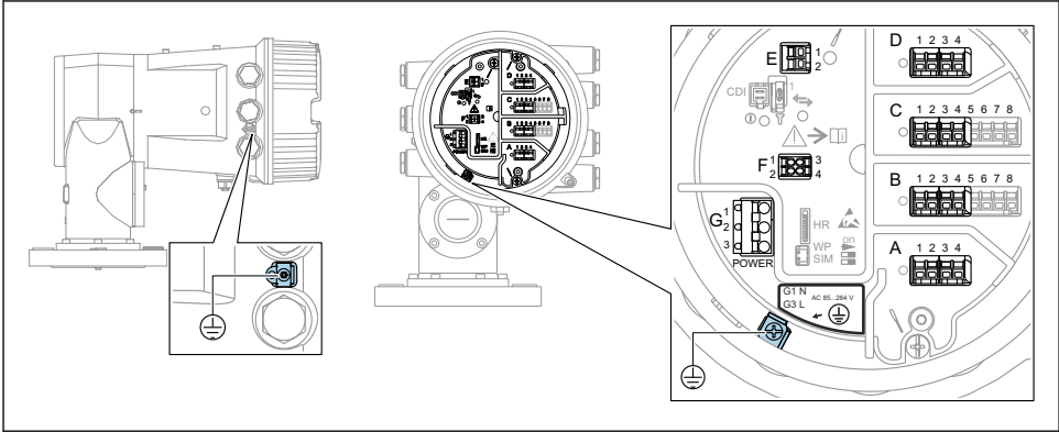
9 Plintenhet (typexempel) och jordningsplintar
