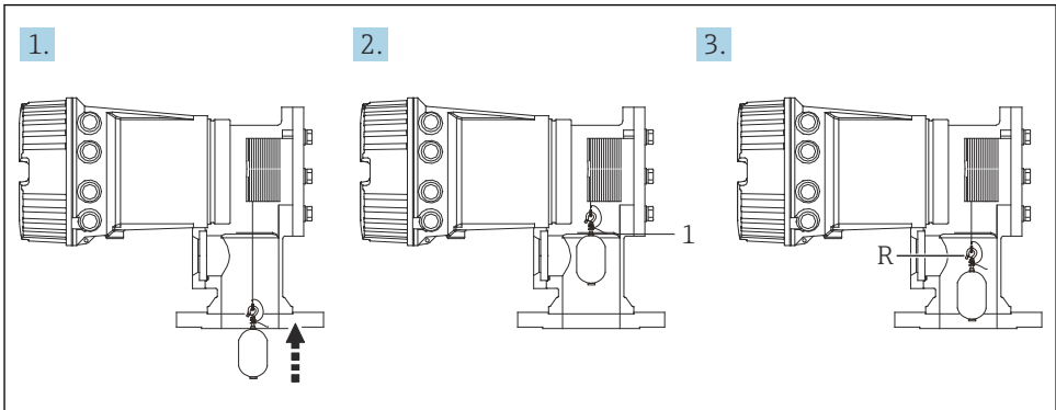
☐ 28 기준 교정 순서
