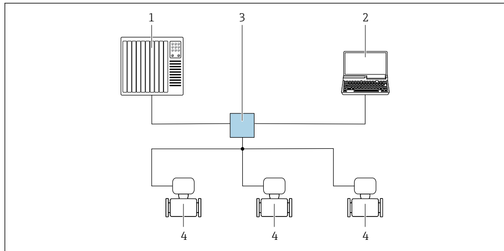
18 Möglichkeiten der Fernbedienung via PROFINET Netzwerk: Sterntopologie
