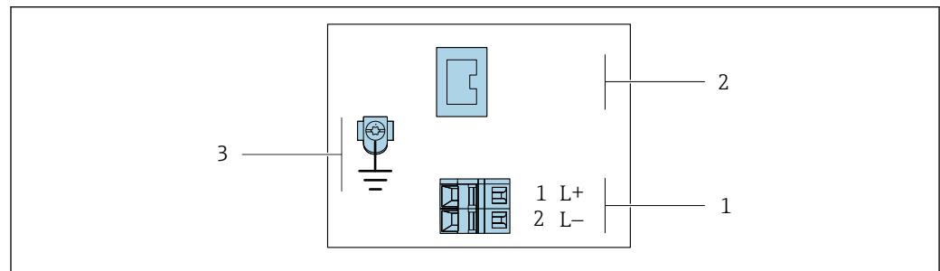
8 Klemmenbelegung EtherNet/IP
