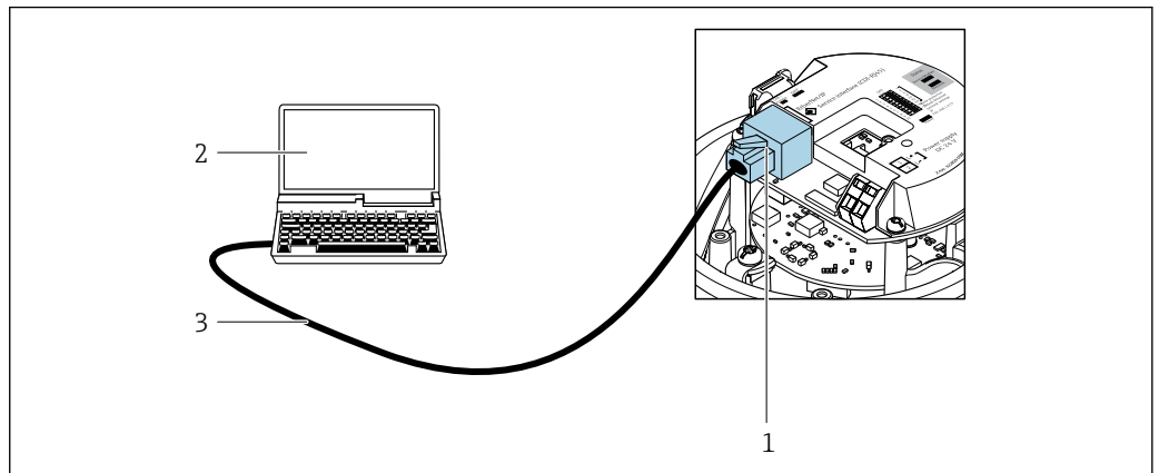
18 Anschluss bei Bestellmerkmal "Ausgang", Option N: EtherNet/IP
