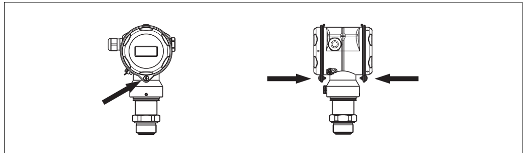
图 4: 关闭外壳盖
