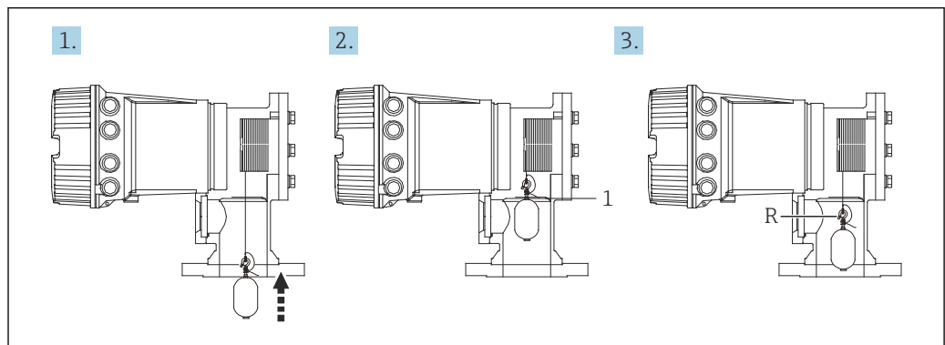
图 46 参考标定步骤
