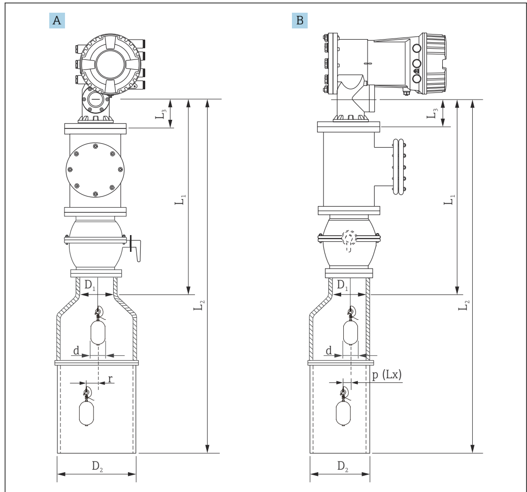
图 7 非对中心导波管的安装示意图
