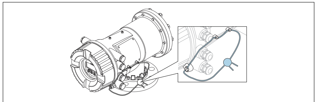
36 密封接线腔盖板
