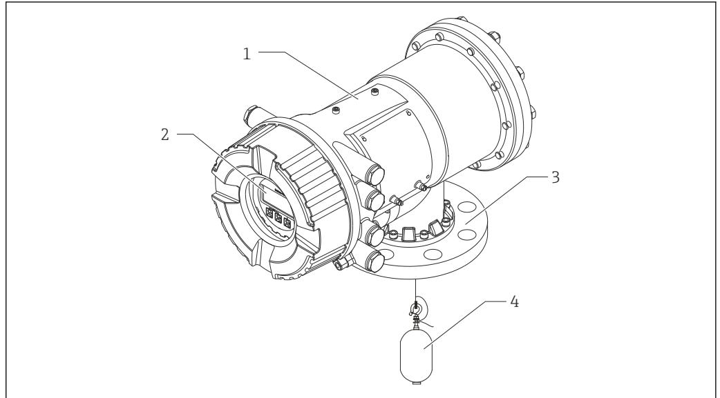
图 1 Proservo NMS81 的结构示意图
