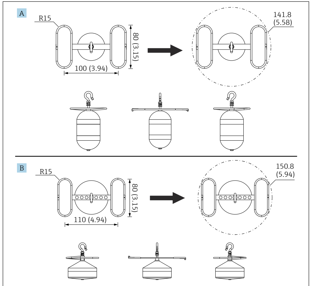
图 10 导向环
