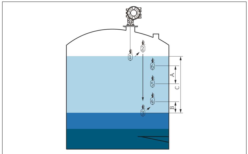
图 58 界面梯度位移（数字显示浮子的移动顺序）示意图
