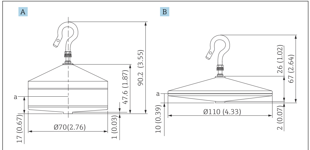
A \varnothing 70 mm (2.76 in)直径的 316L 圆锥形浮子 B \varnothing 110 mm (4.33 in)直径的 316L 圆锥形浮子 a 浸没点
