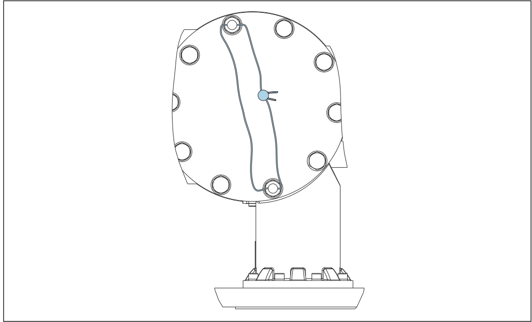
图 37 密封后盖 (例如 NMS81/NMS83)
