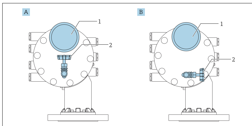
图 83 减压阀和压力表的安装位置
