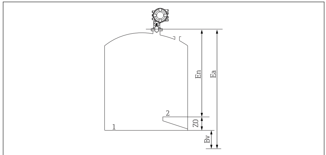
图 52 敞开式无液体储罐
