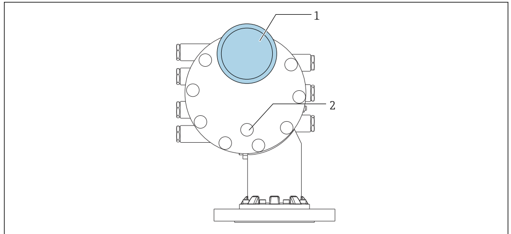
图 88 压力表和气体吹扫短管
