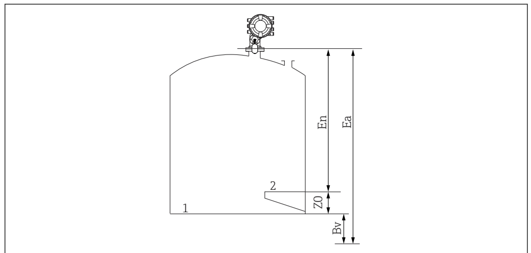
图 45 敞开式无液体储罐
