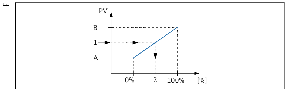
图 67 按百分比调整罐体参数
