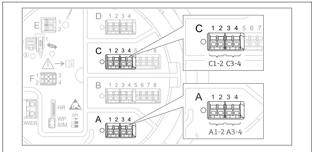
图 60 数字量输入/输出模块的可能安装位置 (示例) ; 订货号确定数字量输入模块的数量和位置 → 37。
