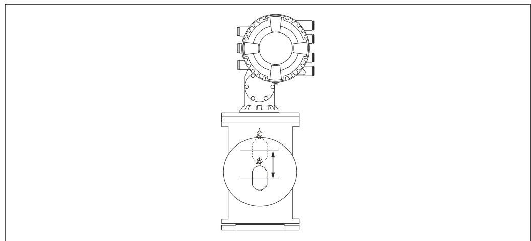
图 37 移动浮子
