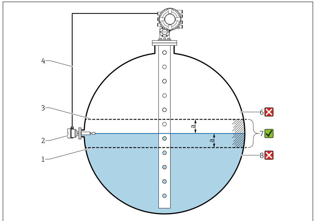
图 63 带液位开关的应用实例
