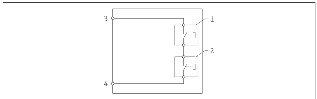
88 数字量输出的两个继电器
