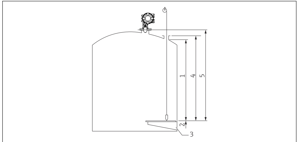
图 43 罐体高度
