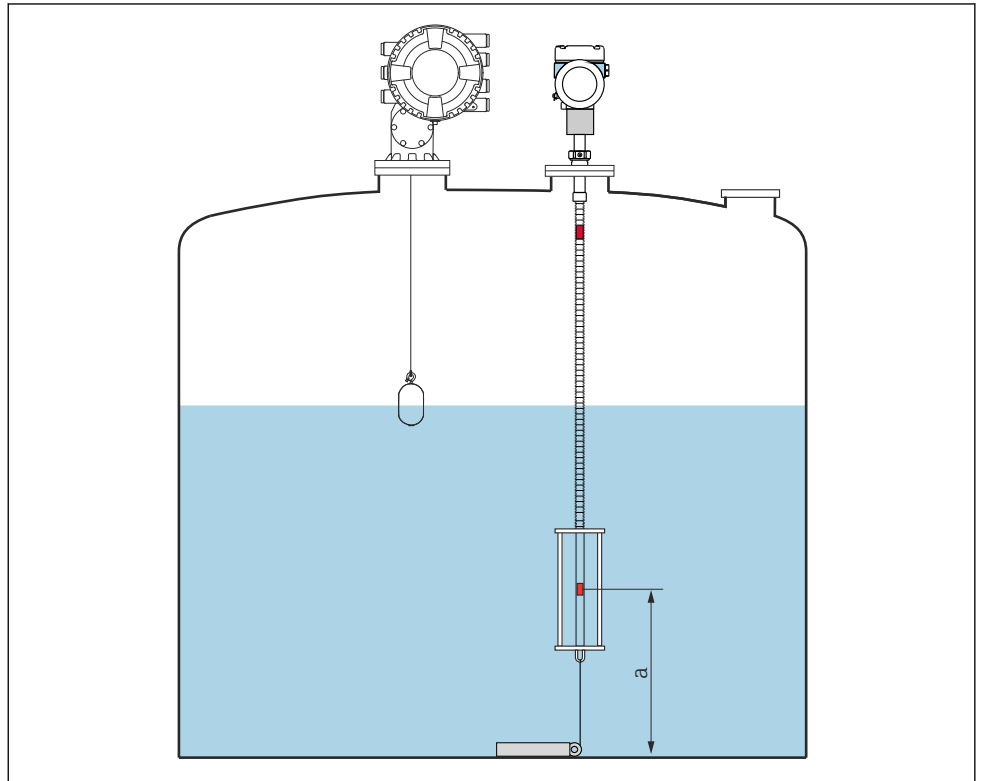
图 54 Prothermo NMT53x: 罐底测温元件位置
