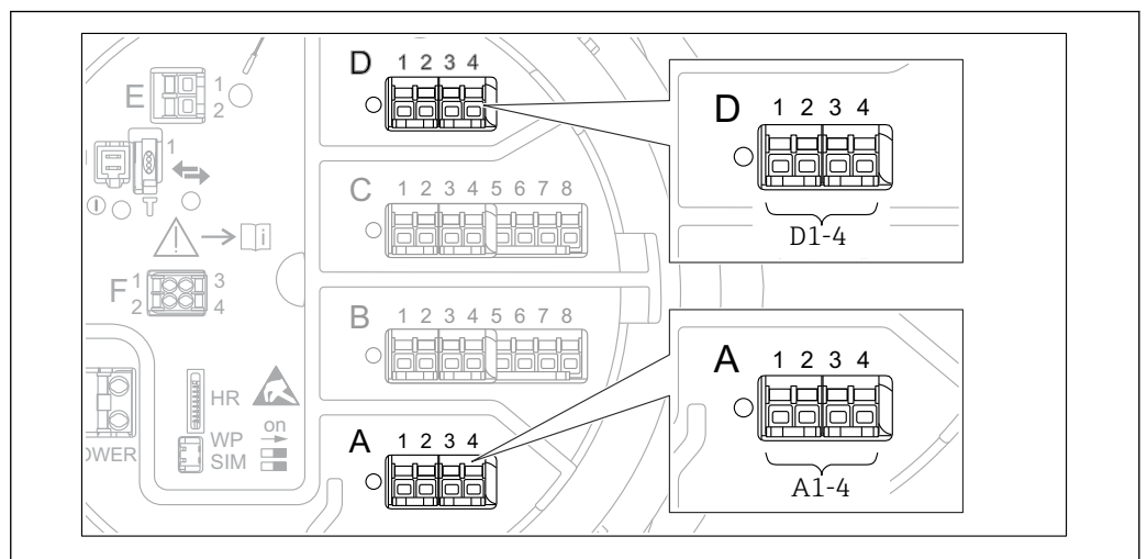
图 70 WM550 模块的可能安装位置 (实例)；取决于设备型号，上述模块还可以安装在插槽 B 或 C 中 → 图 37。
