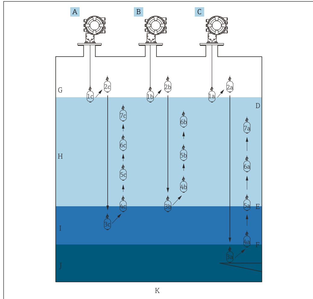
图 49 密度梯度示意图 (1a、2a、3a...显示浮子移动顺序)
