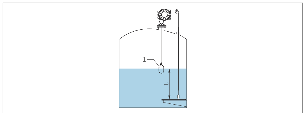
图 44 设置敞开式液体储罐液位示意图
