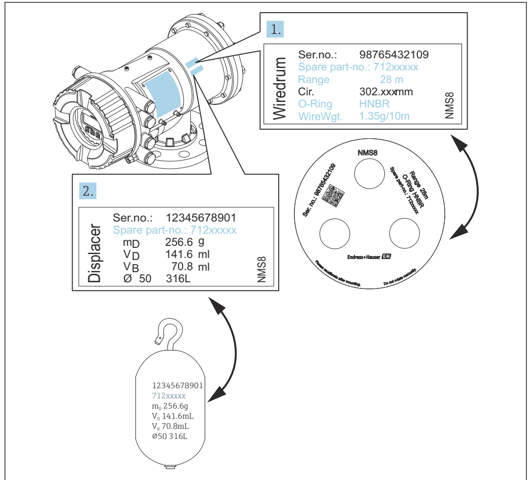
11 验证浮子和轮鼓
