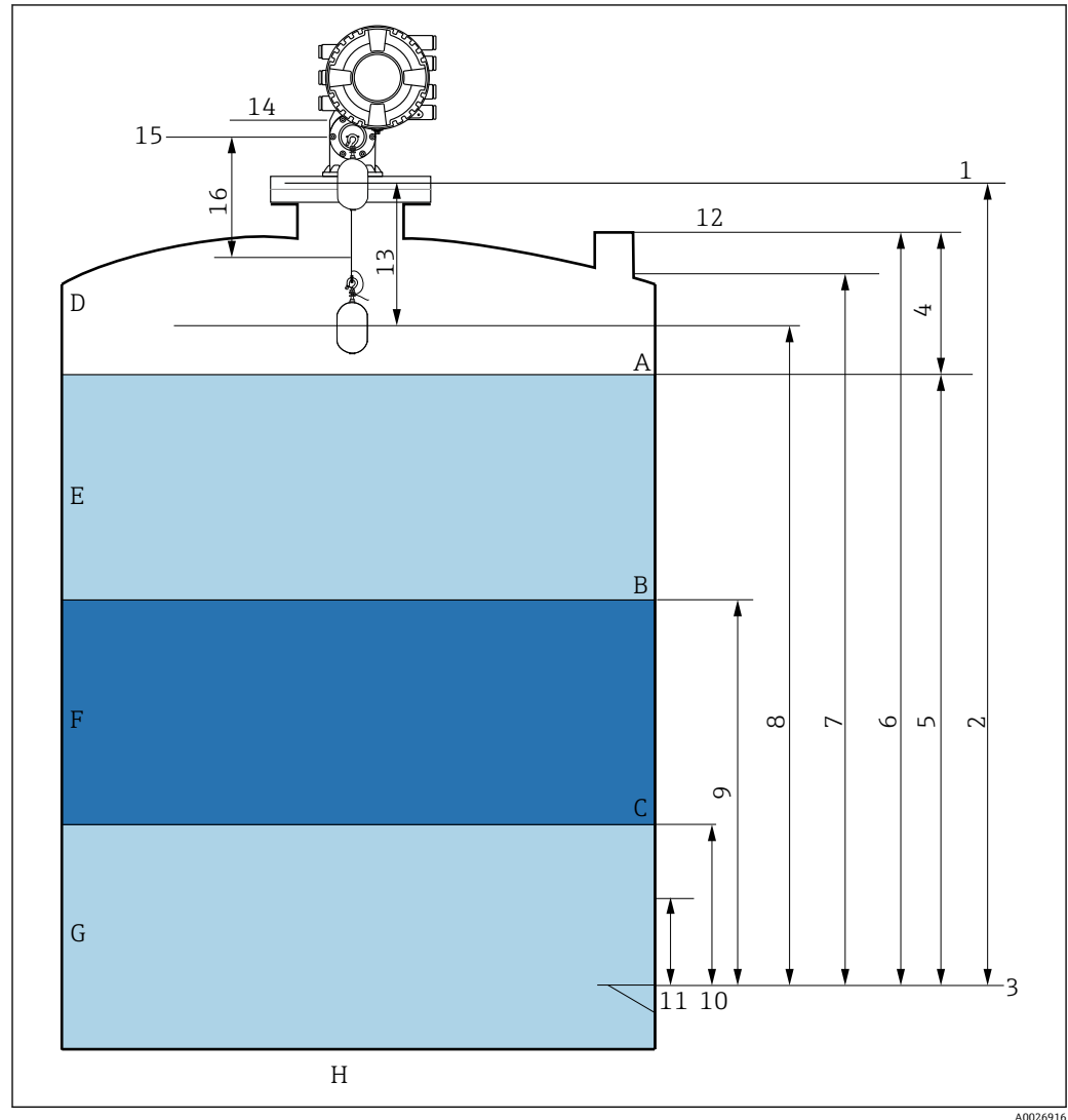
图 35 NMS8x 安装术语 (例如 NMS81)
