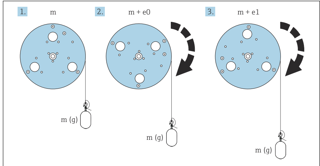
图 40 测量重量
