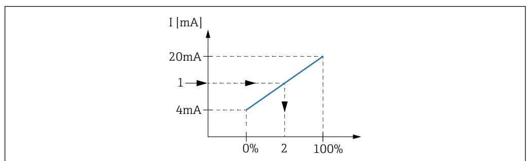
图 57 4...20 mA 输入对应过程变量
