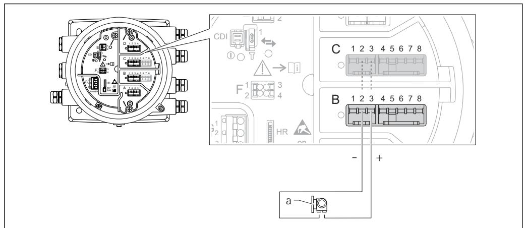
图 20 输入模式下的有源模拟量输入/输出模块
