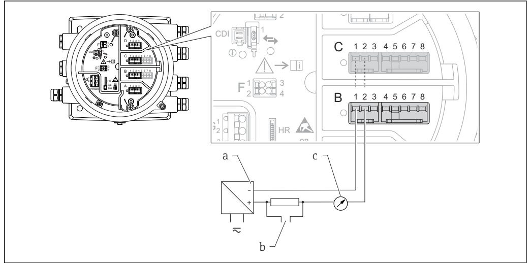
图 16 输出模式下的无源模拟量输入/输出模块
