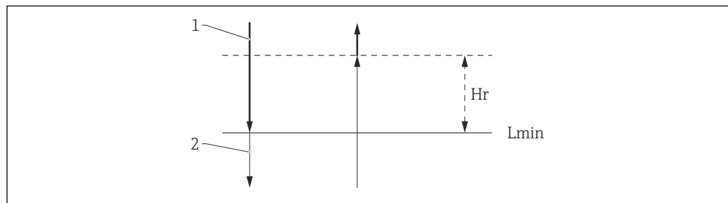
图 94 HTMS 单点回差控制范围
