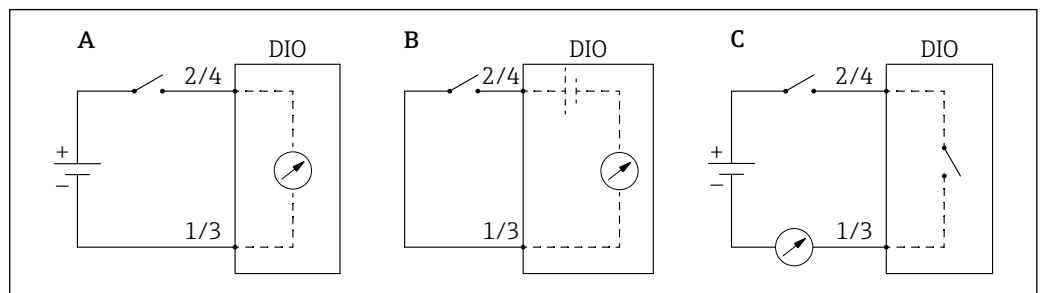
87 数字量输入/输出模块的工作模式
