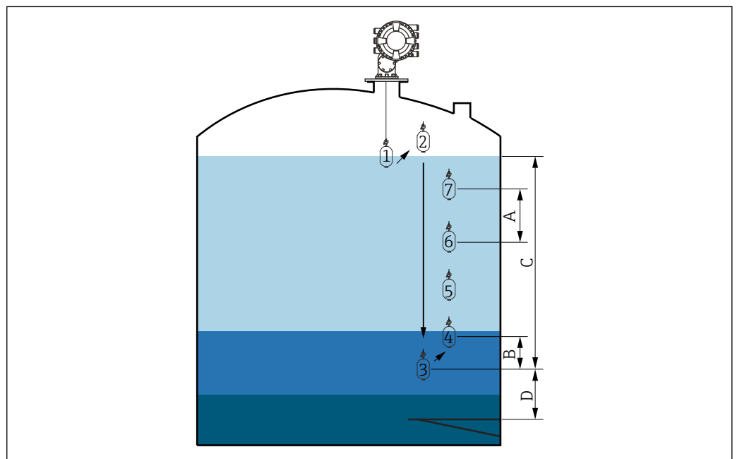
图 52 手动梯度位移 (数字显示浮子的移动顺序) 示意图
