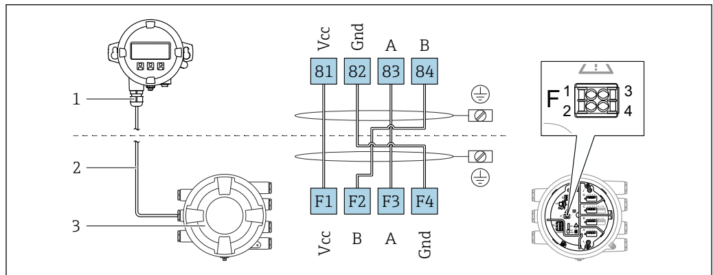
图 14 分离型显示单元与操作单元 DKX001 连接至伺服罐表设备 (NMR8x、NMS8x 或 NRF8x)
