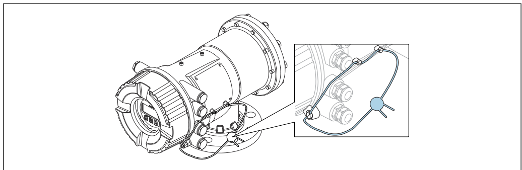
29 密封接线腔盖板
