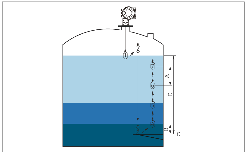
图 50 罐体梯度位移（数字显示浮子的移动顺序）示意图
