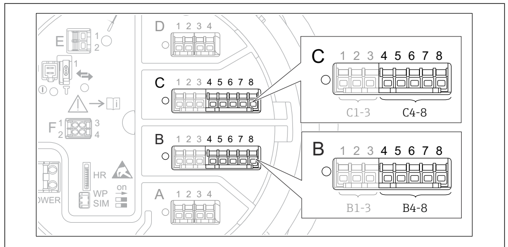
图 84 “Analog IP” 子菜单的接线端子（分别为“B4-8”或“C4-8”）
