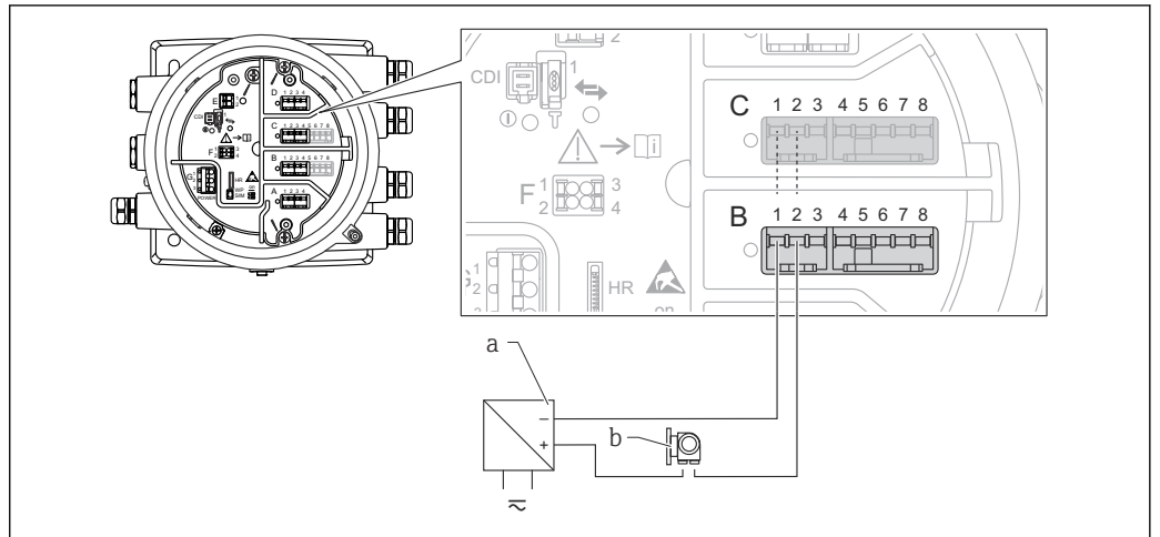
图 17 输入模式下的无源模拟量输入/输出模块
