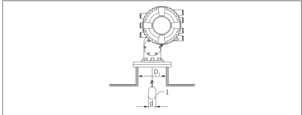
图 5 无导向系统的安装示意图
