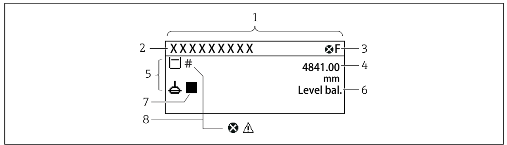
图 24 典型的标准显示界面 (测量值显示)
