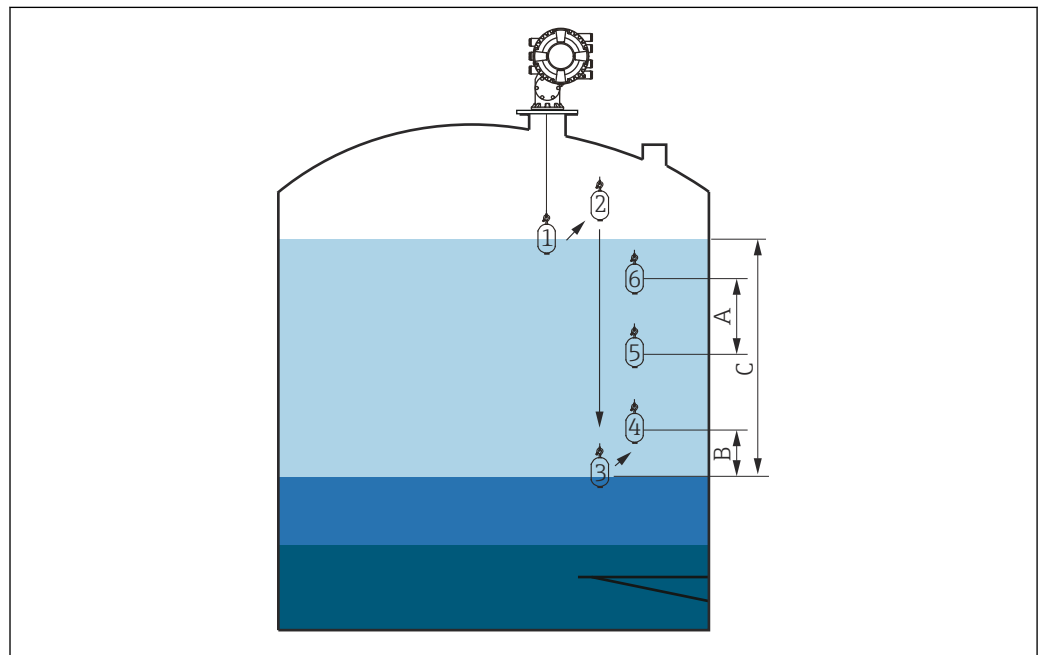
图 51 界面梯度位移（数字显示浮子的移动顺序）示意图
