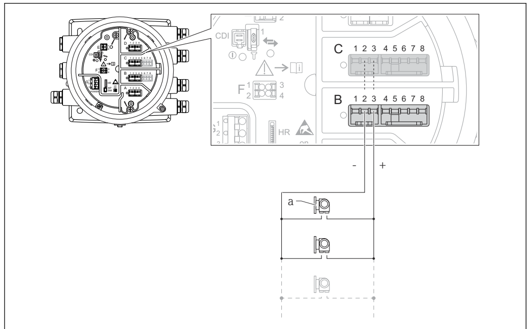
图 21 HART 主站模式下的有源模拟量输入/输出模块
