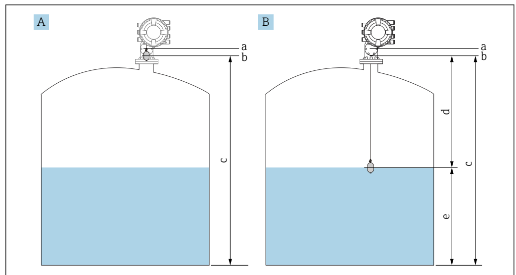
图 47 空罐液位设置示意图 (NMS83)
