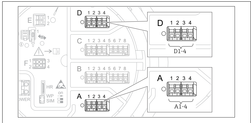
图 89 “Modbus”、“V1”或“WM550”模块名称实例；取决于设备型号，上述模块可以安装在插槽 B 或插槽 C 中。
