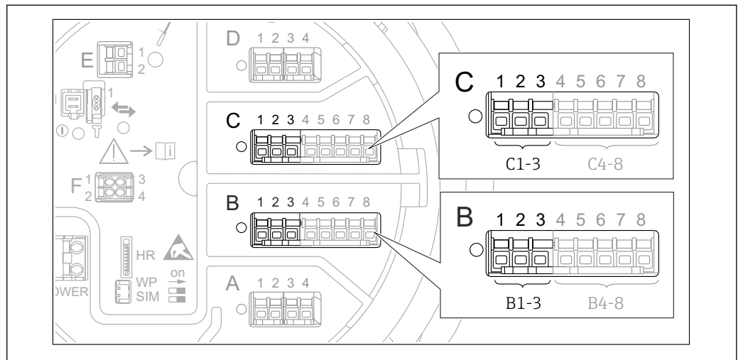
85 “Analog I/O” 子菜单的接线端子（分别为“B1-3”或“C1-3”）
