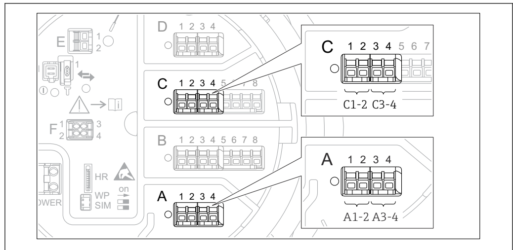
图 71 数字量输入/输出模块的可能安装位置 (实例)；订货号定义数字量输入/输出模块的数量和位置 → 图 37。
