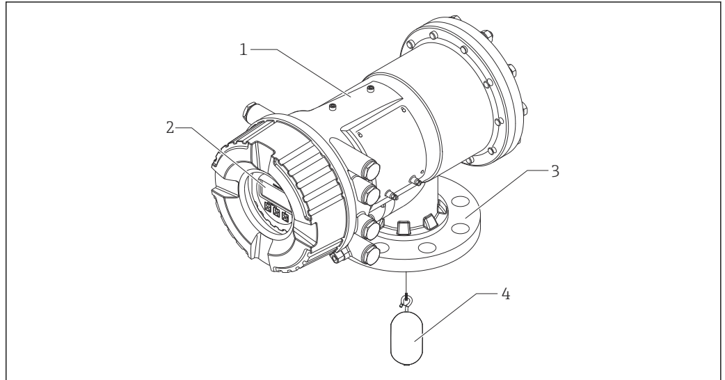
图 1 Proservo NMS83 的结构示意图
