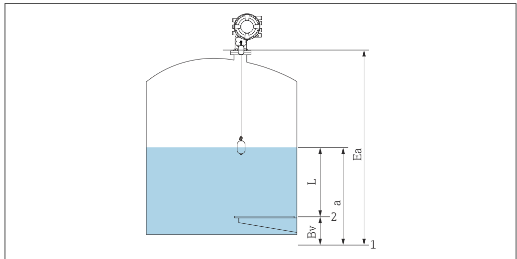
图 46 NMS83 封闭储罐示意图
