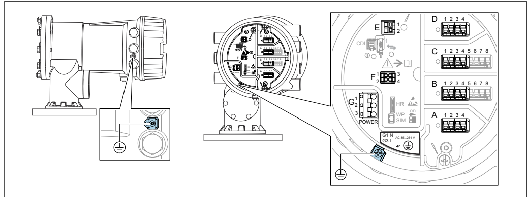
图 12 端子接线腔（典型实例）和接地端子示意图
