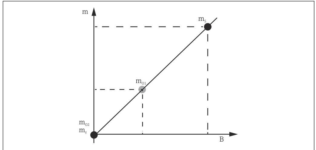
图 38 传感器标定原理
