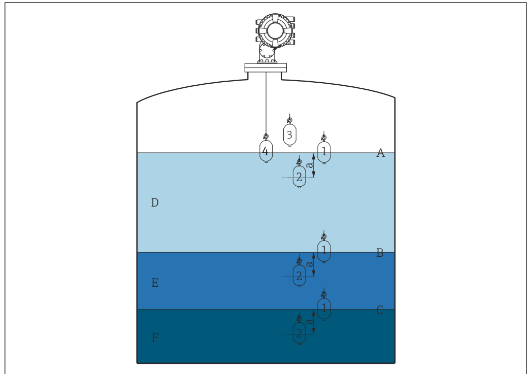
图 48 单点密度（数字显示浮子的移动顺序）示意图
