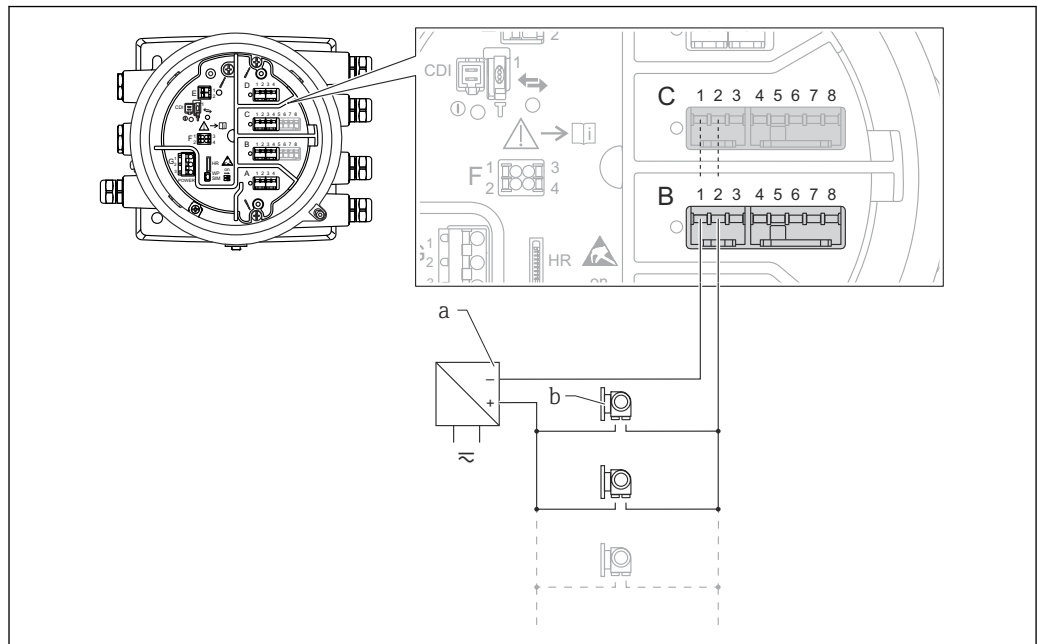
图 18 HART 主站模式下的无源模拟量输入/输出模块
