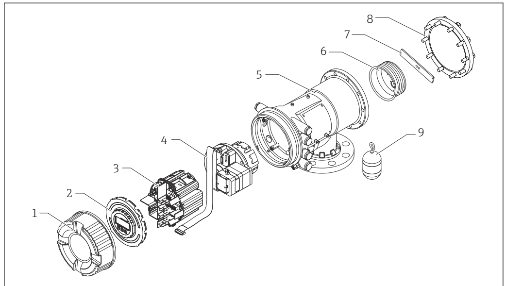
图 2 NMS83 的部件分解图
