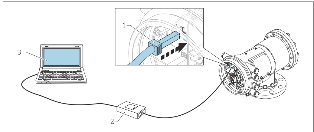
图 33 通过服务接口操作
