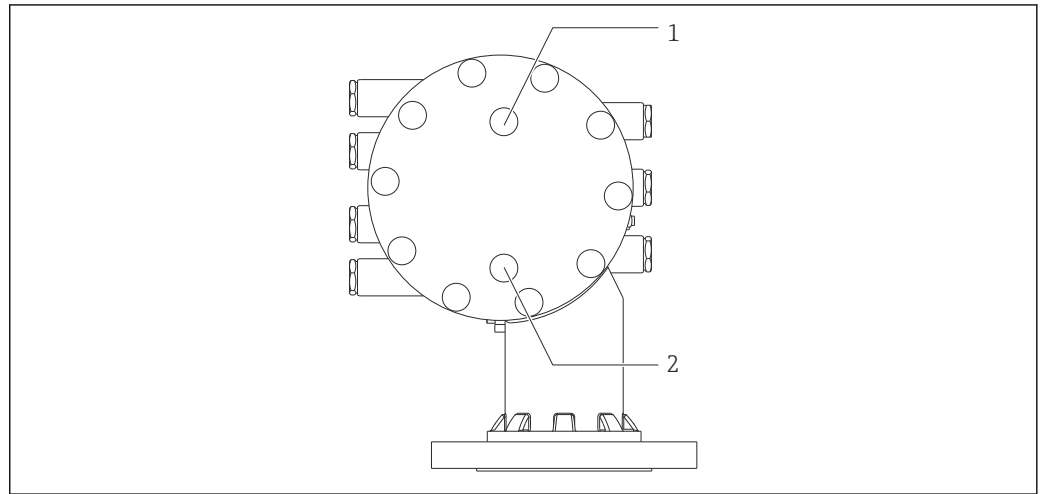
图 79 清洗短管和气体吹扫短管的连接孔口
