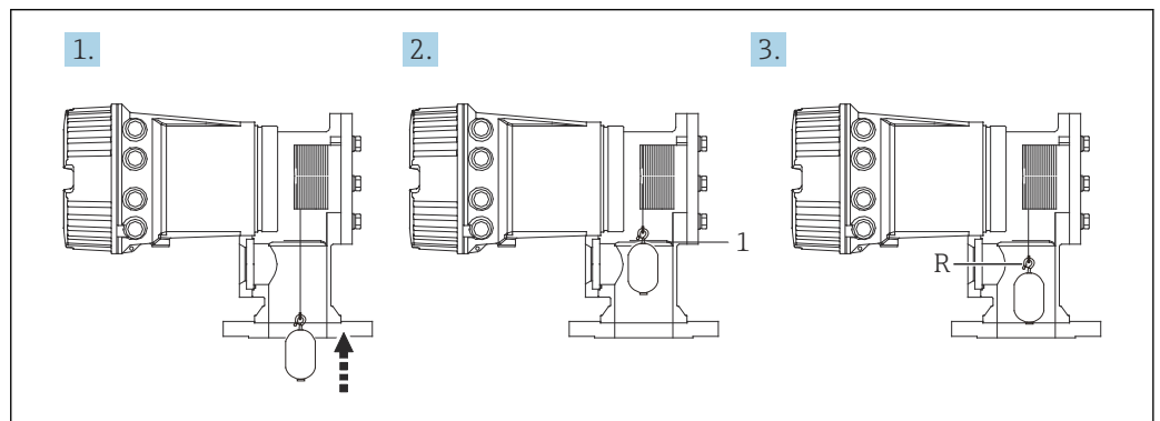
图 39 参考标定步骤
