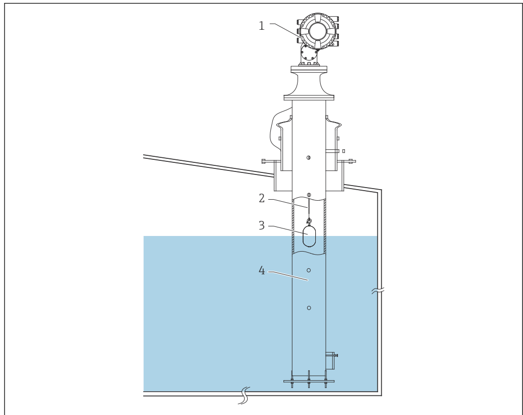
图 4 典型罐体安装方式 1 示意图
