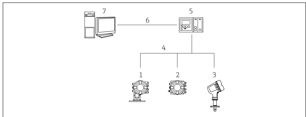
图 34 通过 Tankvision 储罐扫描仪 NXA820 连接伺服罐表设备至 FieldCare
