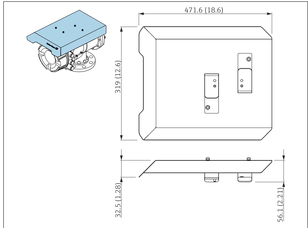
图 75 防护罩的外形尺寸示意图；单位：mm (in)
