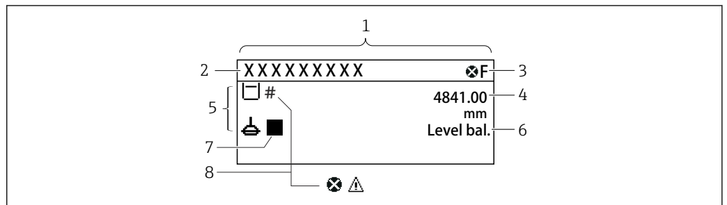
图 73 典型的标准显示界面（测量值显示）
