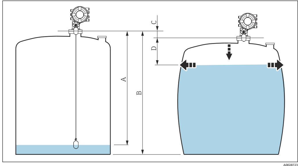
图 61 静压式储罐变形校正值 (HyTD)
