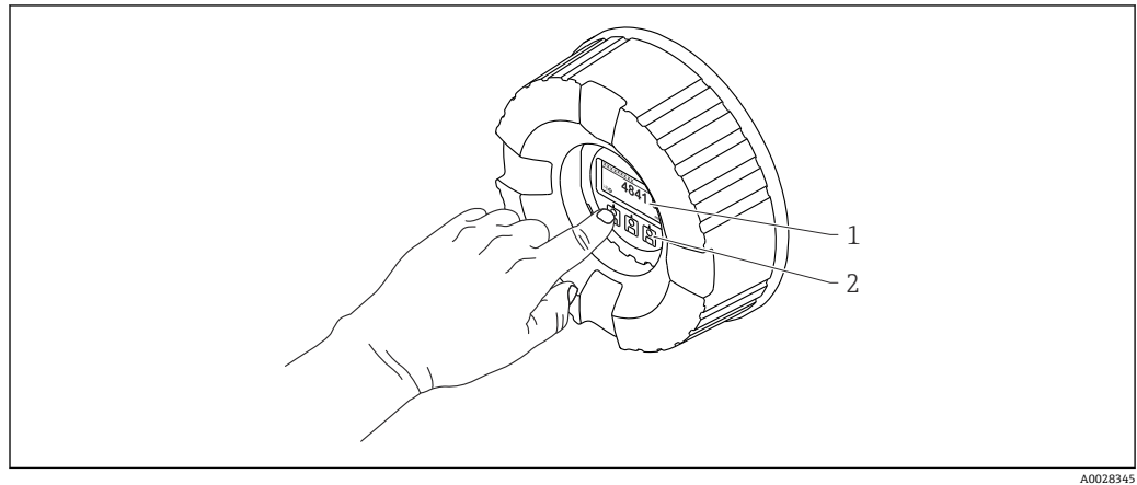
图 23 显示与操作单元
