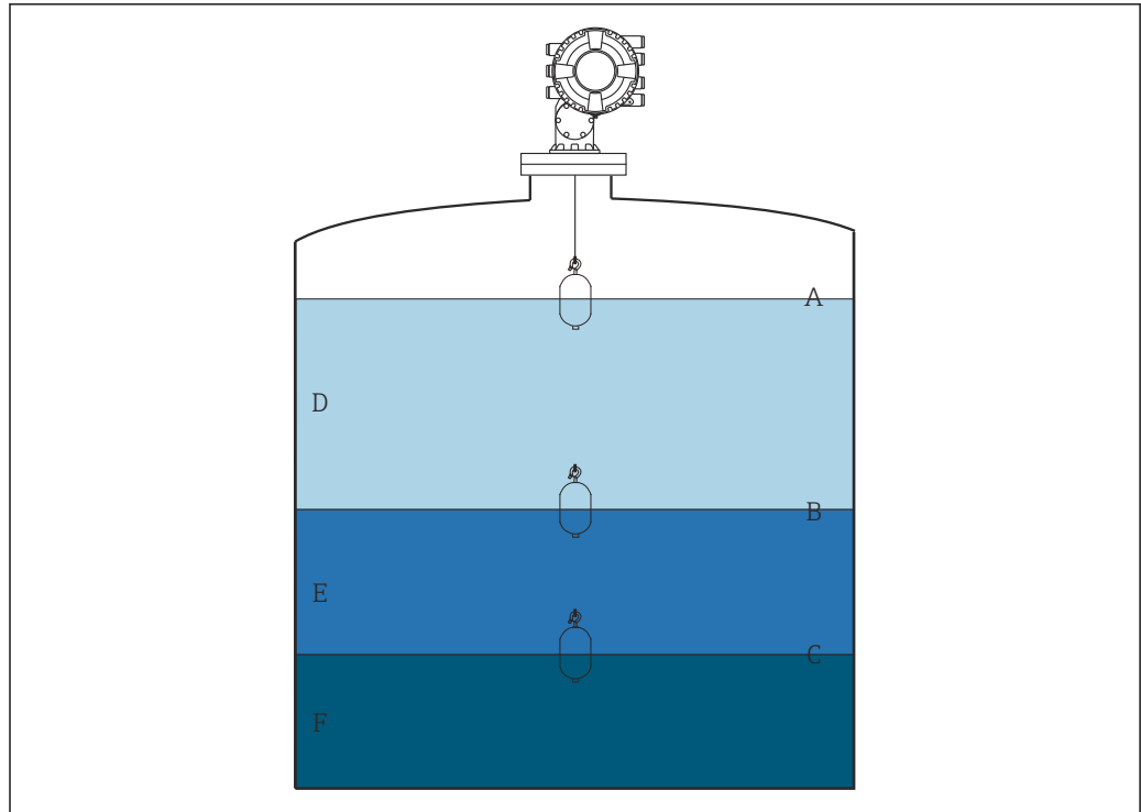
图 42 储罐设置示意图
