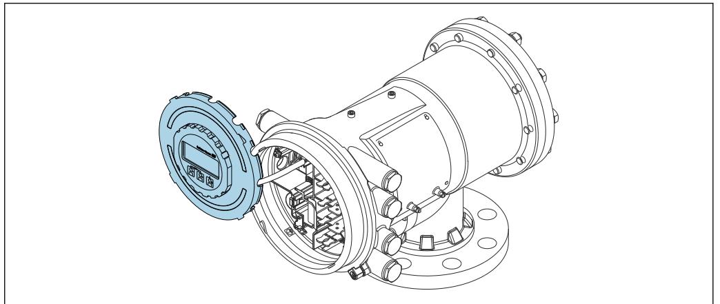
31 NMS83: 显示单元安装在接线腔边缘处
