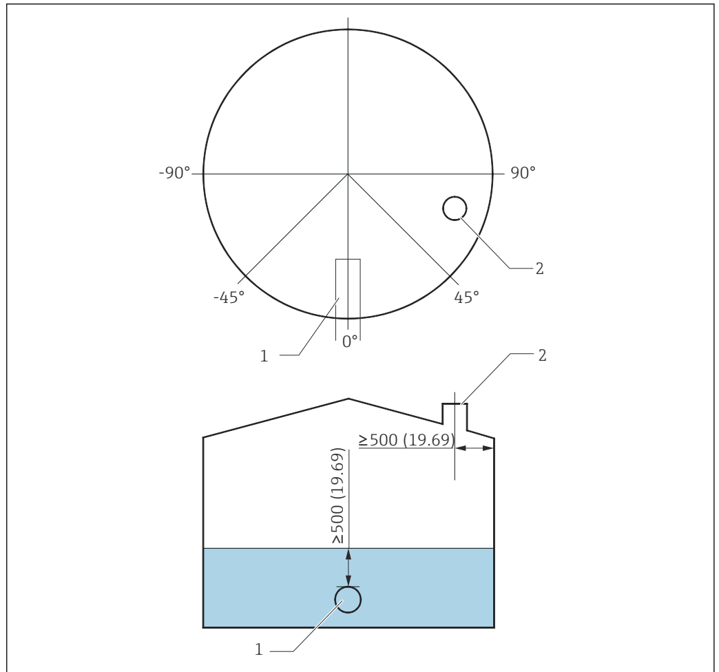
图 10 NMS8x 的推荐安装位置和最低测量液位；单位：mm (in)
