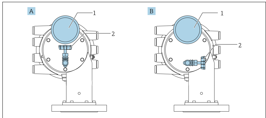
29 Montagelage von Überdruckventil und Druckanzeiger
