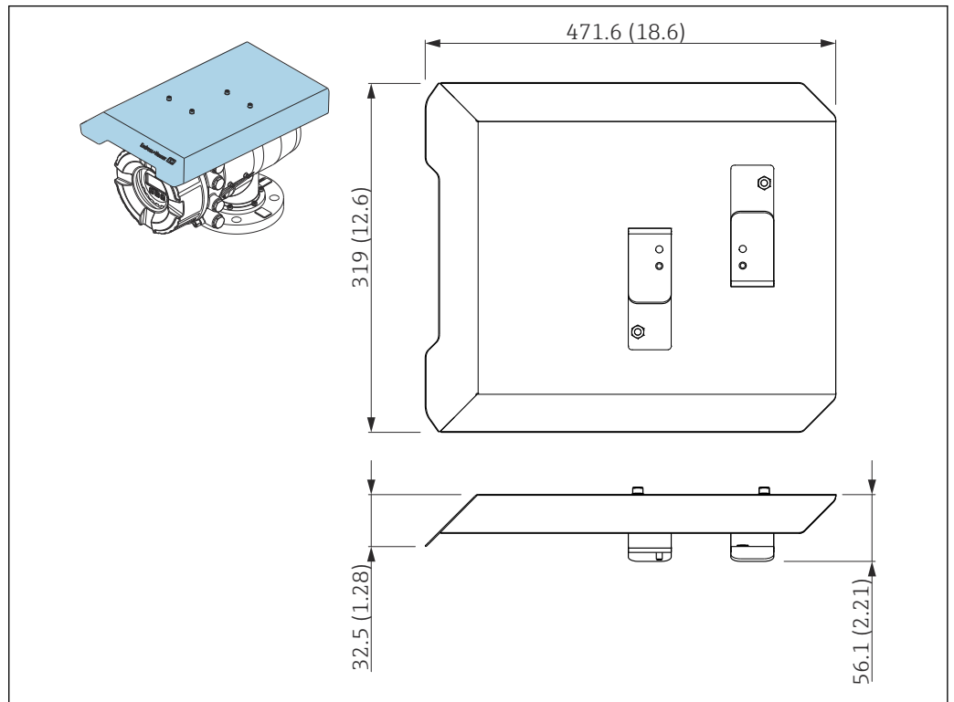
28 Wetterschutzhaube; Abmessungen: mm (in)
