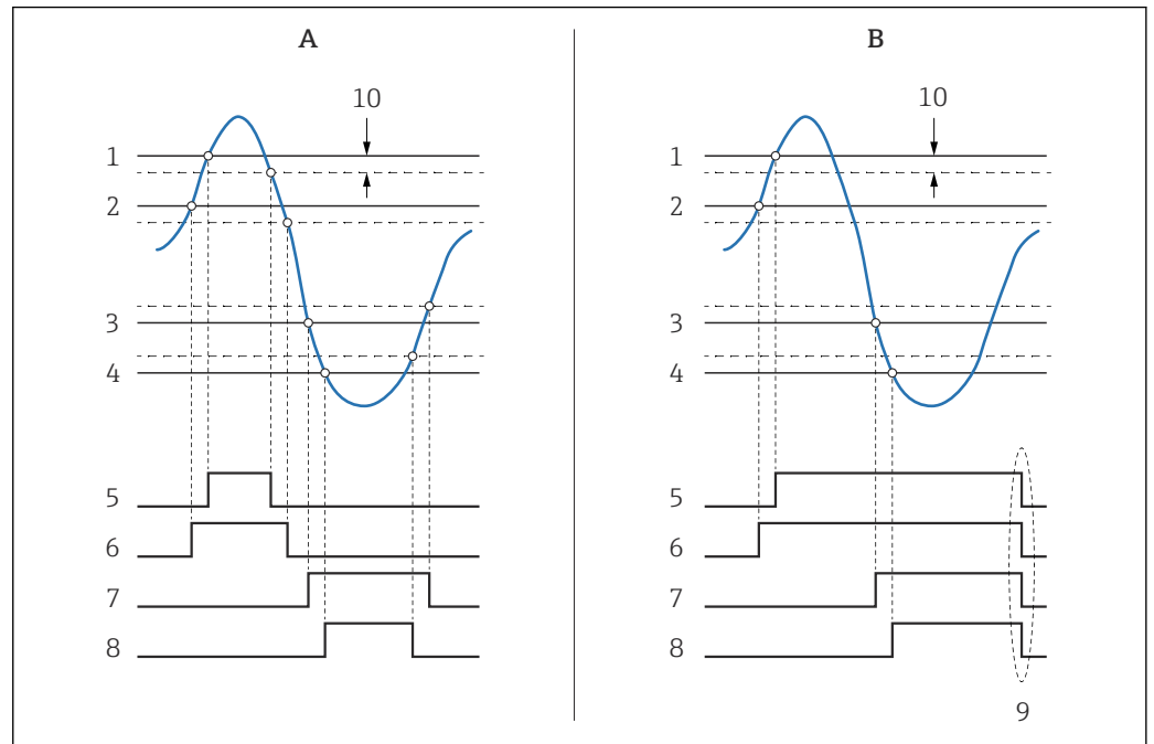
64 Princípio da avaliação de limite
