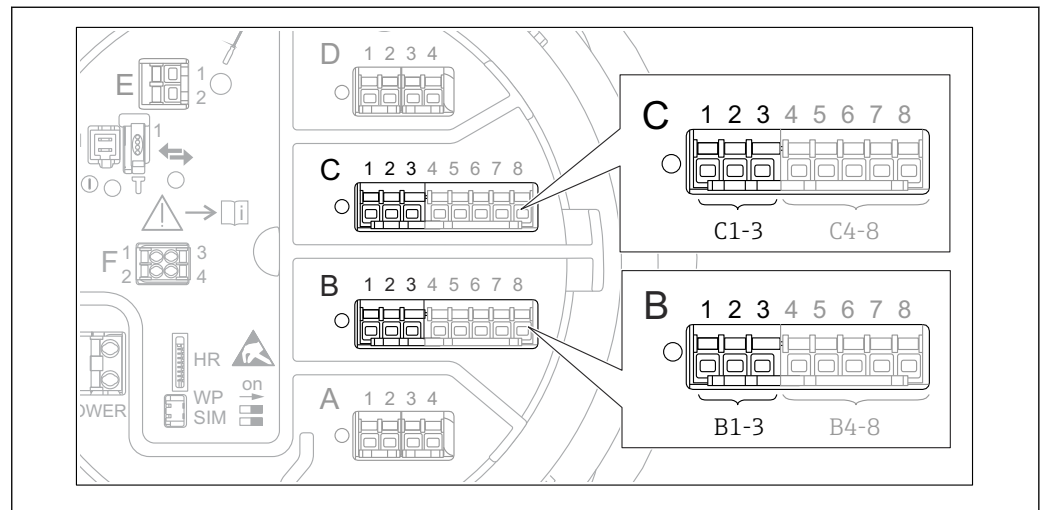
85 Terminais para a submenu "Analog I/O" ("B1-3" ou "C1-3", respectivamente)
