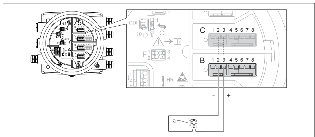
20 Utilização ativa do módulo de E/S analógica no modo de entrada
