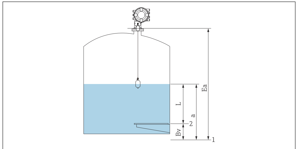
46 Tanque fechado para NMS83
