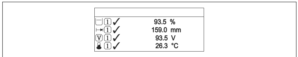
100 "Formato de exibição" = "4 valores"
