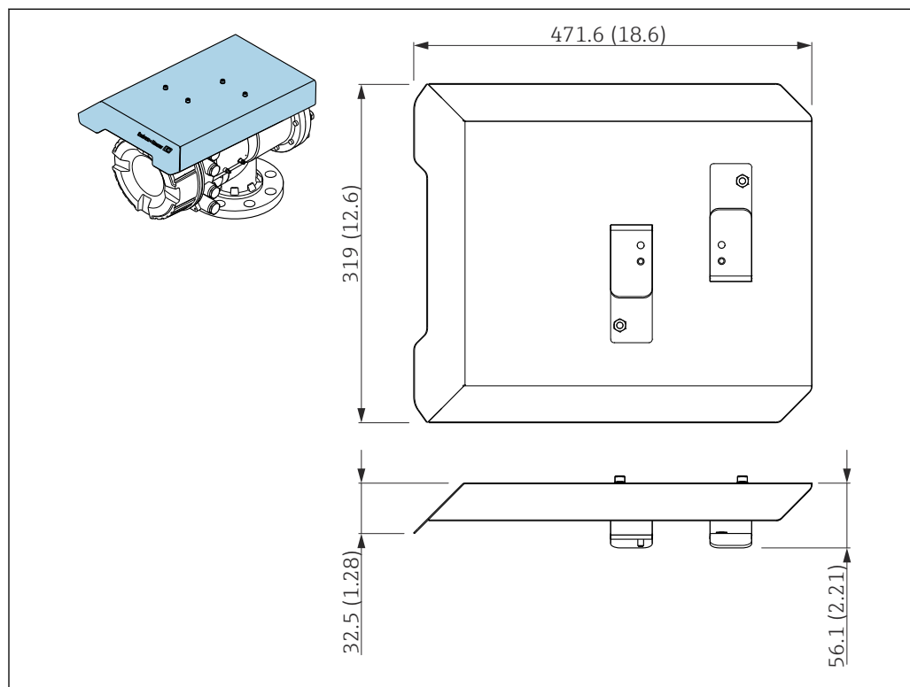
75 Tampa de proteção contra tempo, dimensões: mm (pol.)
