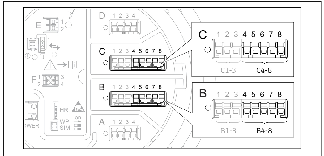
84 Terminais para a submenu "Analog IP" ("B4-8" ou "C4-8", respectivamente)
