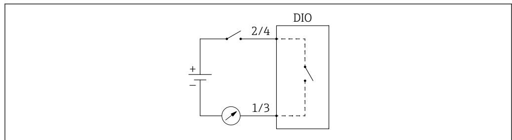
72 Utilização do módulo E/S digital como uma saída digital
