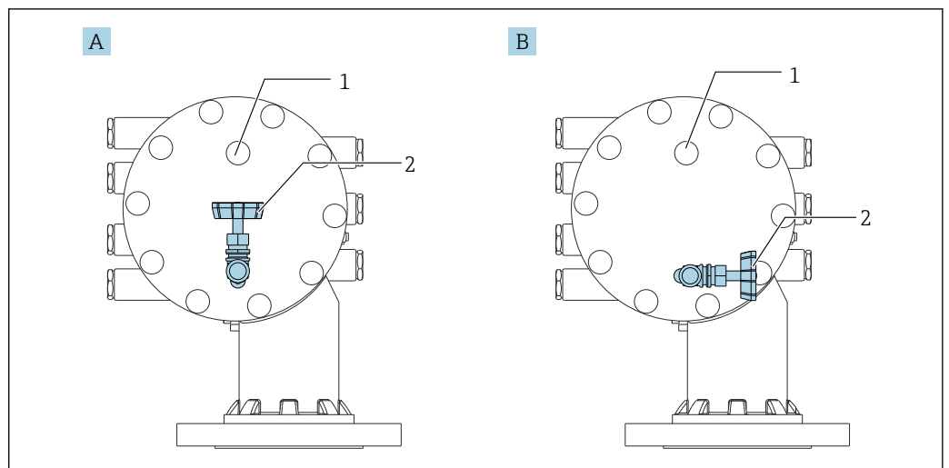
80 Bocal de limpeza e válvula de alívio
