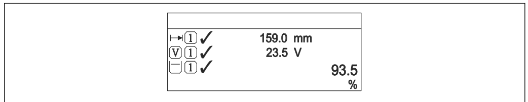
99 "Formato de exibição" = "1 valor grande + 2 valores"
