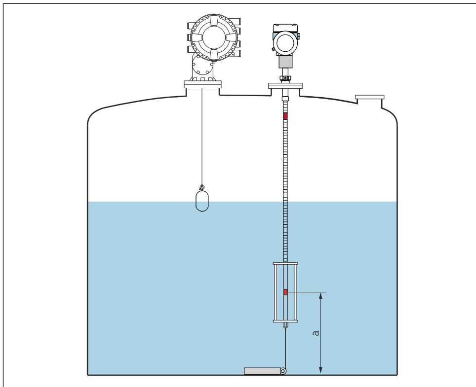
54 Prothermo NMT53x: Posição do elemento de temperatura de fundo
