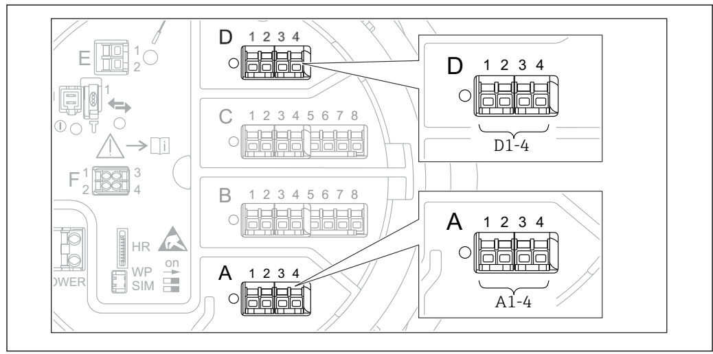
89 Designação dos módulos "Modbus", "V1" ou "WM550" (exemplos); dependendo da versão do equipamento, esses módulos também podem estar no slot B ou C.
