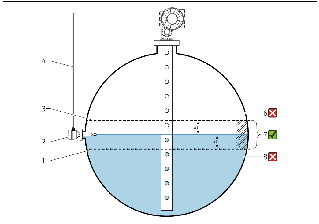
63 Exemplo de aplicação com chave de nível
