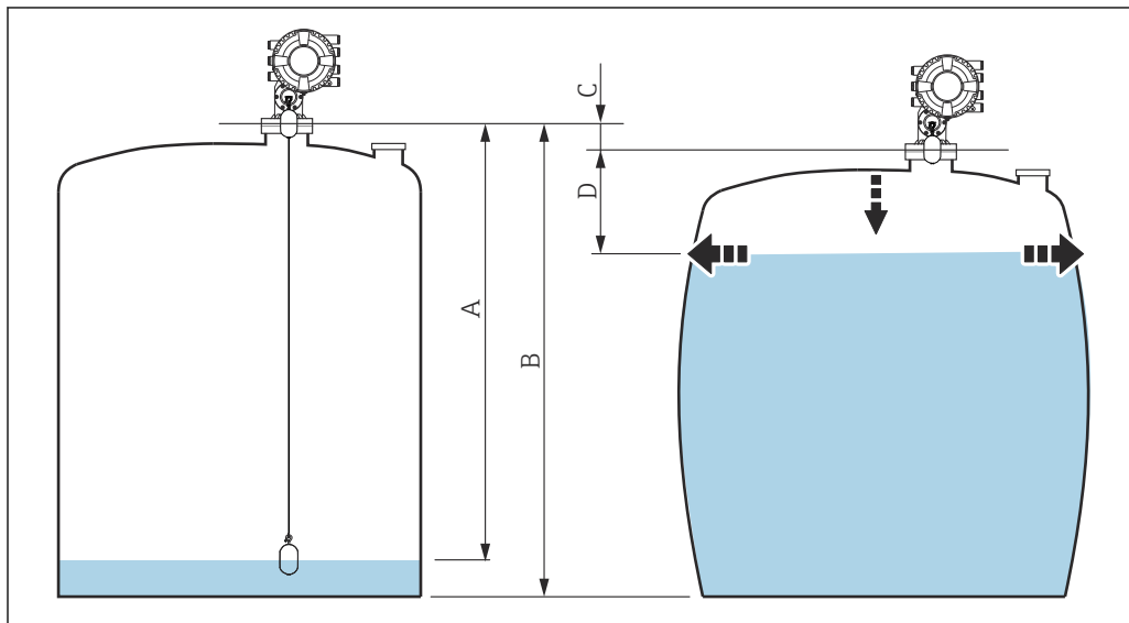
61 Correção da deformação hidrostática do tanque (HyTD)
