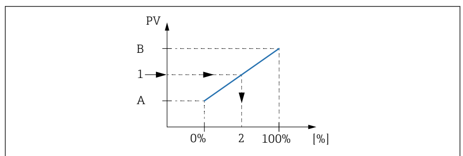
67 Escala da variável do tanque para a porcentagem
