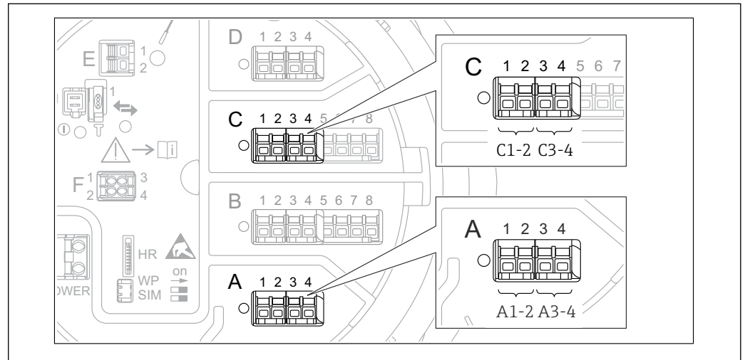
86 Designação das entradas ou saídas digitais (exemplos)
