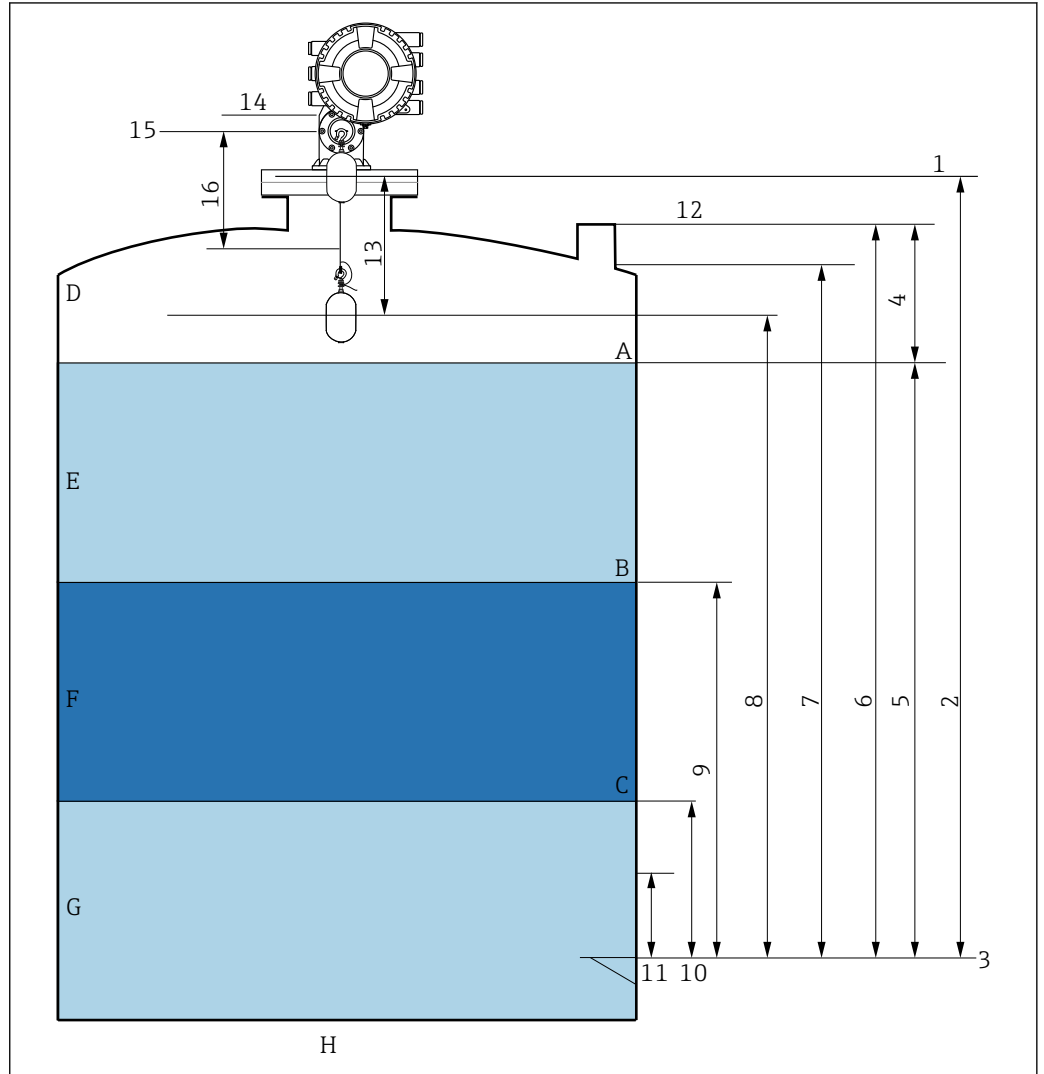
35 Termos relativos à instalação do NMS8x (ex. NMS81)
