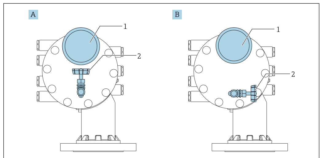
76 Posição de instalação da válvula de alívio e do medidor de pressão
