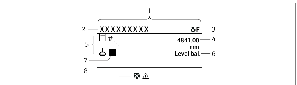
73 Aparência típica da visualização padrão (display do valor medido)
