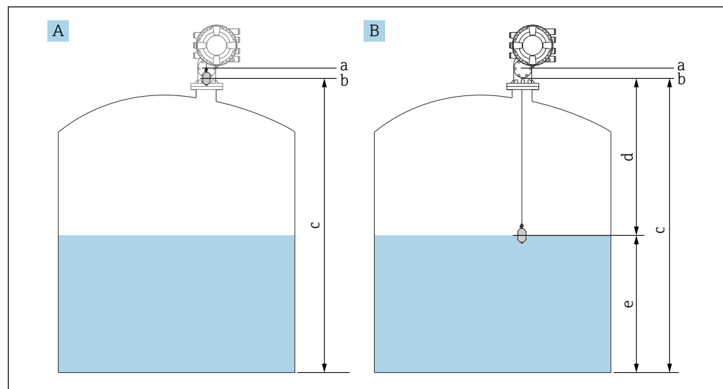
47 Ajuste do nível no caso de vazio (NMS83)
