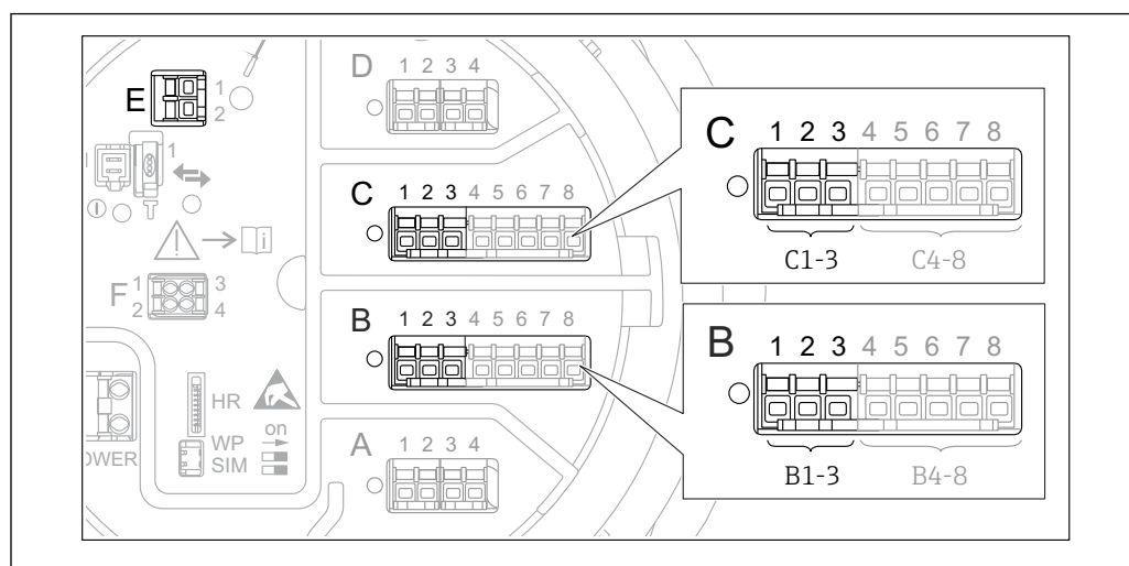
53 Possíveis terminais para malhas HART
