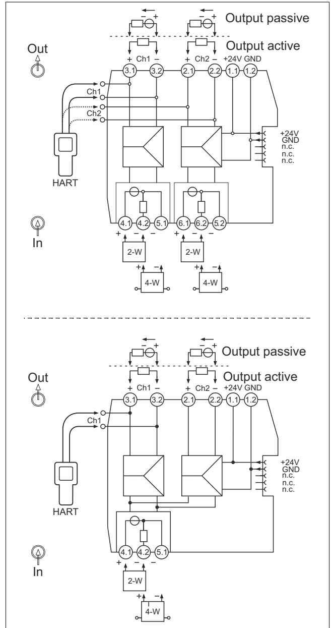
☐ 3 단자 할당: 1 및 2채널 버전(위), 신호 더블러(아래)
