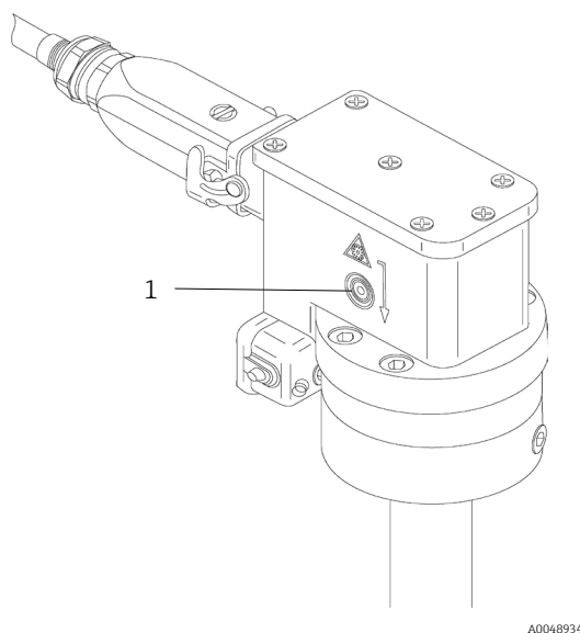
図 2. レーザー放射インジケータライトの位置 (1)
