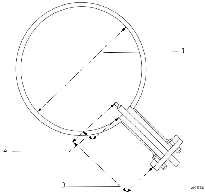
図 11. LNG バンカリング用の Rxn-41 プローブの設置パラメータ
