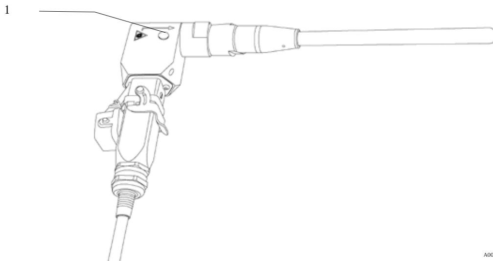
図 3. 直角ファイバーコネクタ (EO 方式) アセンブリ上にある LED レーザーインジケータ (1)
