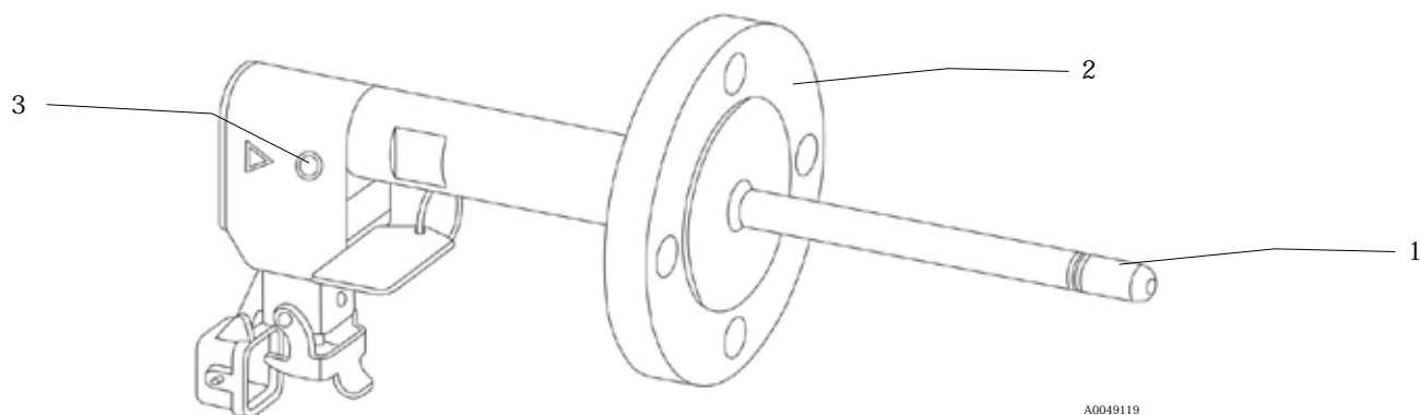
図 9. フランジ構成の Rxn-40 プローブ
