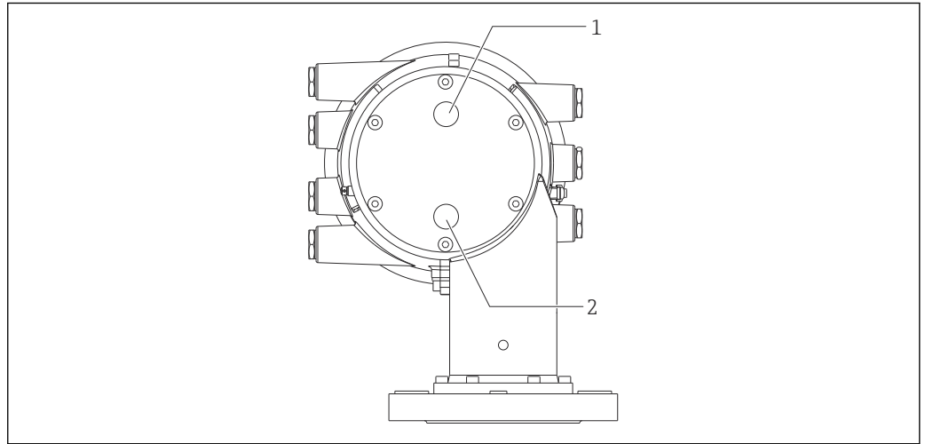
图 32 清洗短管和气体吹扫短管的连接孔口
