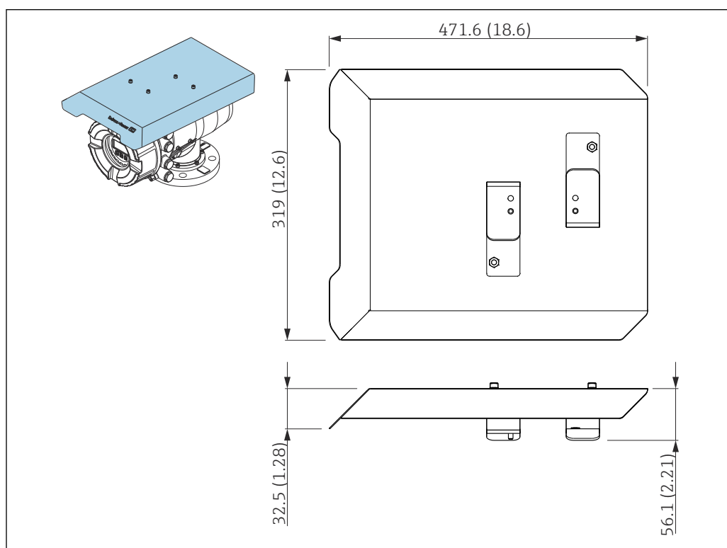
图 28 防护罩的外形尺寸示意图；单位：mm (in)
