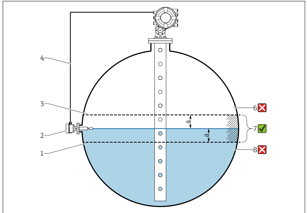
图 27 带液位开关的应用实例
