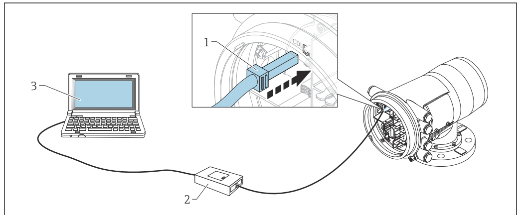
图 24 通过服务接口操作
