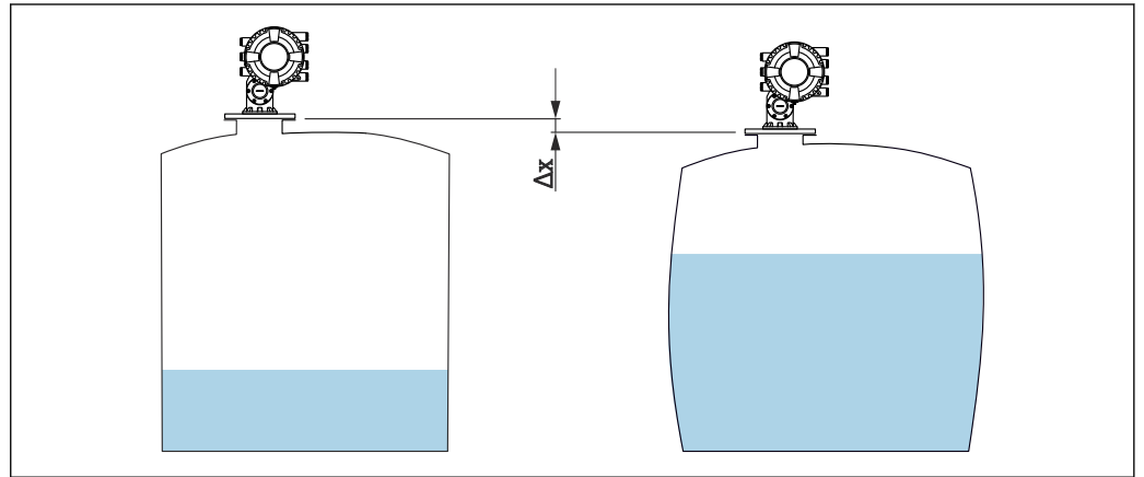
图 25 静压力导致罐体外壳膨胀，从而引起罐体参考高度位移 \Delta x
