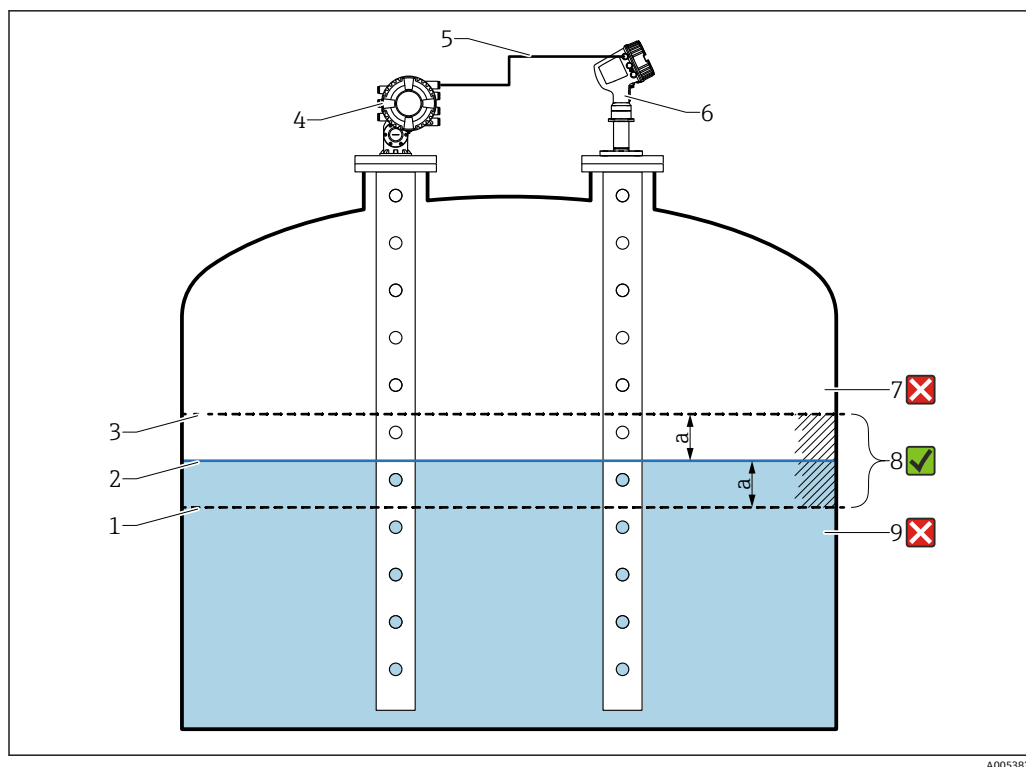
图 26 Proservo NMS8x 的应用实例
