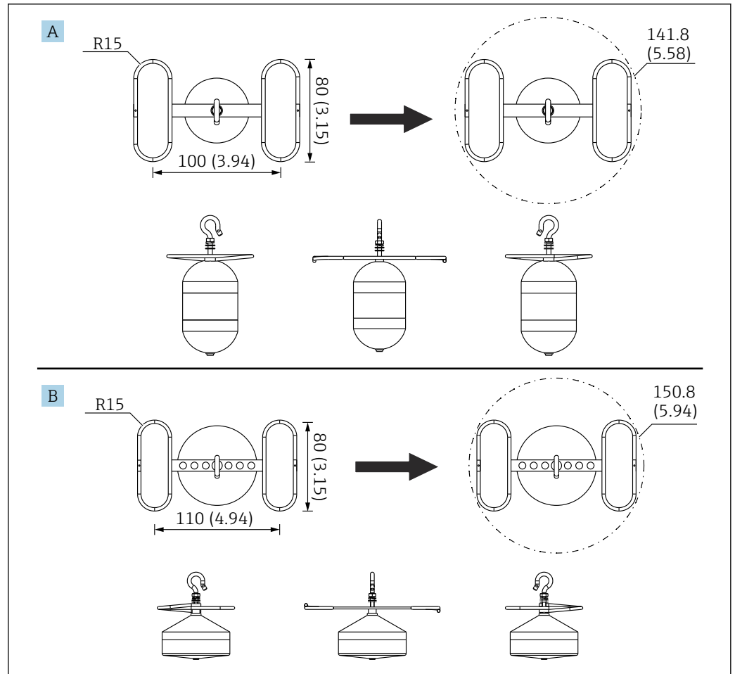
18 导向环
