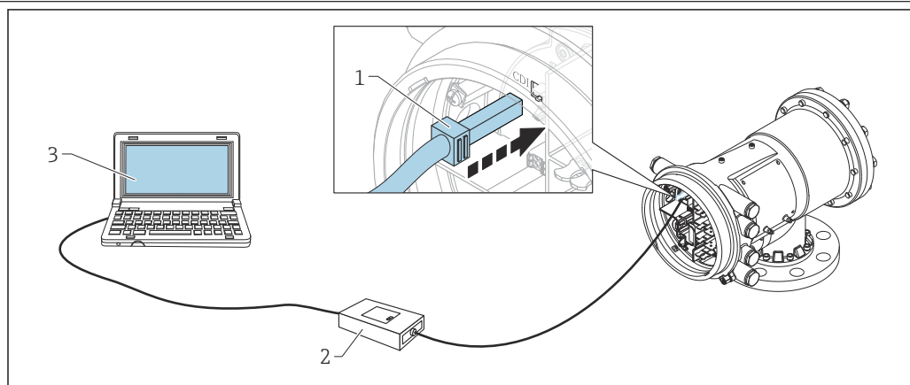
图 24 通过服务接口操作
