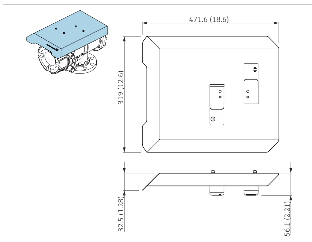
图 28 防护罩的外形尺寸示意图；单位：mm (in)
