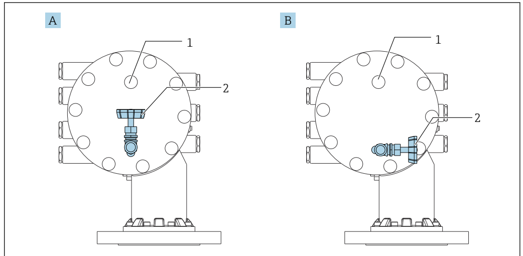
图 33 清洗短管和减压阀
