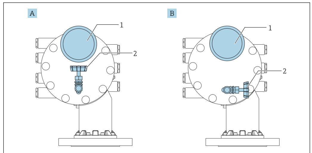
图 29 减压阀和压力表的安装位置
