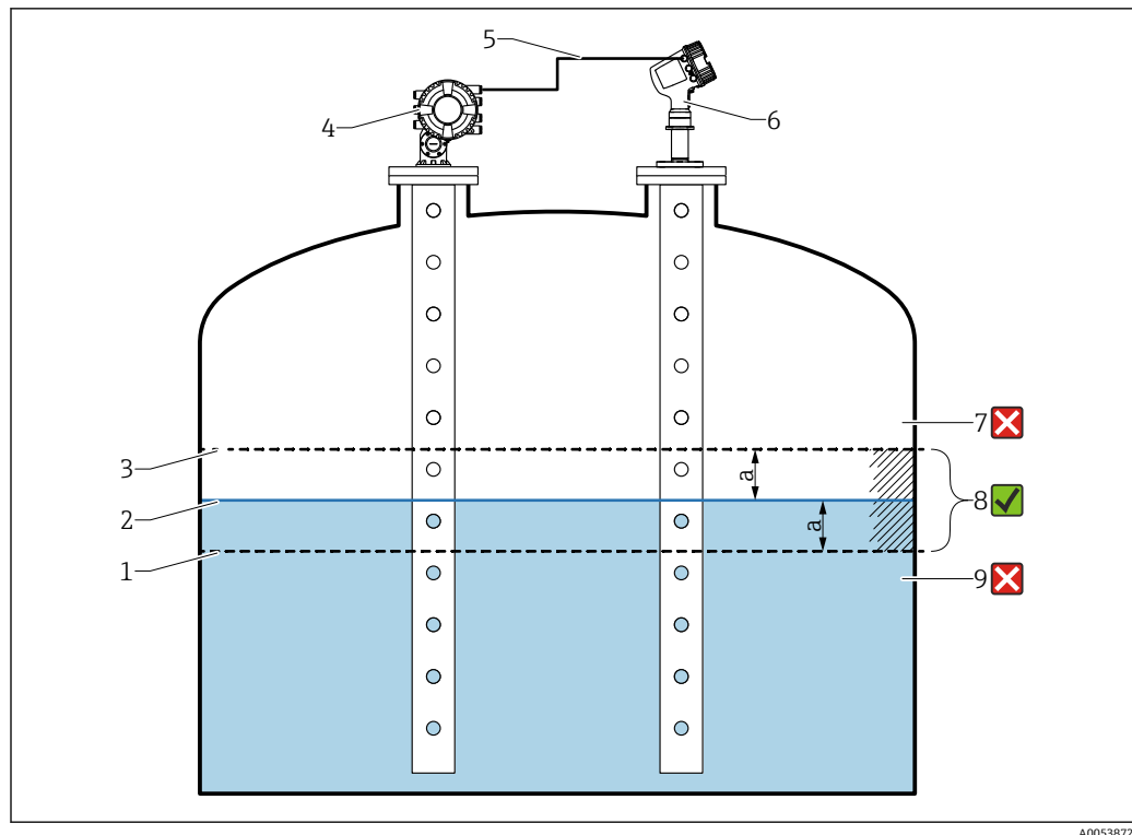
图 26 Proservo NMS8x 的应用实例
