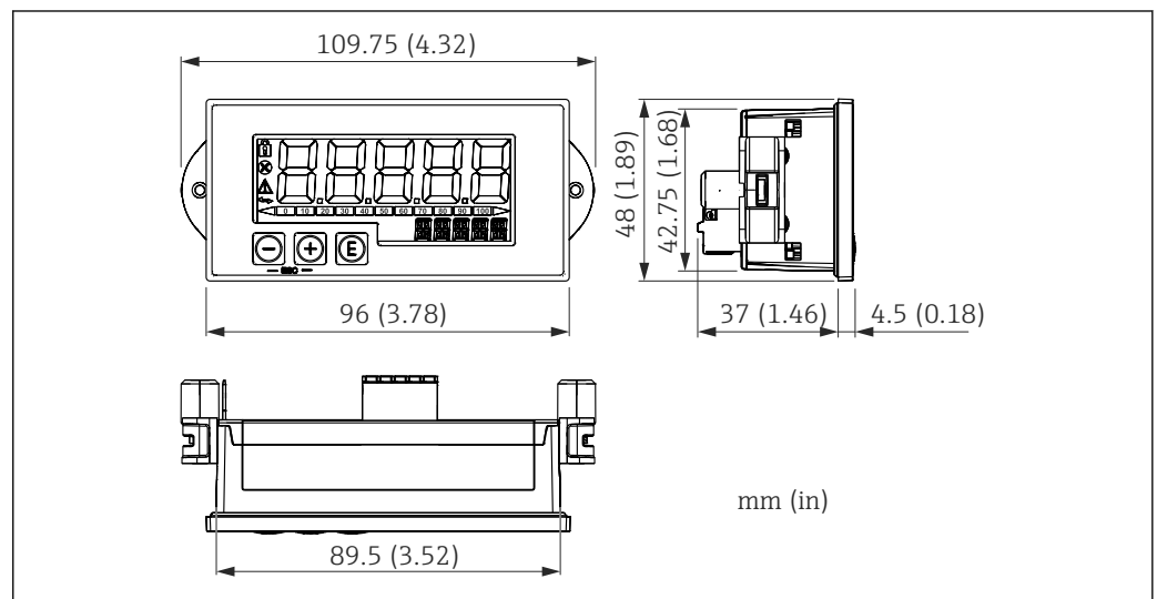
26 Dimensioni della custodia per montaggio a fronte quadro
