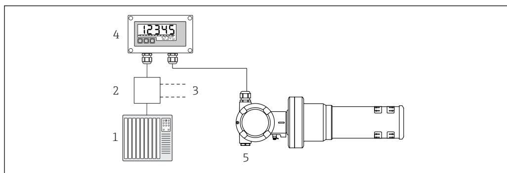
Fig. 6 Funzionamento a distanza di FMG50 tramite RIA15
