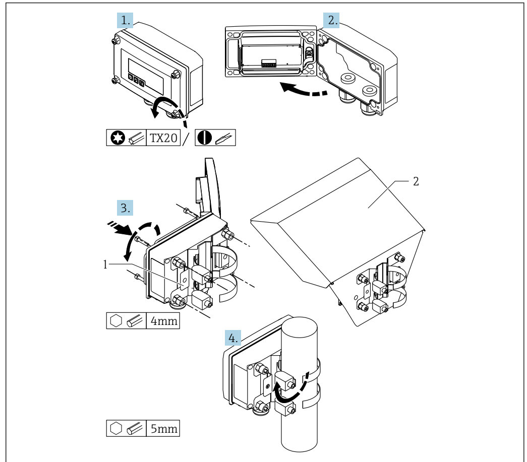
12 Montaggio su palina dell'indicatore di processo
