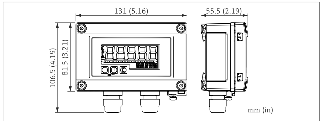
27 Dimensioni della custodia da campo con ingresso cavi (M16)
