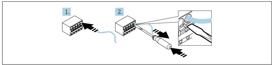
15 Funzionamento dei morsetti a molla
