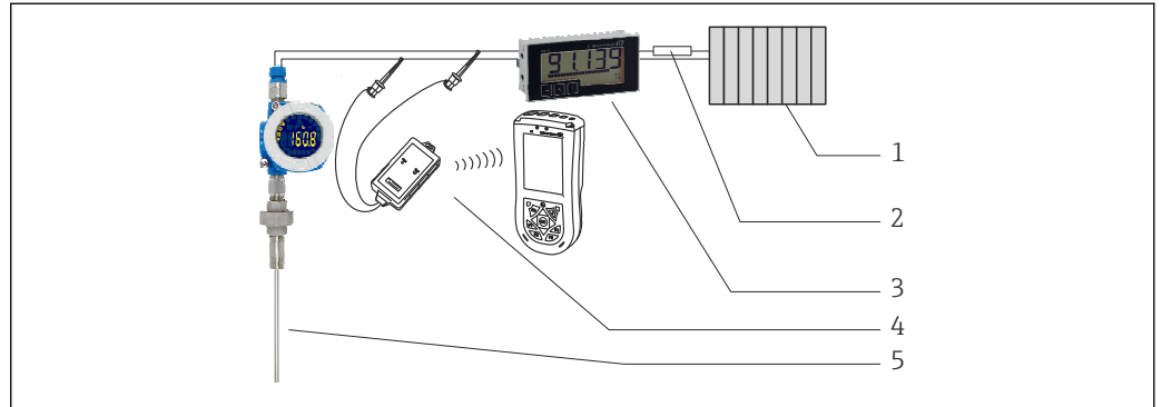
16 Configurazione dei dispositivi HART; esempio iTEMP TMT162
