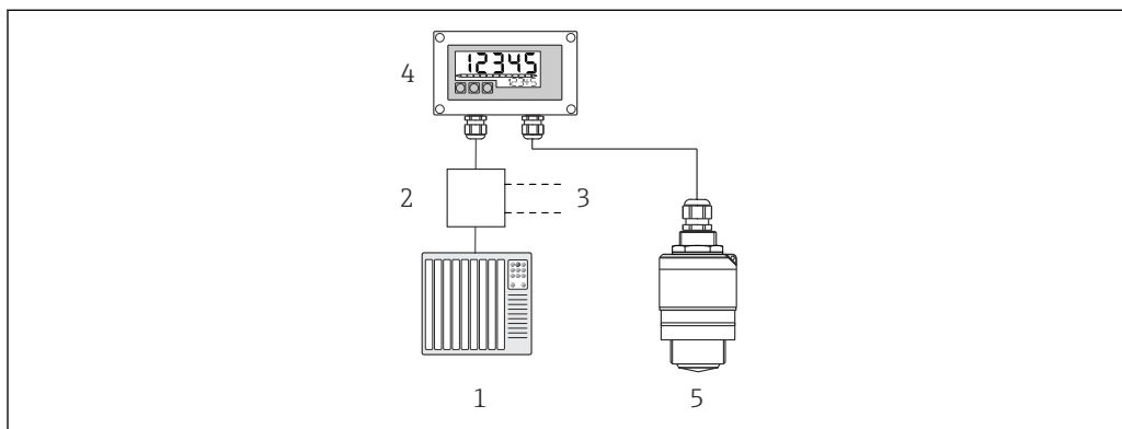
2 Funzionamento a distanza di Micropilot mediante RIA15
