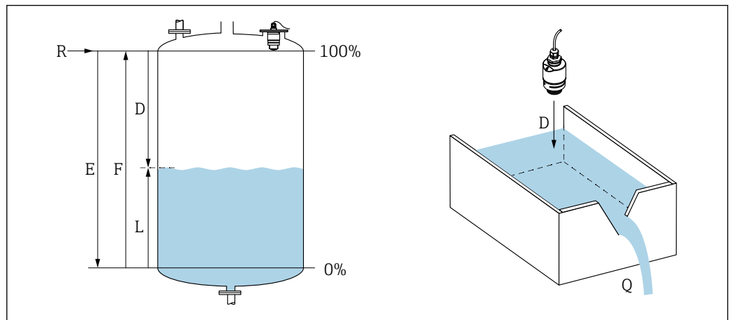
1 Parametro di taratura con Micropilot
