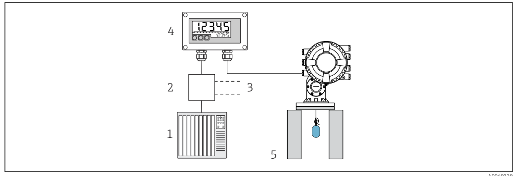
8 Funzionamento a distanza di NMS8x tramite RIA15
