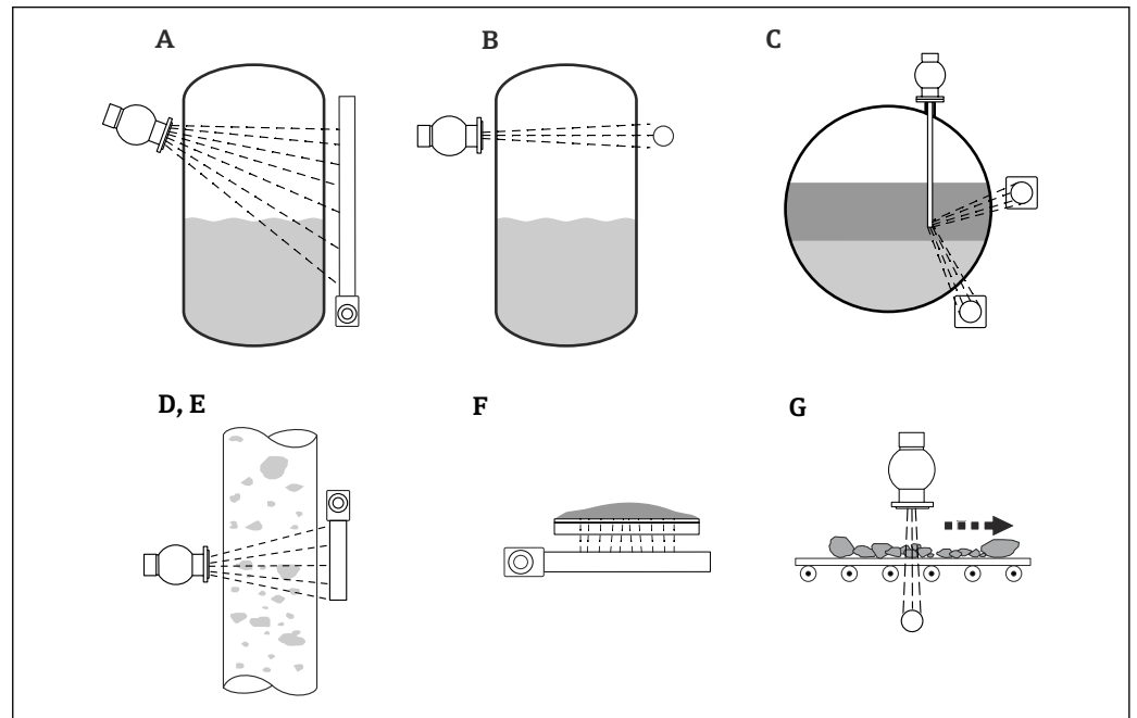
5 Operazioni di misura di Gammapilot FMG50
