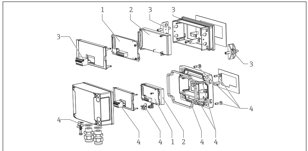
22 Parti di ricambio dell'indicatore di processo
