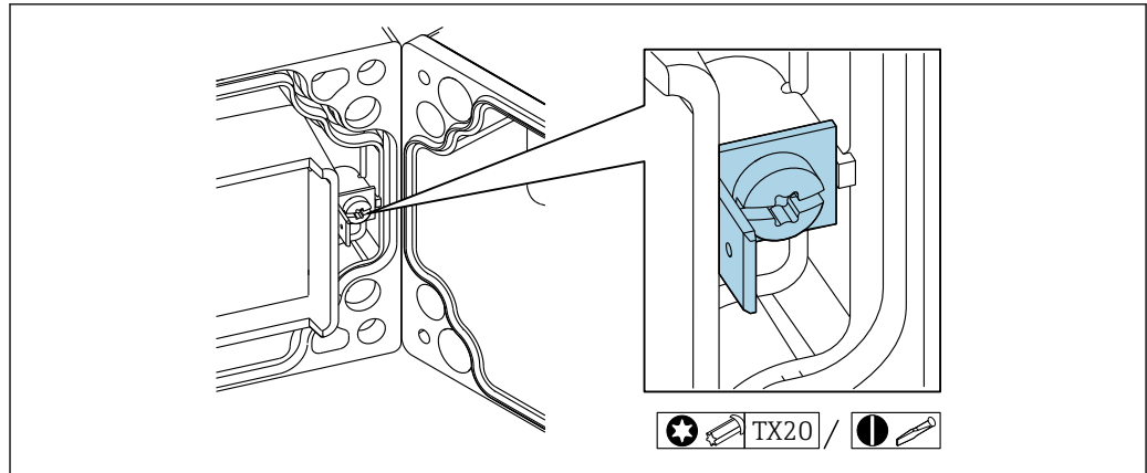
19 Messa a terra funzionale: morsetto di terra nella custodia da campo
