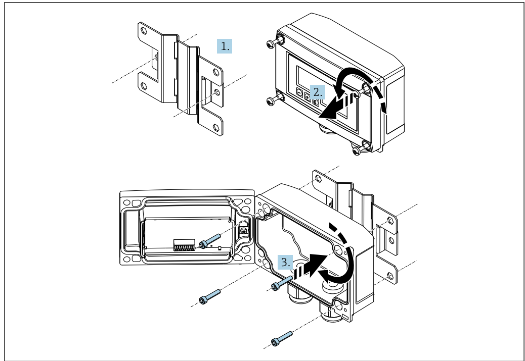
图 13 在墙上安装回路显示仪
