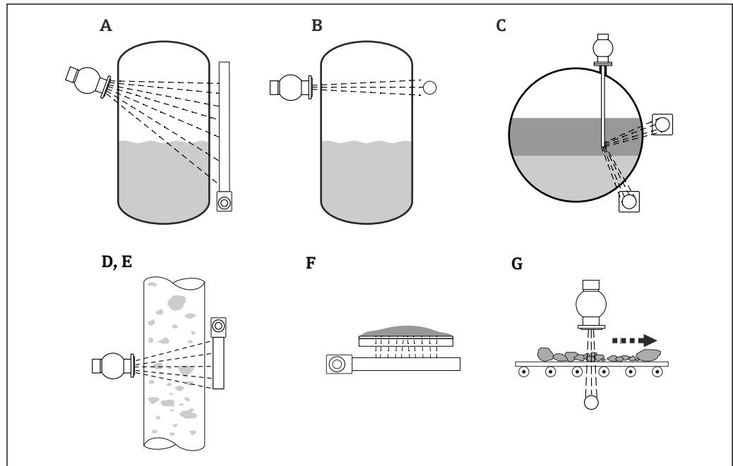
图 5 Gammapilot FMG50 的测量任务
