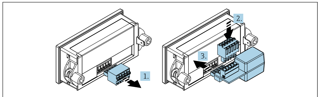
图 14 安装可选 HART 通信电阻模块
