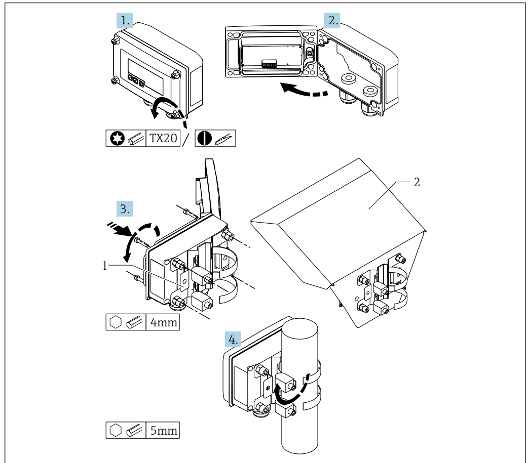
图 12 在管道上安装回路显示器
