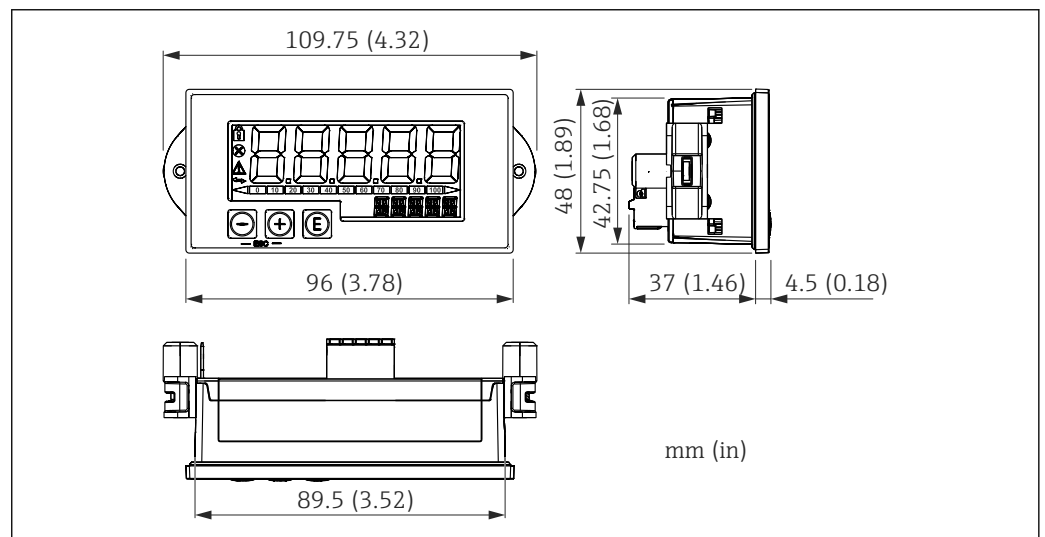
图 26 盘装型外壳的外形尺寸
