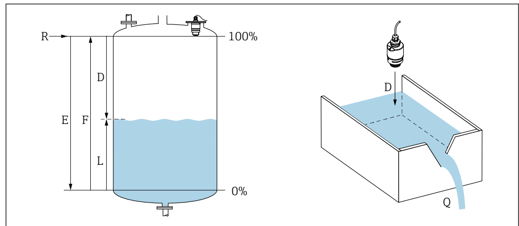
图 1 标定参数 Micropilot
