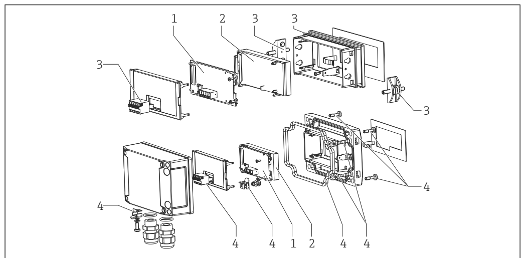
图 22 回路显示仪备件
