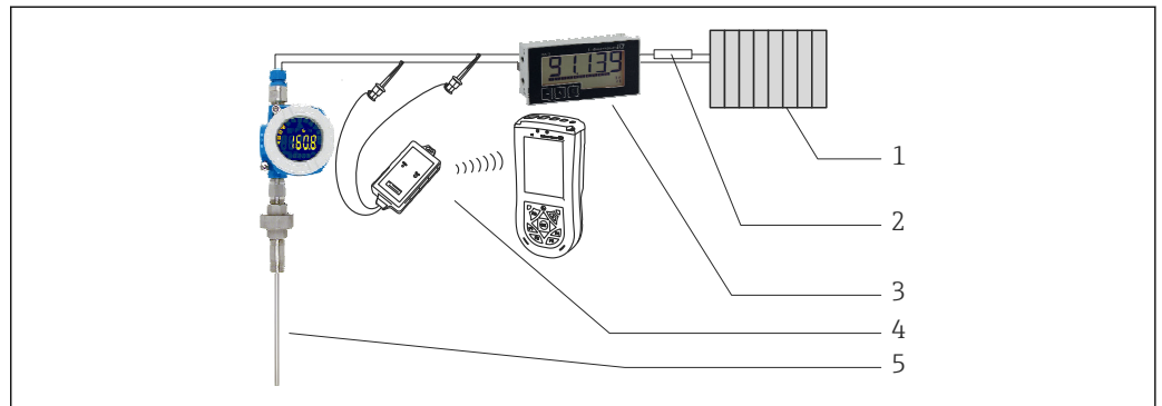
图 16 设置 HART 设备，示例 iTEMP TMT162
