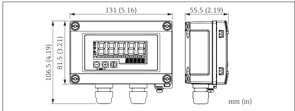
图 27 现场型外壳的外形尺寸，包括缆塞 (M16)
