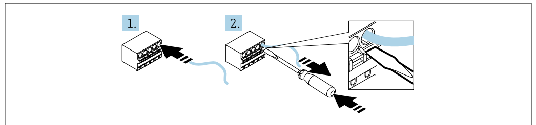
图 15 弹簧端子的操作
