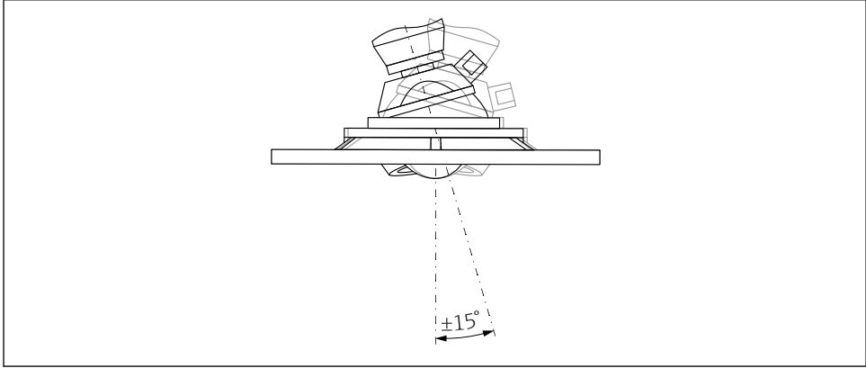
2 Antenna a cono flush mounted con unità di puntamento
