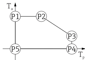
▣ 36 Boîtier plastique ; température de process 0 ... +150 °C (+32 ... +302 °F) avec agrément CSA C/US
