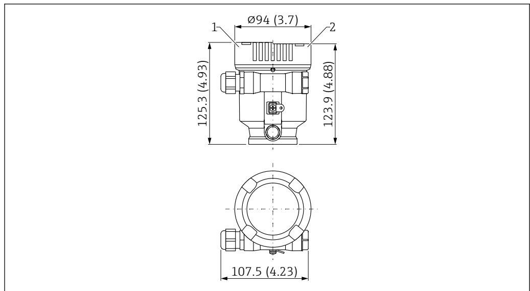
61 Dimensions ; boîtier à simple compartiment, plastique ; avec raccord M20 et bouchon, plastique. Unité de mesure mm (in)
