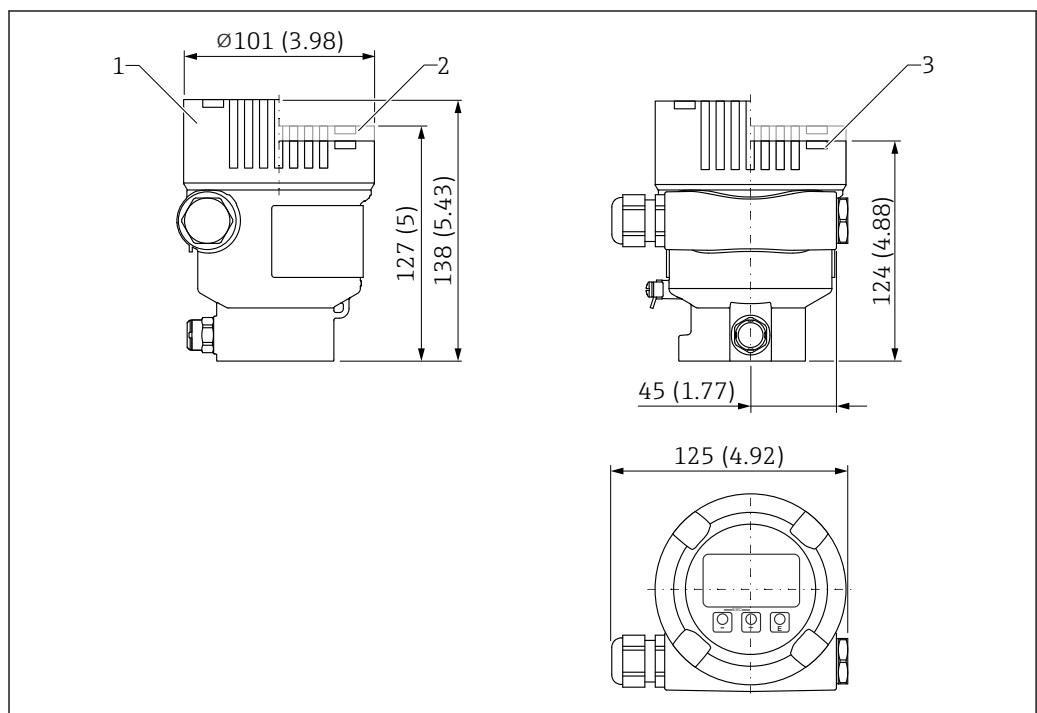
62 Dimensions ; boîtier à simple compartiment, aluminium, revêtu ; avec raccord M20 et bouchon, plastique. Unité de mesure mm (in)
