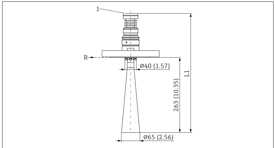
67 Dimensions de l'antenne cornet DN65 - raccord process à bride. Unité de mesure mm (in)
