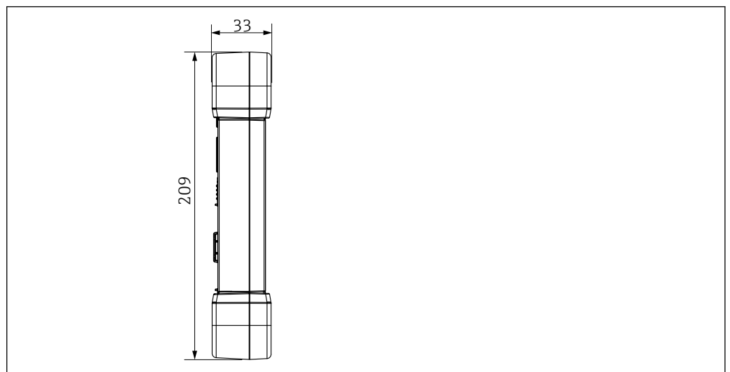
11 側面図
