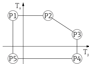
▣ 26 Корпус 316L, гигиенический; рабочая температура -40 до +80 °C ( -40 до +176 °F)
