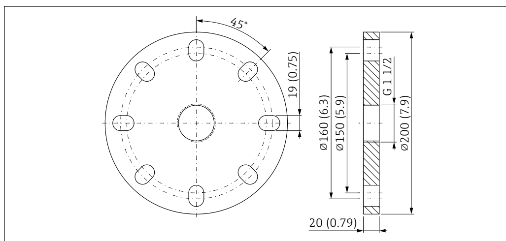
41 Размеры фланца UNI 3 дюйма/DN80/80A. Единица измерения мм (дюйм)
