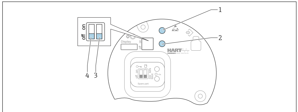
46 Кнопки управления и DIP-переключатели на электронной вставке HART
