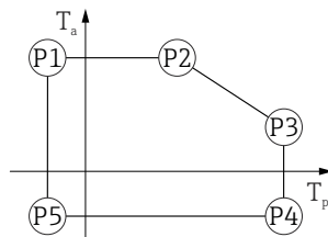
▣ 27 Корпус 316L, гигиенический; рабочая температура -40 до +130 °C ( -40 до +266 °F)
