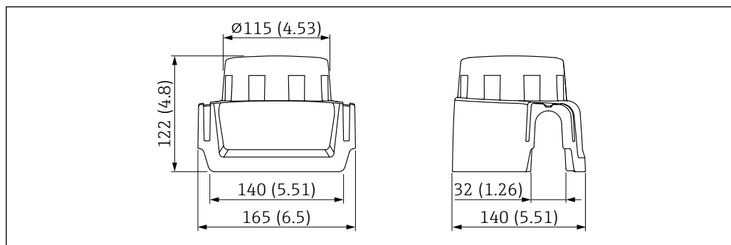
49 Размеры козырька для защиты от атмосферных воздействий, пластмассовый, XW111. Единица измерения мм (дюйм)
