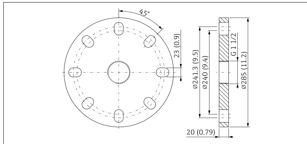
43 Размеры фланца UNI 6 дюймов/DN150/150A. Единица измерения мм (дюйм)
