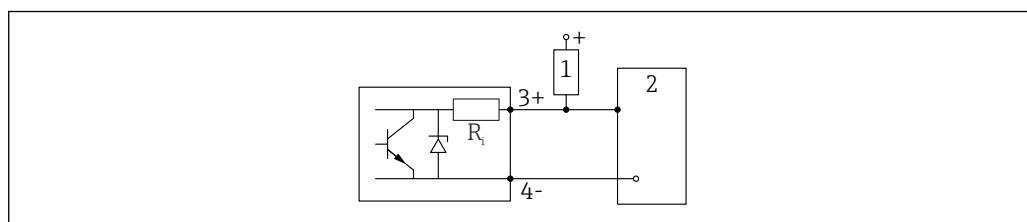
14 Пример подключения через цифровой вход
