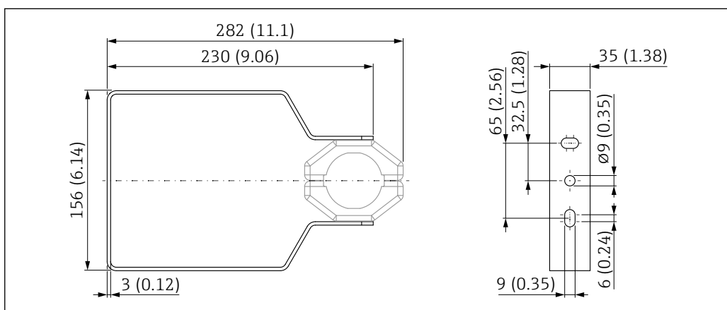
51 Размеры; регулируемый монтажный кронштейн FMR6xB. Единица измерения мм (дюйм)
