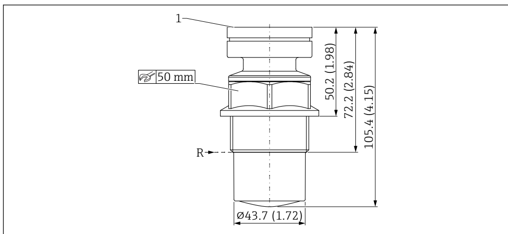
34 Размеры герметичной антенны, PVDF, 40 мм (1,5 дюйм). Единица измерения мм (дюйм)
