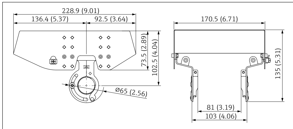
48 Размеры козырька для защиты от атмосферных воздействий: сталь 316L, XW112. Единица измерения мм (дюйм)
