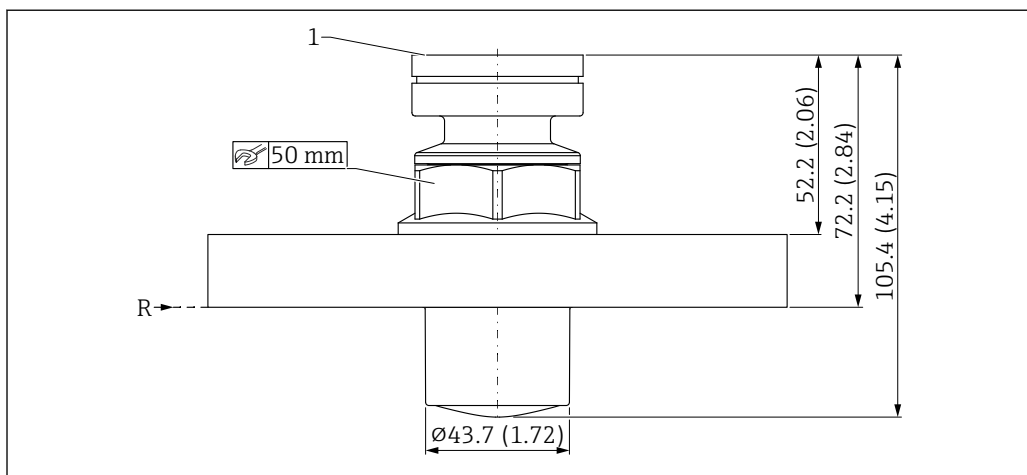
35 Размеры герметизированной антенны, PVDF, 40 мм (1,5 дюйм), присоединение к процессу – фланец UNI. Единица измерения мм (дюйм)
