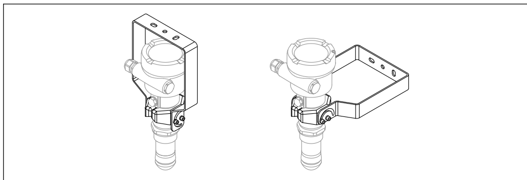
50 Регулируемый монтажный кронштейн FMR6xB; потолочный или настенный монтаж
