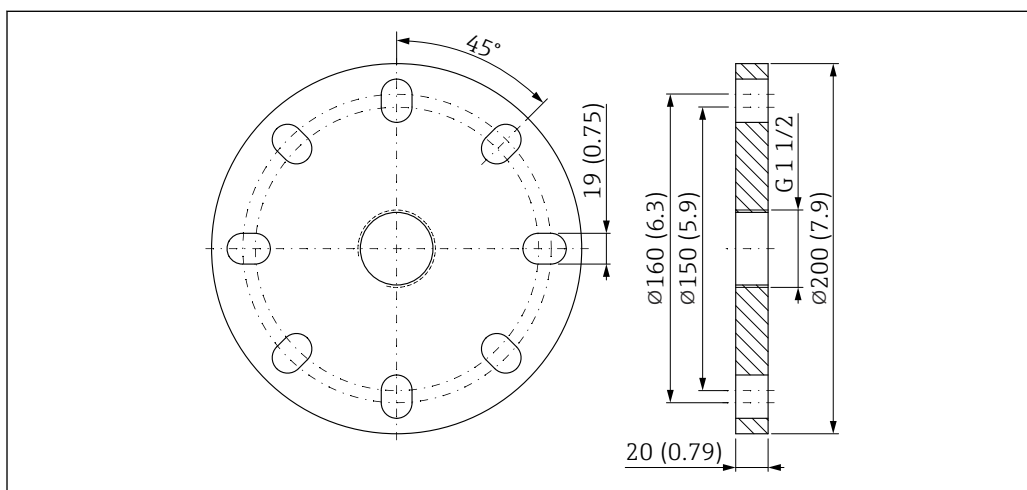
36 Размеры фланца UNI 3 дюйма/DN80/80A. Единица измерения мм (дюйм)
