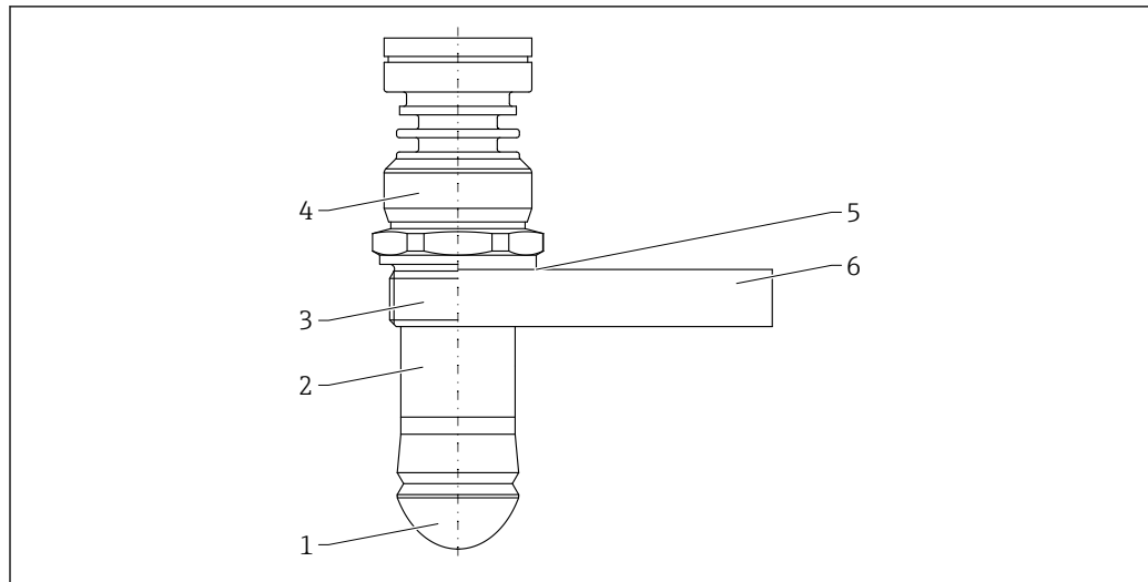
45 Материал; антенна с защитой от конденсата 50 мм (2 дюйм)
