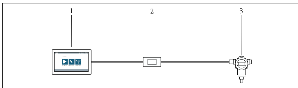
図 5 フィールド機器との CDI ポイント・トゥー・ポイント接続
