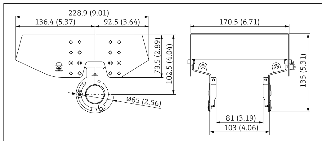
48 Dimensões da tampa de proteção contra tempo: 316 L, XW112. Unidade de medida mm (in)
