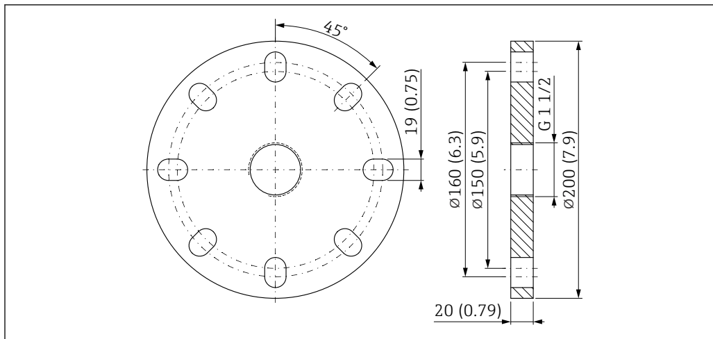
36 Dimensões da flange UNI 3"/DN80/80A. Unidade de medida mm (in)
