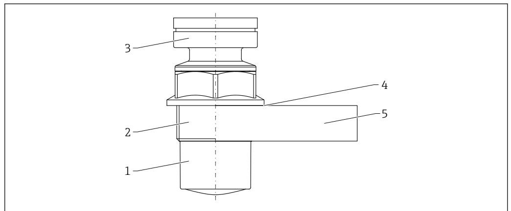
44 Material: antena encapsulada de PVDF, 40 mm (1.5 in)
