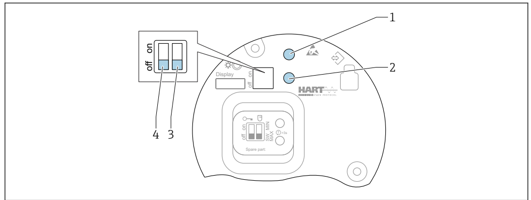
46 Teclas de operação e minisseletoras na unidade eletrônica HART
