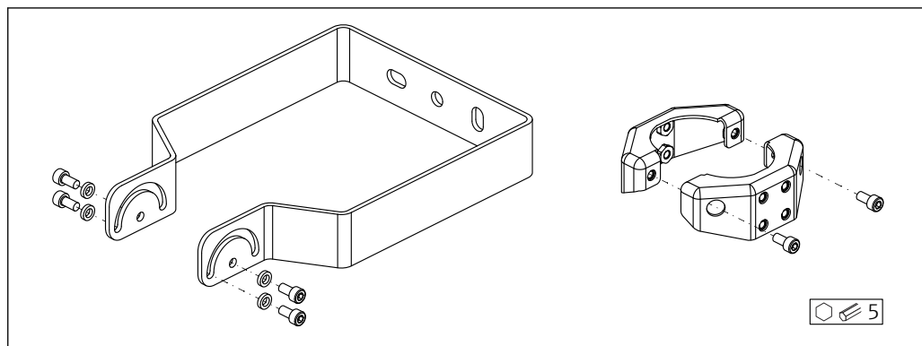
52 Escopo de entrega; suporte de montagem ajustável FMR6xB
