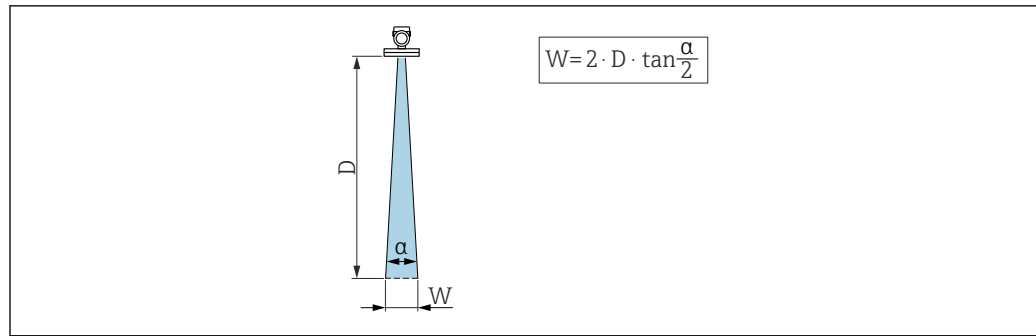
17 Relação entre o ângulo do feixe \alpha , a distância D e o diâmetro do feixe W
