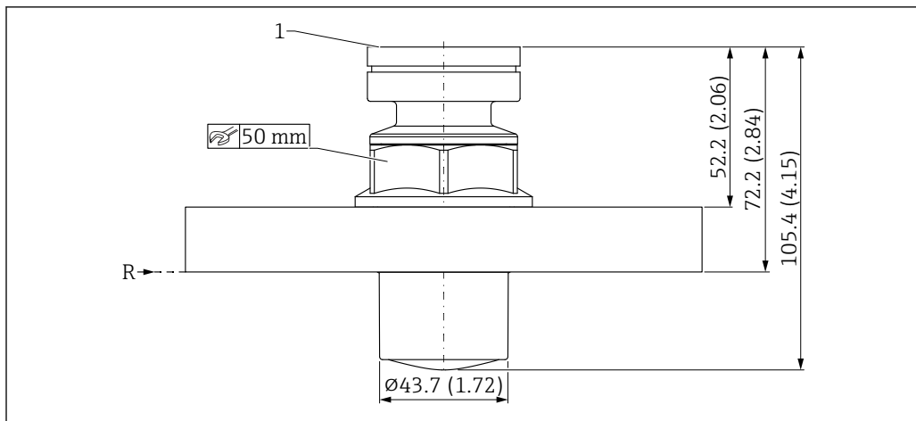
35 Dimensões da antena encapsulada, PVDF, 40 mm (1.5 in), conexão de processo flange UNI. Unidade de medida mm (in)
