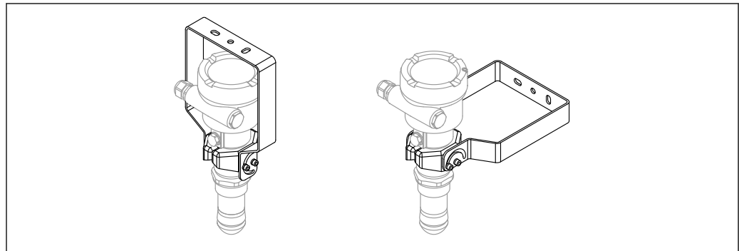
50 Suporte de montagem ajustável FMR6xB; montagem no teto ou em parede
