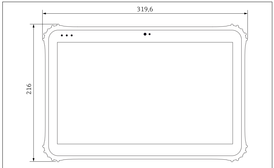
10 Вид спереди
