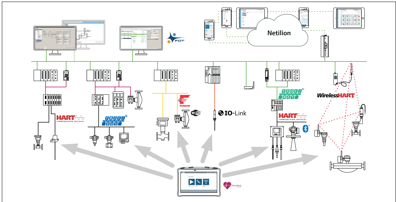
图 1 Field Xpert SMT70 的应用
