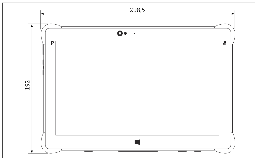
図 10 前面図
