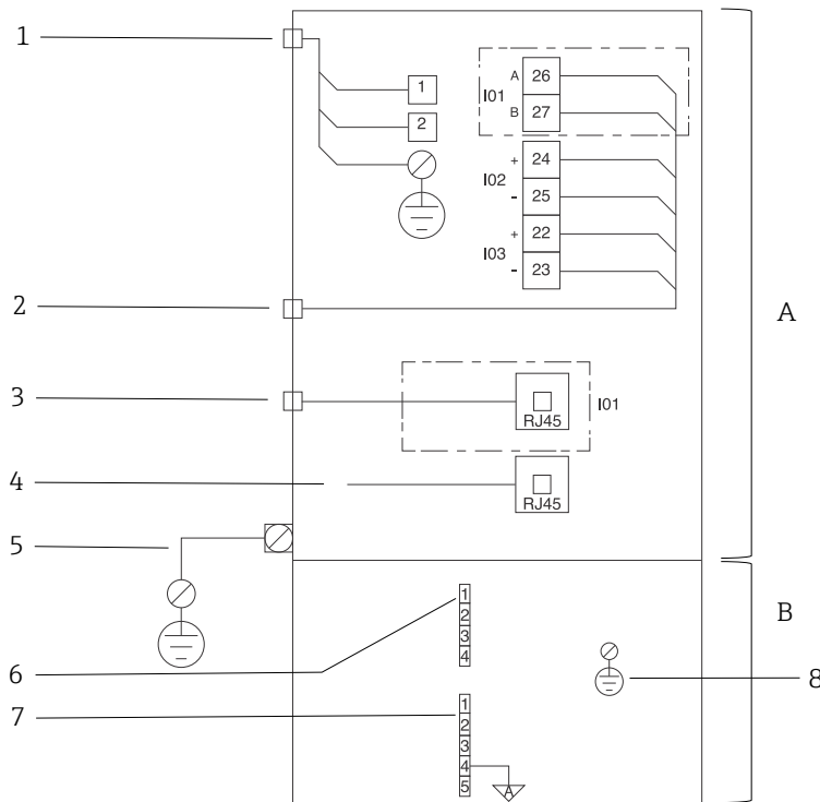
Рисунок 16. Электрические соединения анализатора JT33
