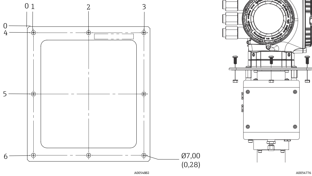
Рисунок 10. Монтажная пластина для установки корпуса и крепежные элементы. Единицы измерения: мм (дюймы)
