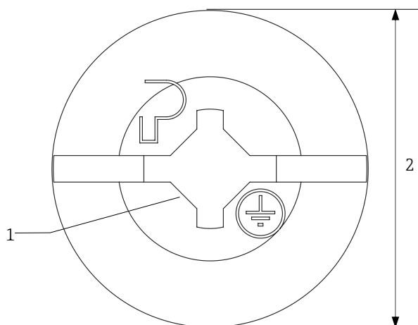
Рисунок 17. Винт заземления корпуса MAC
