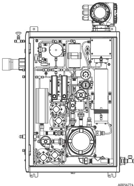
Рисунок 8. Газоанализатор JT33 типа TDLAS
