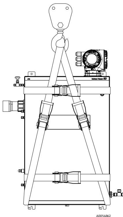
Рисунок 4. Анализатор JT33, оснащенный ремнями с храповиком для подъема и перемещения
