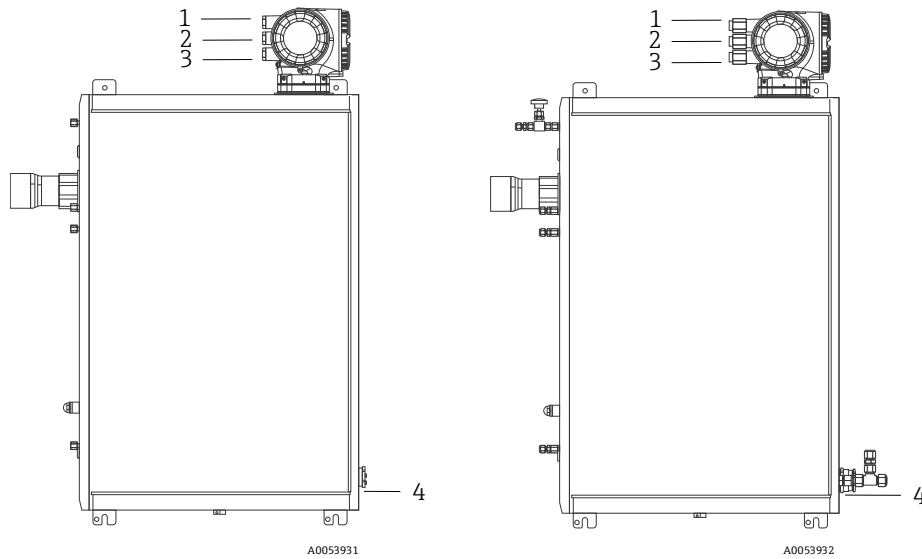
Рисунок 20. Резьбовые вводы на анализаторах JT33: ATEX (слева) и CSA (справа)
