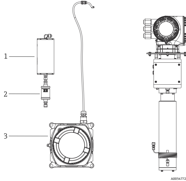
Рисунок 6. Спектрометр JT33 типа TDLAS, MAC, скруббер и индикатор
