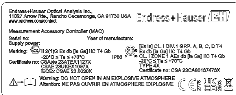
Рисунок 2. Заводская табличка MAC с разрешениями и предупреждениями
