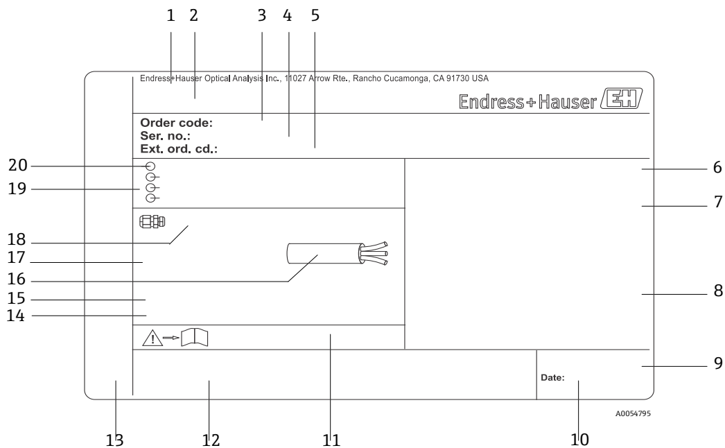
Рисунок 1. Заводская табличка анализатора JT33 типа VA с разрешениями и предупреждениями
