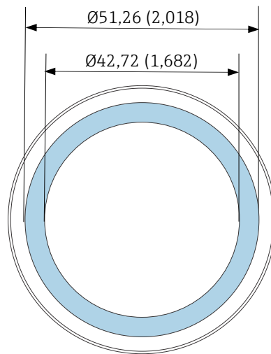
Рисунок 25. Требуемая чистая область на зеркале. Размеры: мм (дюймы)
