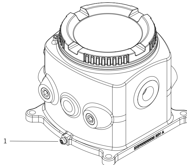
Рисунок 19. Точка заземления корпуса MAC (1)
