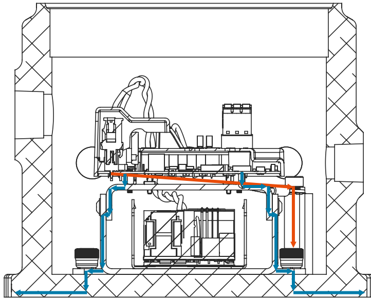
Рисунок 18. Контур заземления PCBA MAC
