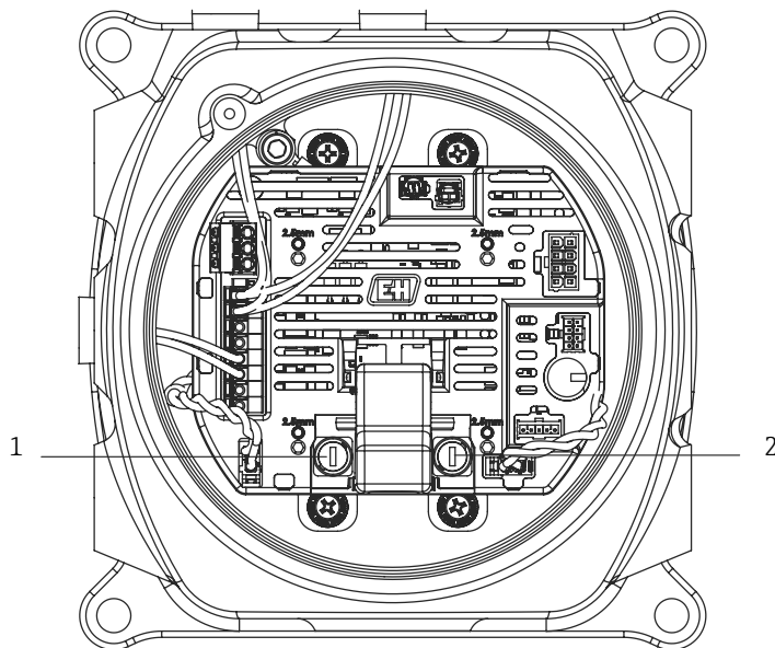
Рисунок 27. Расположение предохранителей на печатной плате MAC
