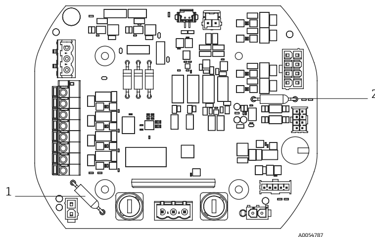
Рисунок 28. Расположение тепловых предохранителей
