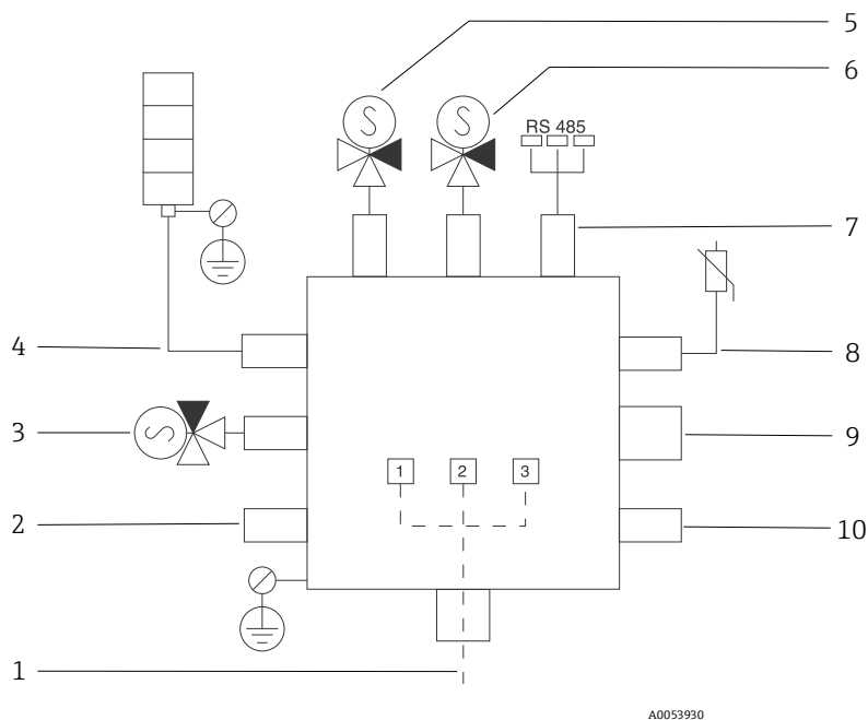
Рисунок 22. Места расположения приборов / датчиков в корпусе MAC
