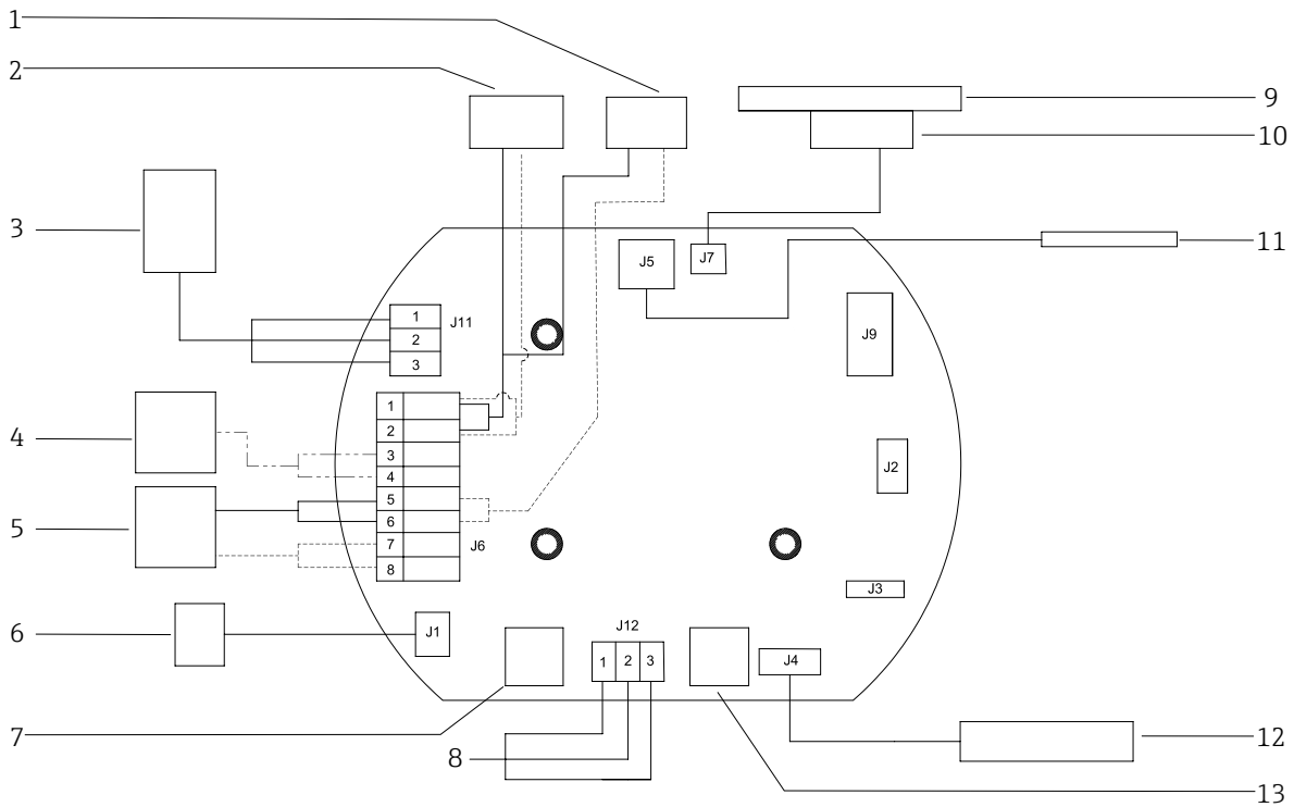
Рисунок 23. Схема подключения печатной платы MAC (напряжение от 120 до 240 В перем. тока)
