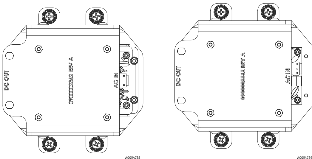
Рисунок 29. Монтажное положение блока питания: TDK (слева) и Sincon (справа)
