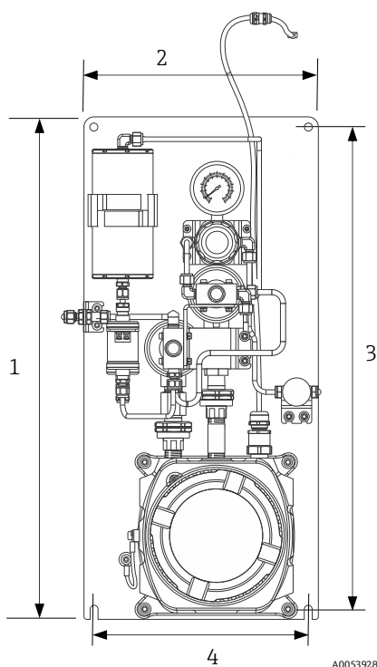
Рисунок 15. Дифференциальная панель для JT33
