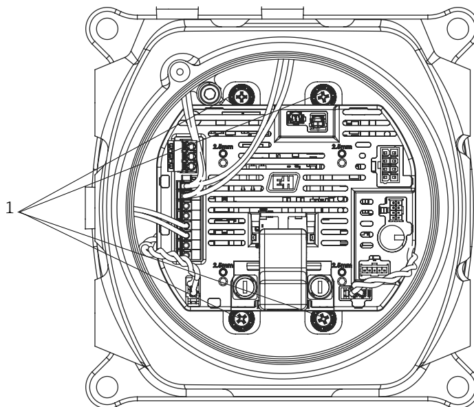
Рисунок 26. Расположение невыпадающих винтов (1) на панели
