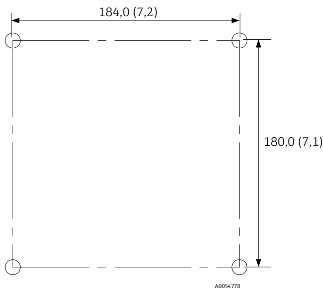
Рисунок 12. Схема отверстий для монтажа MAC в корпусе. Размеры: мм (дюймы)
