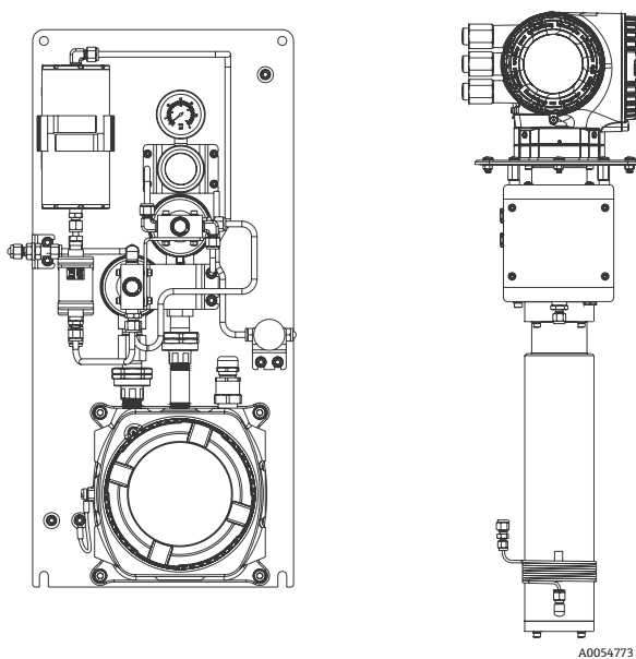
Рисунок 7. Газоанализатор JT33 типа TDLAS (без системы подготовки проб)
