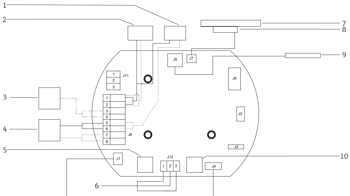
Рисунок 24. Схема подключения печатной платы MAC (напряжение 24 В пост. тока)
