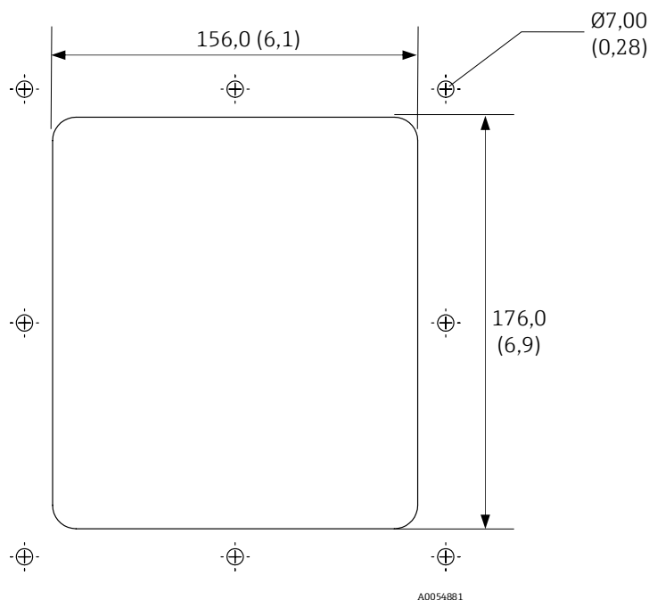
Рисунок 9. Вырез для монтажа в корпусе. Размеры: мм (дюймы)
