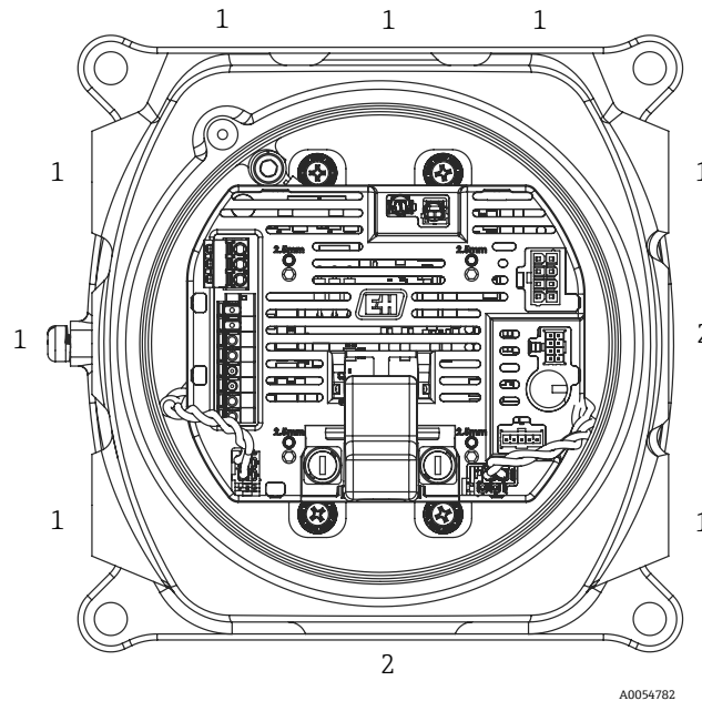
Рисунок 21. Размеры резьбы точек входа в корпус MAC
