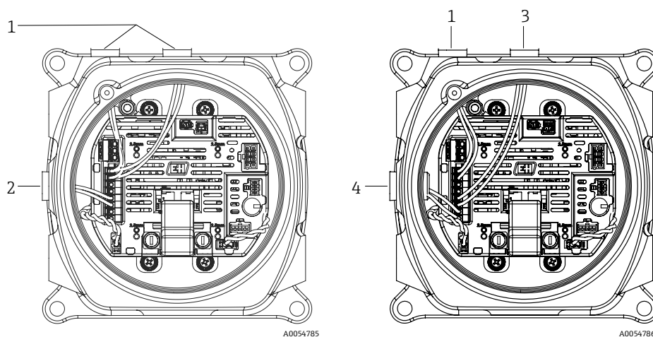
Рисунок 31. Провода электромагнита: электрическая (слева) и пневматическая (справа) конфигурация
