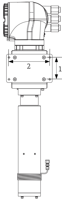
Рисунок 11. Размеры при панельном монтаже
