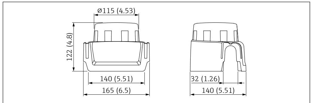
65 Dimensões da tampa de proteção contra tempo, plástico, XW111. Unidade de medida mm (in)
