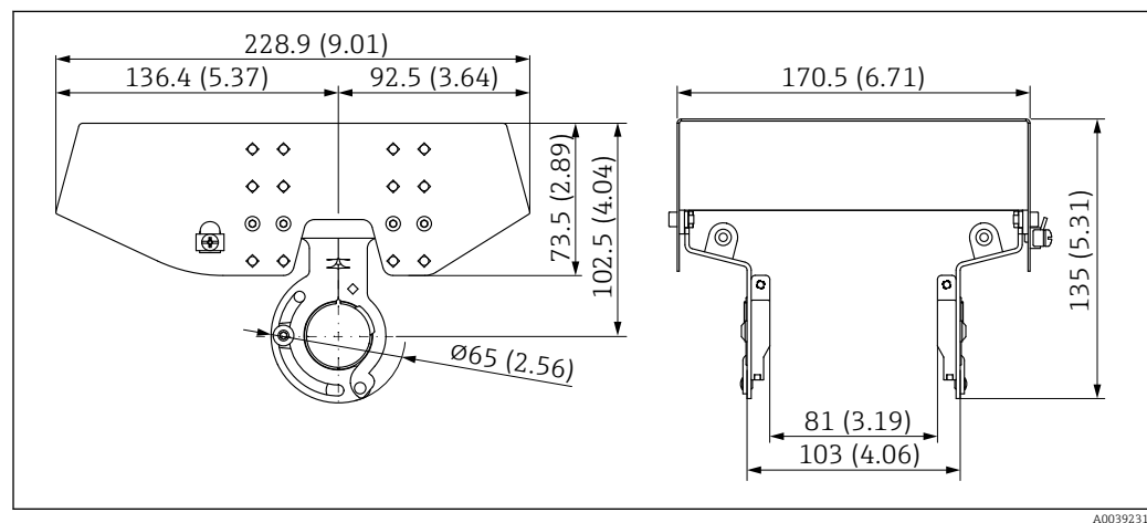
64 Dimensões da tampa de proteção contra tempo: 316 L, XW112. Unidade de medida mm (in)
