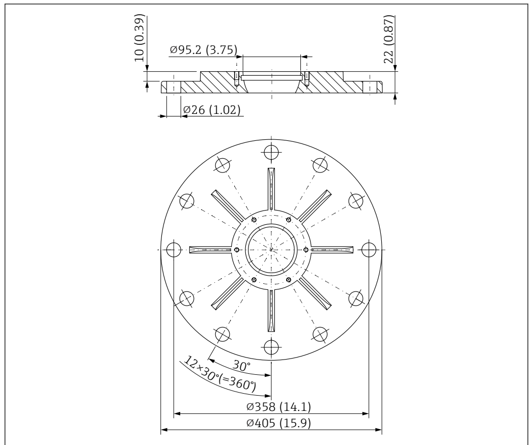
59 Medidas de la brida UNI 10" / DN 250 / 250 A para antenas con unidad de alineación. Unidad de medida mm (in)
