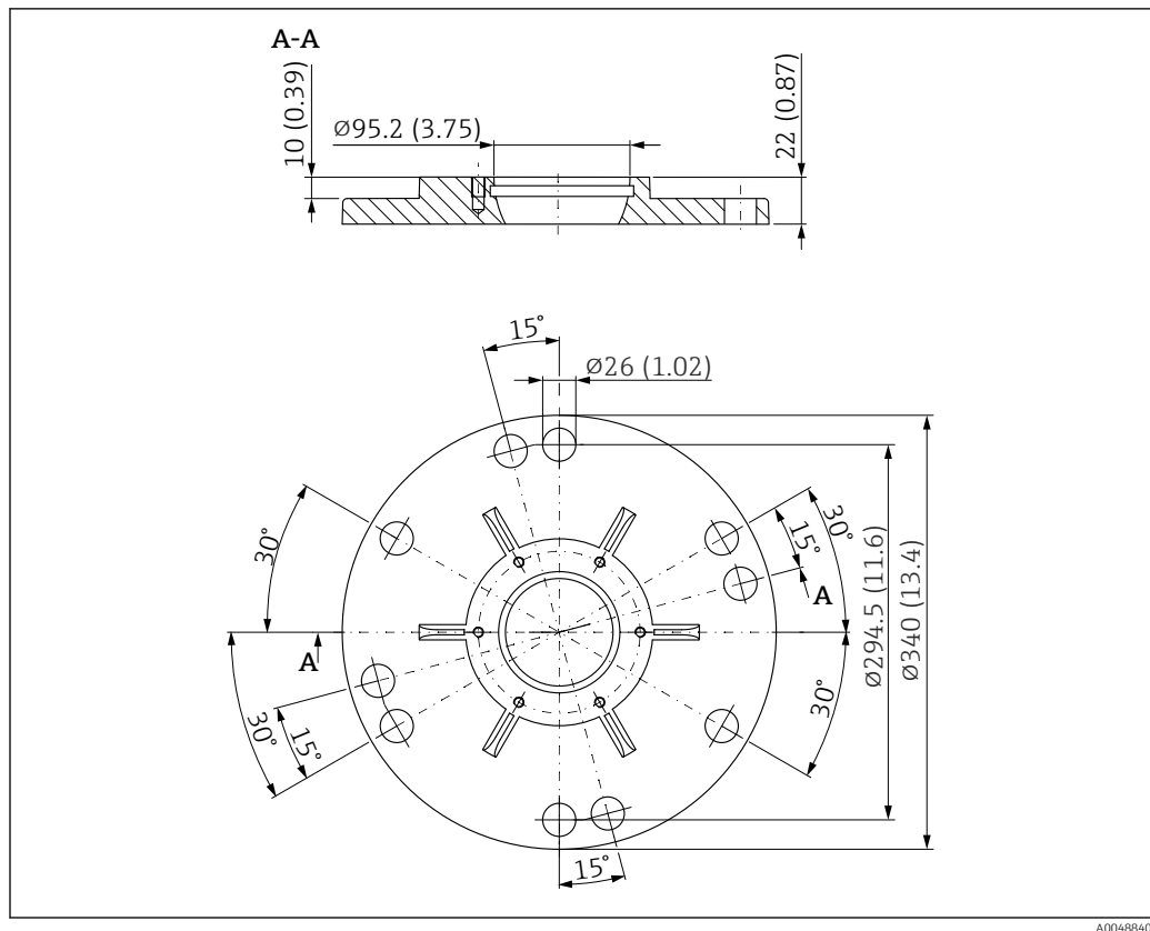
58 Medidas de la brida UNI 8" / DN 200 / 200 A para antenas con unidad de alineación. Unidad de medida mm (in)
