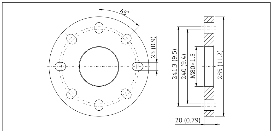
50 UNI brida 6" / DN 150 / 150 A para antena de goteo, PTFE, 50 mm (2 in) con conexión de aire de purga. Unidad de medida mm (in)
