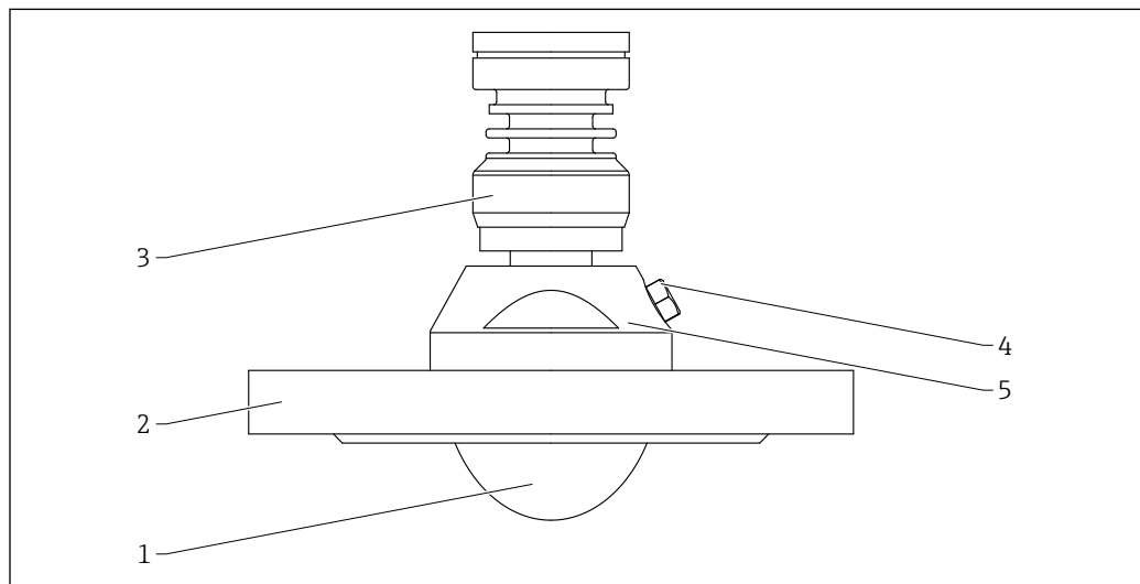
63 Material; antena, soporte para montaje enrasado, 80 mm (3 in), con brida y conexión de aire de purga. Unidad de medida mm (in)
