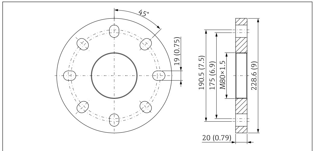
49 Brida UNI 4" / DN 100 / 100 A para antena de goteo, PTFE, 50 mm (2 in) con conexión de aire de purga. Unidad de medida mm (in)
