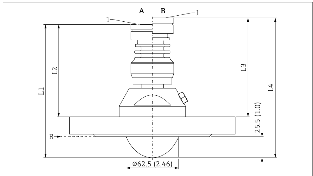
51 Medidas de la antena de montaje enrasado, PTFE, 80 mm (3 in), con brida estándar y conexión de aire de purga. Unidad de medida mm (in)
