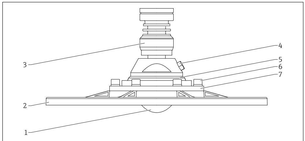
65 Material, antena, soporte para montaje enrasado, 80 mm (3 in), con brida UNI, unidad de alineación y conexión de aire de purga
