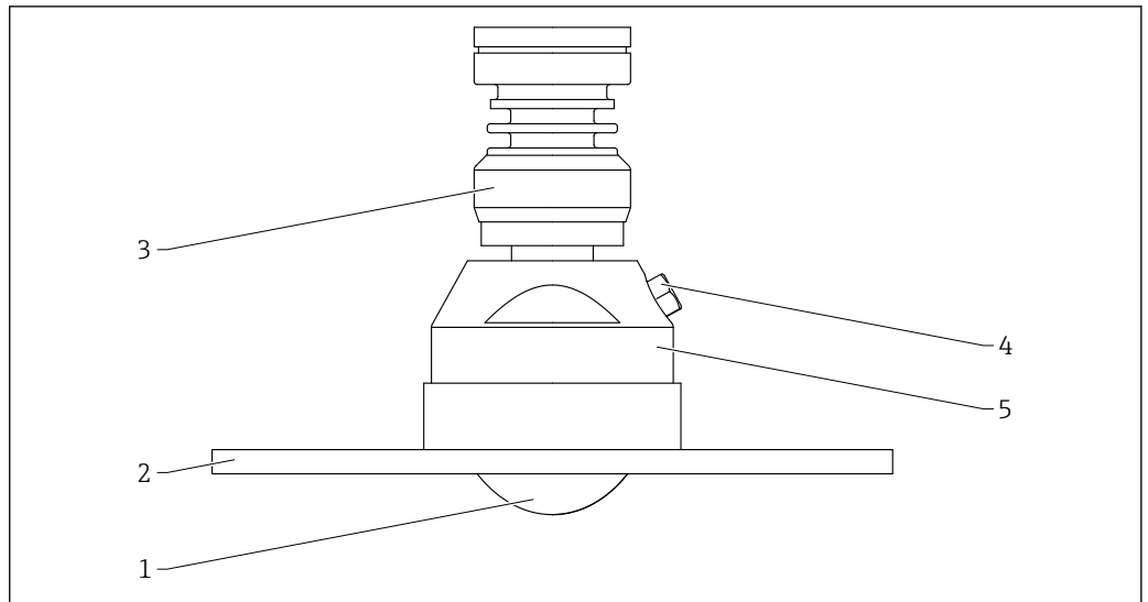
64 Material; antena, soporte para montaje enrasado, 80 mm (3 in), con brida UNI y conexión de aire de purga. Unidad de medida mm (in)
