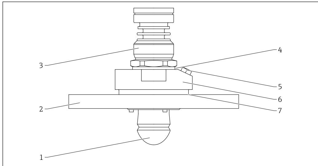
62 Material; antena de goteo, conexión de aire de purga . Unidad de medida mm (in)
