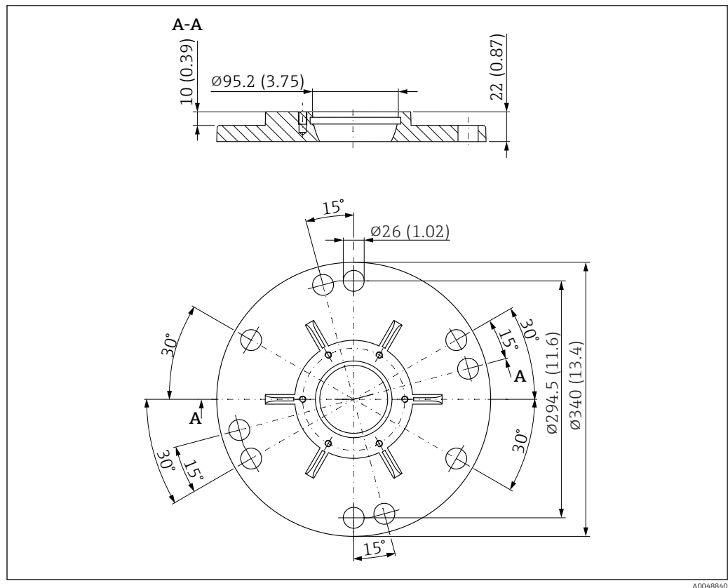
45 Medidas de la brida UNI 8" / DN 200 / 200 A para antenas con unidad de alineación. Unidad de medida mm (in)
