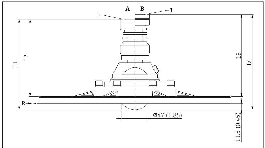
55 Medidas de la antena de montaje enrasado, 80 mm (3 in), con brida UNI, unidad de alineación y conexión de aire de purga. Unidad de medida mm (in)
