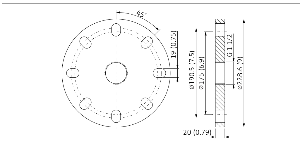
50 Dimensões da flange UNI 4"/DN100/100A. Unidade de medida mm (in)
