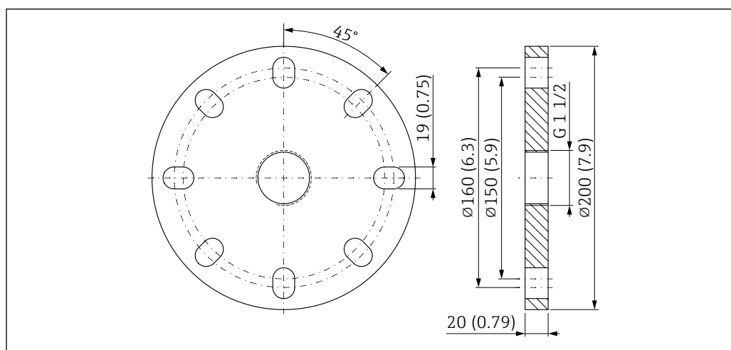
54 Dimensões da flange UNI 3"/DN80/80A. Unidade de medida mm (in)
