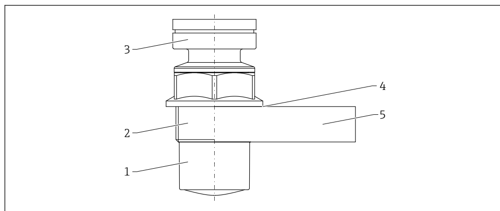
☑ 59 Material: antena encapsulada de PVDF, 40 mm (1.5 in)
