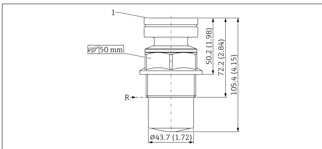
47 Dimensões da antena encapsulada, PVDF, 40 mm (1.5 in). Unidade de medida mm (in)
