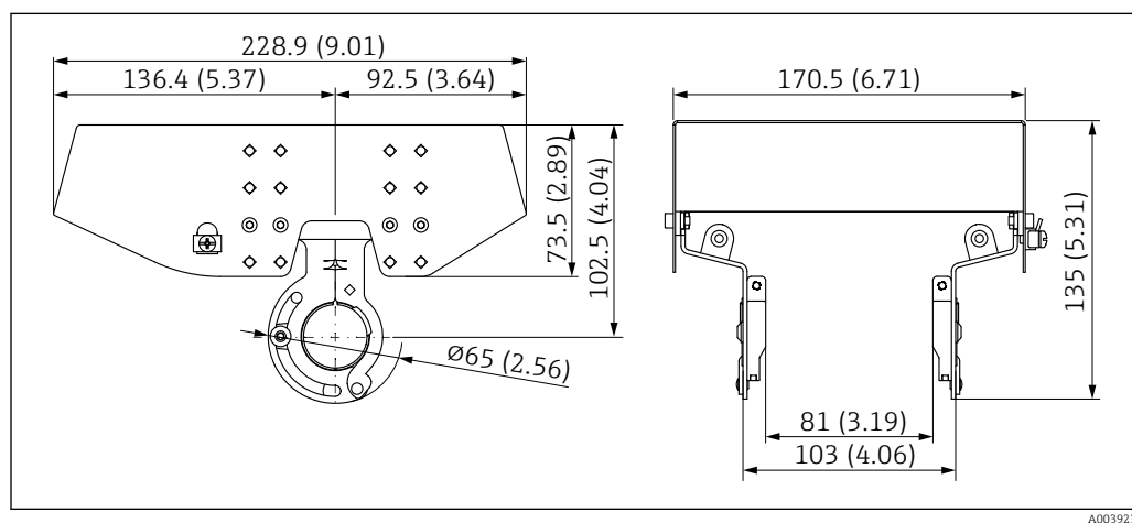
66 Dimensões da tampa de proteção contra tempo: 316 L, XW112. Unidade de medida mm (in)
