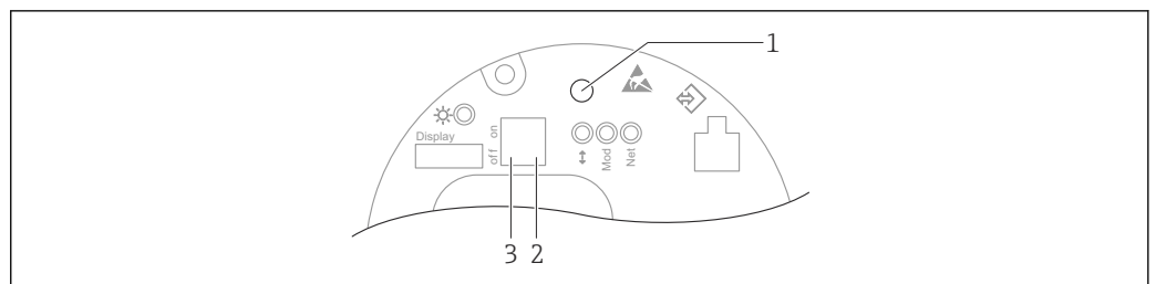
63 Teclas de operação e seletoras DIP na unidade eletrônica Ethernet-APL
