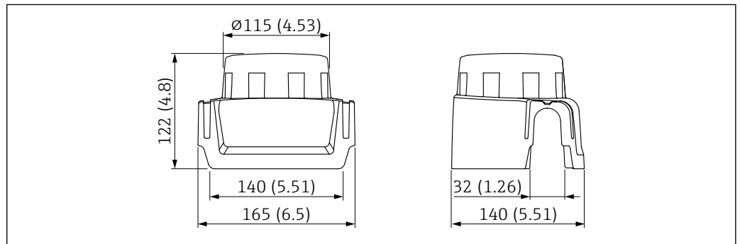
67 Dimensões da tampa de proteção contra tempo, plástico, XW111. Unidade de medida mm (in)
