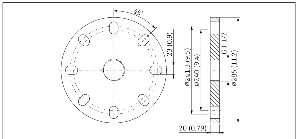
56 Dimensões da flange UNI 6"/DN150/150A. Unidade de medida mm (in)
