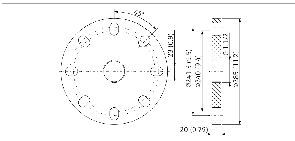
51 Dimensões da flange UNI 6"/DN150/150A. Unidade de medida mm (in)
