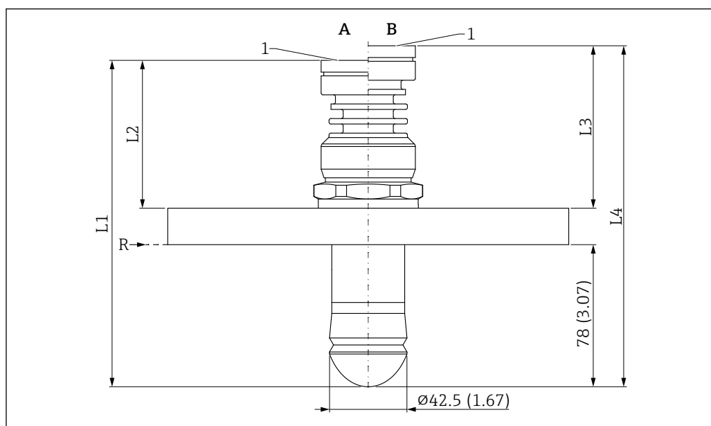
53 Dimensões da antena tipo drip-off 50 mm (2 in), conexão de processo: flange UNI. Unidade de medida mm (in)
