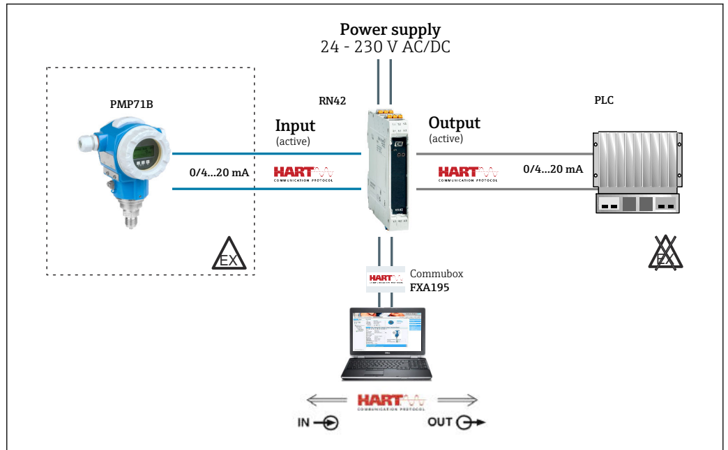
図 11 危険場所における RN42 アクティブバリアを使用した圧力測定
