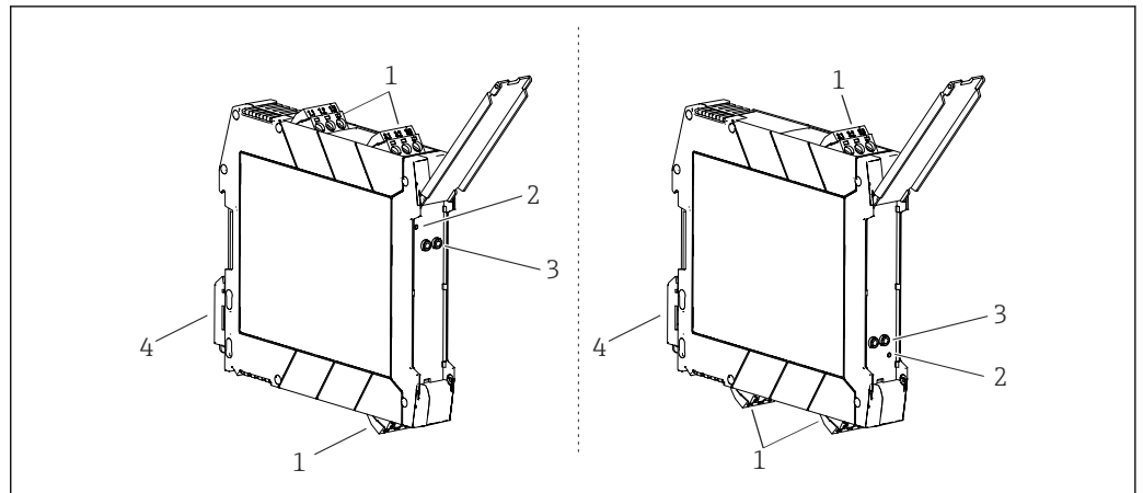
図9 表示部および操作部、左：電源上部；右：電源下部（オプション）
