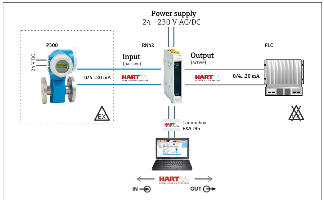
図 12 危険場所における RN42 アクティブバリアを使用した流量測定
