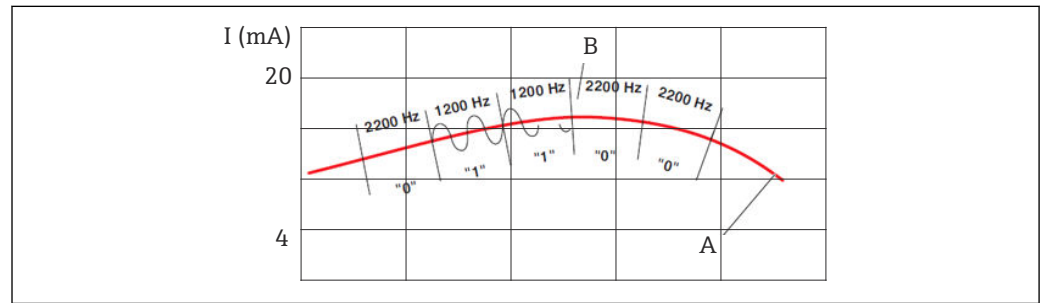
図 10 HART 変調信号
