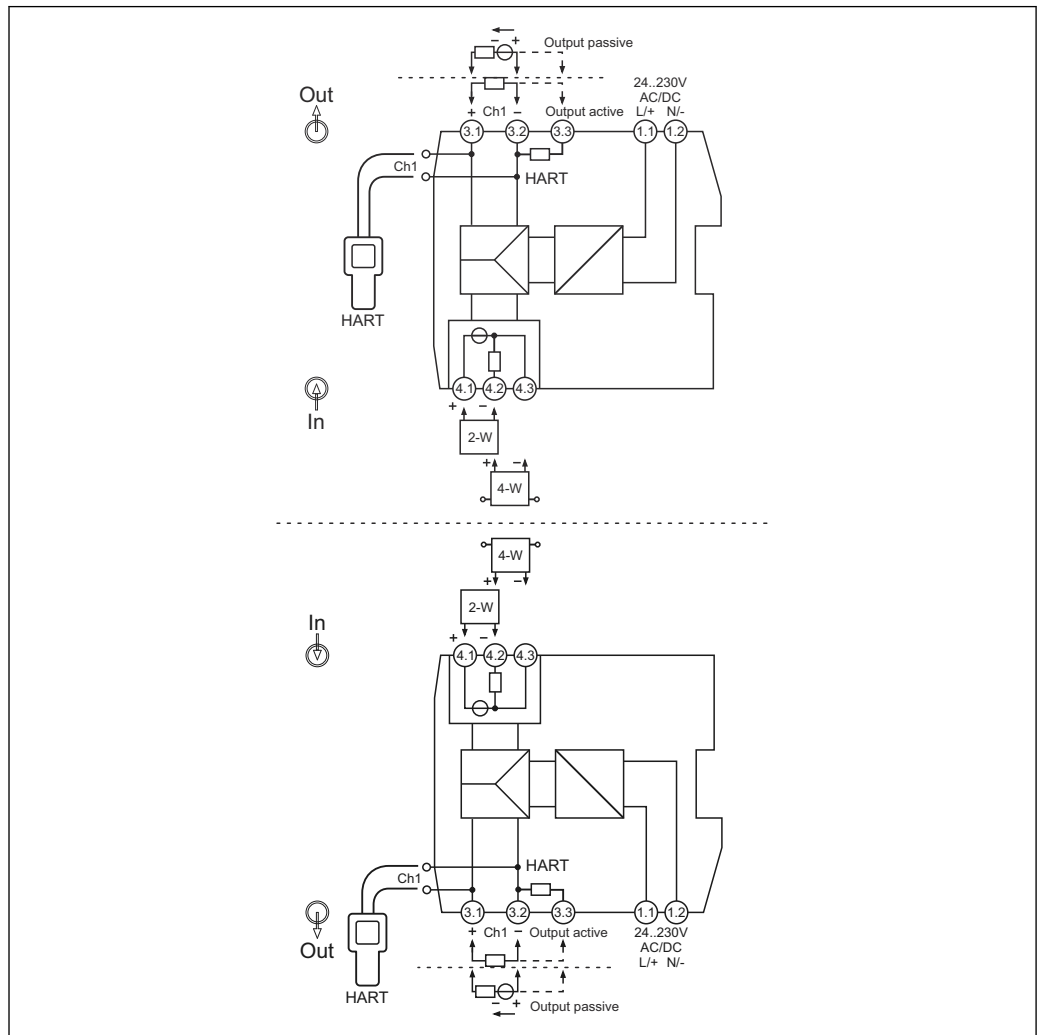
図 6 端子の割当て、上：電源上部；下：電源下部（オプション）
