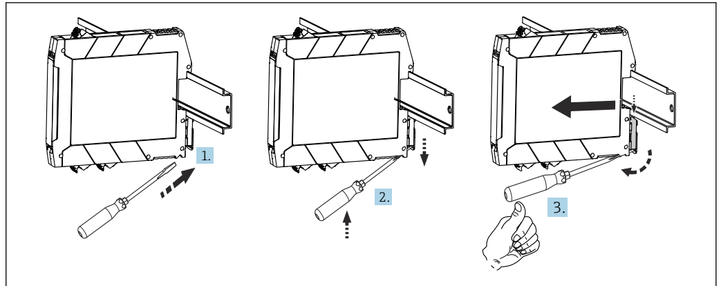
図 2 DIN レール機器の取外し
