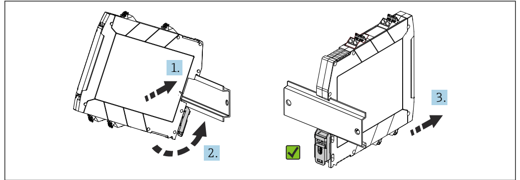
図 8 DIN レールへの取付け
