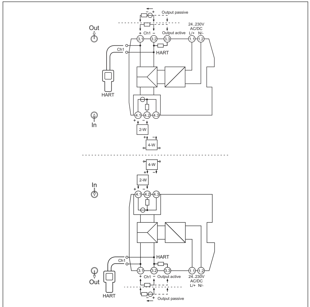
図4 端子の割当て、上：電源上部；下：電源下部（オプション）
