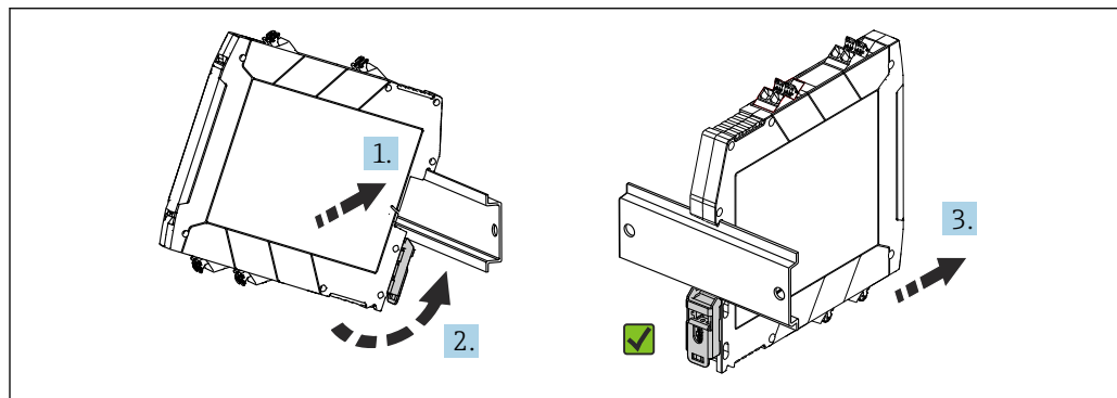
図 1 DIN レールへの取付け
