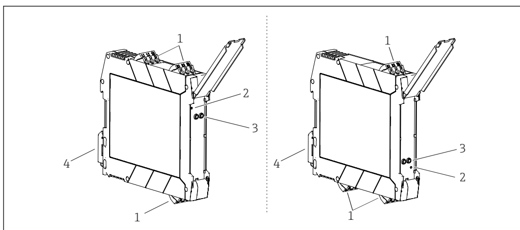
図 5 表示部および操作部、左：電源上部；右：電源下部（オプション）
