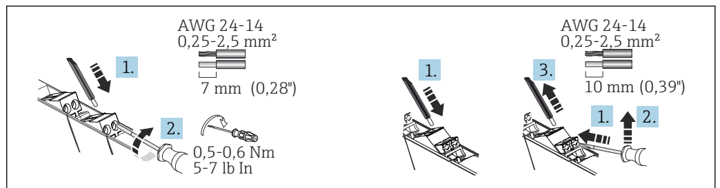
図 7 ネジ端子 (左) およびプッシュイン端子 (右) を使用した電気接続
