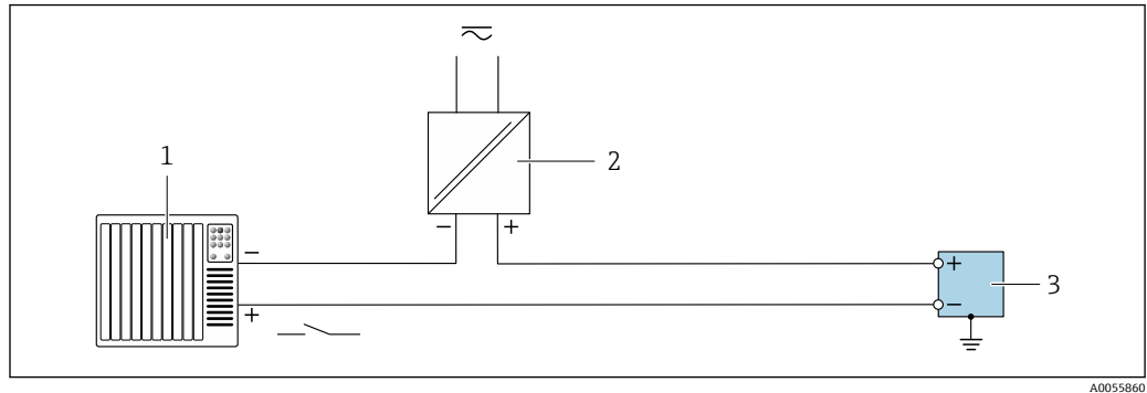
图 16 状态输入
