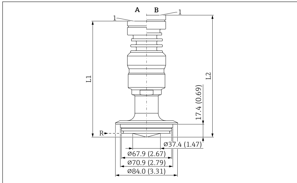
53 Medidas del soporte para montaje enrasado de la antena con revestimiento, PEEK, 40 mm (1,5 in) tubo Varivent N DN65-162. Unidad de medida mm (in)
