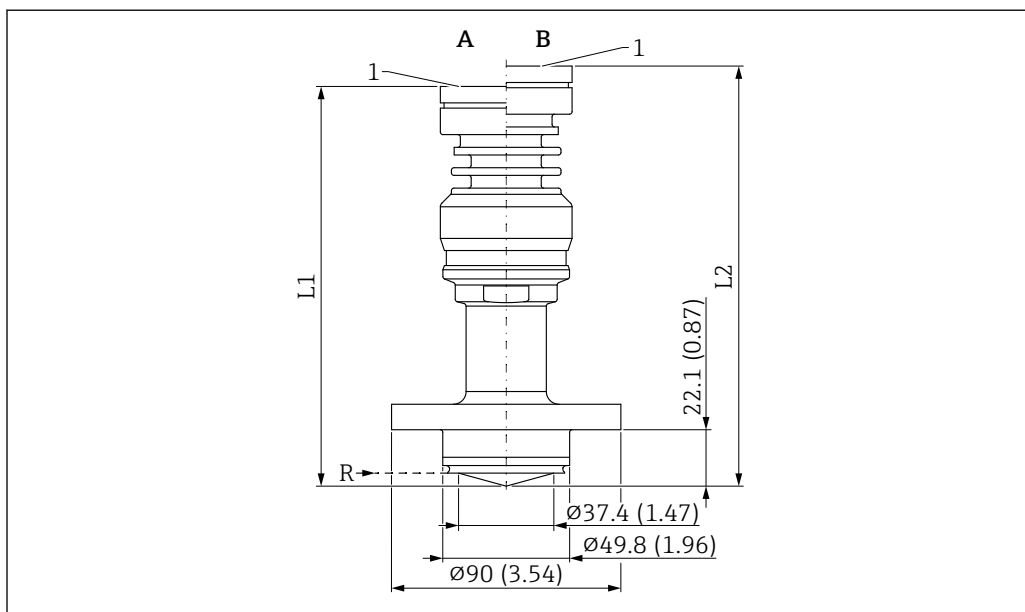
55 Medidas del soporte para montaje enrasado de la antena con revestimiento, PEEK, 40 mm (1,5 in), NEUMO BioControl D50. Unidad de medida mm (in)
