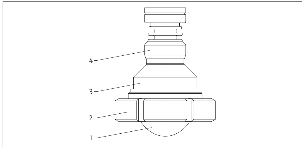
■ 58 Material; soporte para montaje enrasado de la antena con revestimiento, 80 mm (3 in), tuerca DIN11851. Unidad de medida mm (in)
