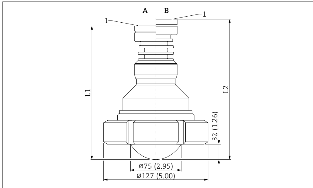
49 Medidas de la antena, montaje enrasado con revestimiento, PTFE, 80 mm (3 in), tuerca ranurada DIN 11851. Unidad de medida mm (in)
