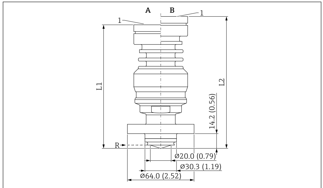
54 Medidas del soporte para montaje enrasado de la antena con revestimiento, PEEK, 20 mm (0,75 in), NEUMO BioControl D25. Unidad de medida mm (in)
