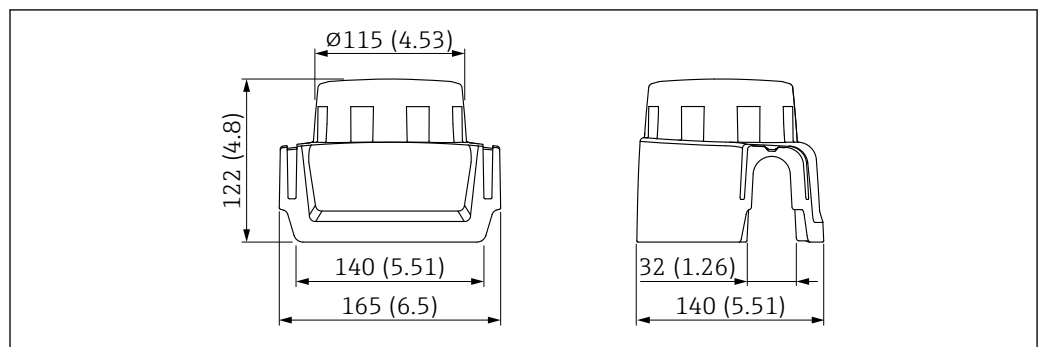
68 Medidas de la tapa de protección ambiental, plástico, XW111. Unidad de medida mm (in)
