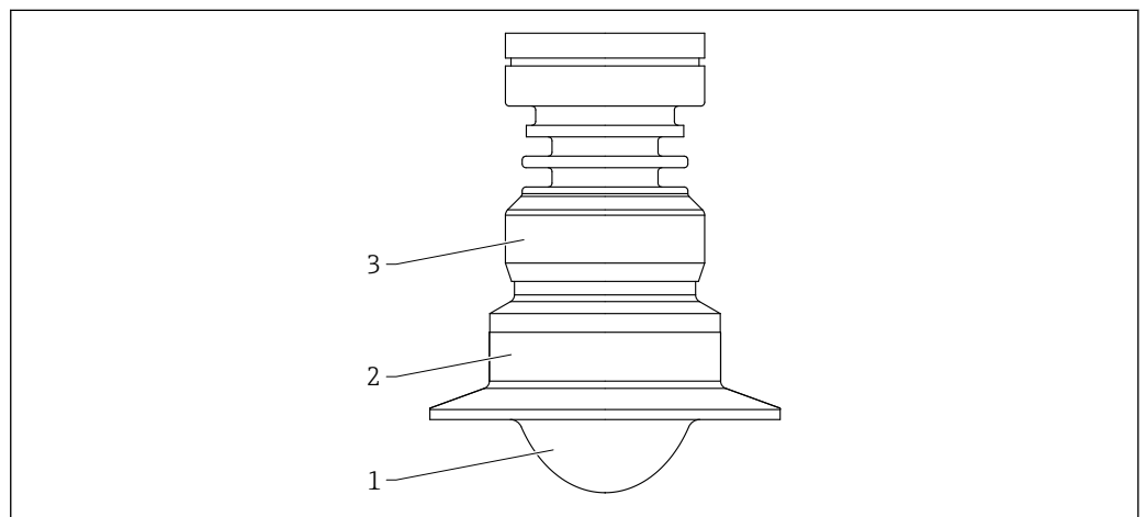
■ 59 Material; soporte para montaje enrasado de la antena con revestimiento, PTFE, 50 mm (2 in), con triclamp ISO2852. Unidad de medida mm (in)
