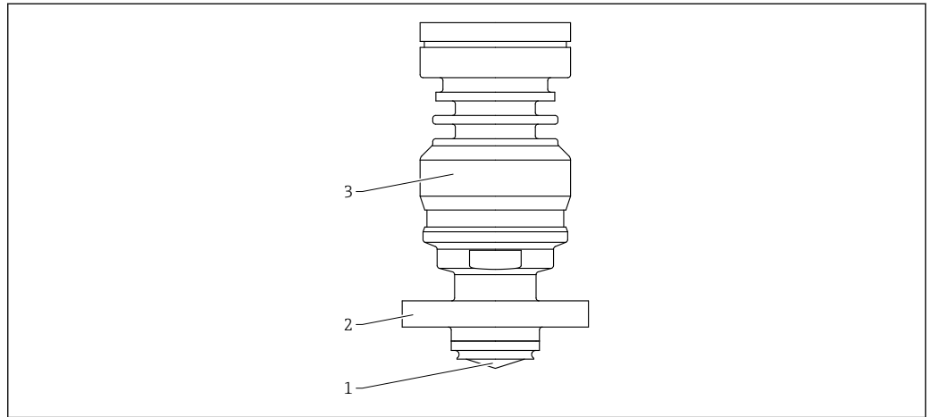
62 Material; soporte para montaje enrasado de la antena con revestimiento, PEEK, 20 mm (0,75 in), NEUMO BioControl D25
