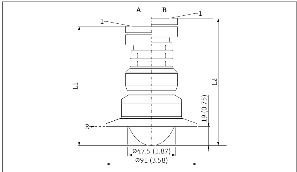
51 Medidas de la antena, montaje enrasado con revestimiento, PTFE, 50 mm (2 in), con Tri-Clamp DN 70-76.1 (3") ISO 2852. Unidad de medida mm (in)
