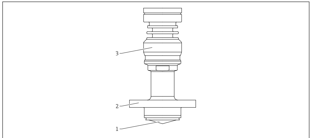
63 Material; soporte para montaje enrasado de la antena con revestimiento, PEEK, 40 mm (1,5 in), NEUMO BioControl D50
