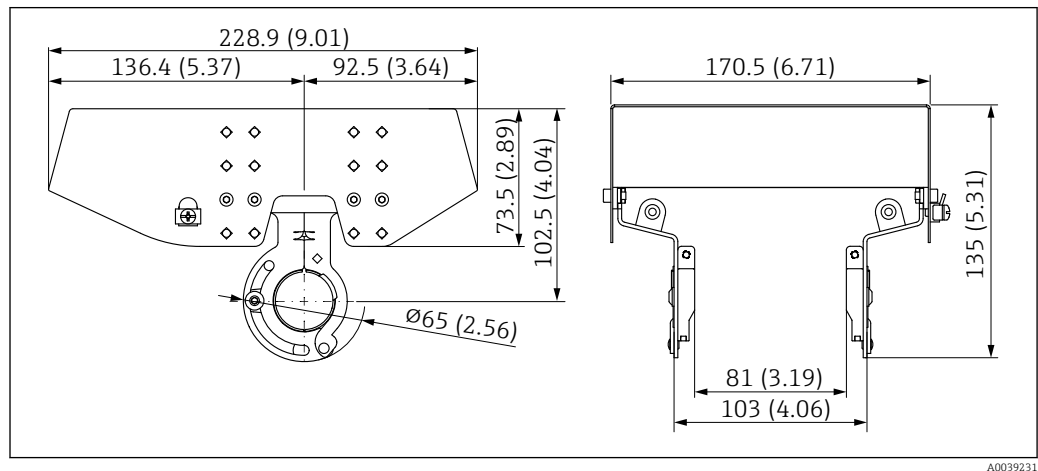
67 Medidas de la tapa de protección ambiental, 316 L, XW112. Unidad de medida mm (in)
