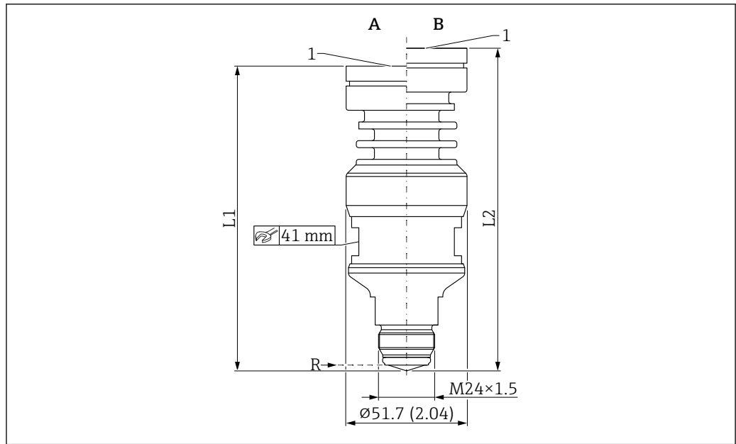
47 Medidas de la antena integrada, PEEK, 20 mm (0,75 in) con rosca de conexión a proceso M24. Unidad de medida mm (in)
